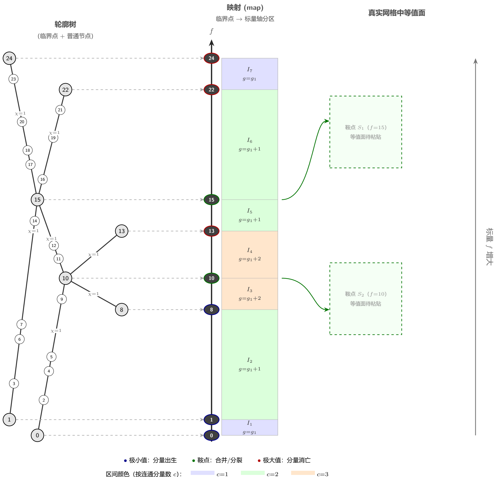
图 1 增广轮廓树 \rightarrow 临界值分区映射
