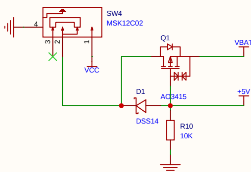
锂电池与外部供电自动切换
