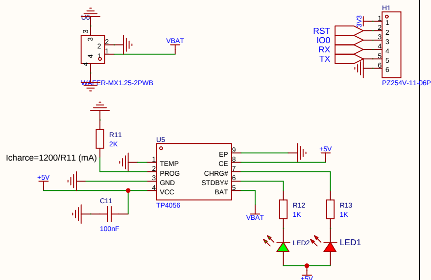
锂电池充电
