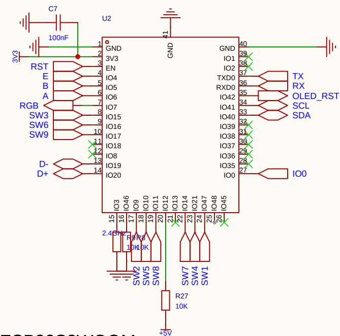
ESP32S3WOOM
