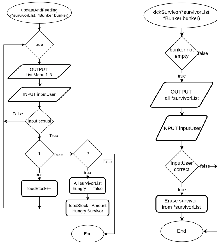
Gambar 1.5. Flowchart Prosedur Cari Makan dan Beri Makan
