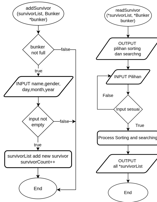
Gambar 1.4 Flowchart Prosedur Menambah dan Melihat Survivor
