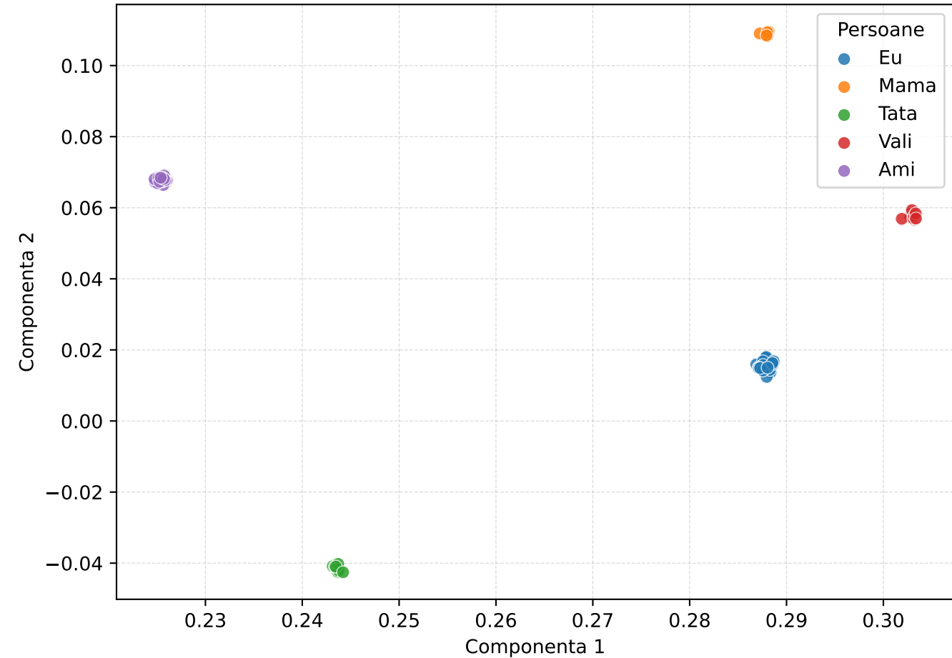
LDA - Supervizat (5 persoane)
