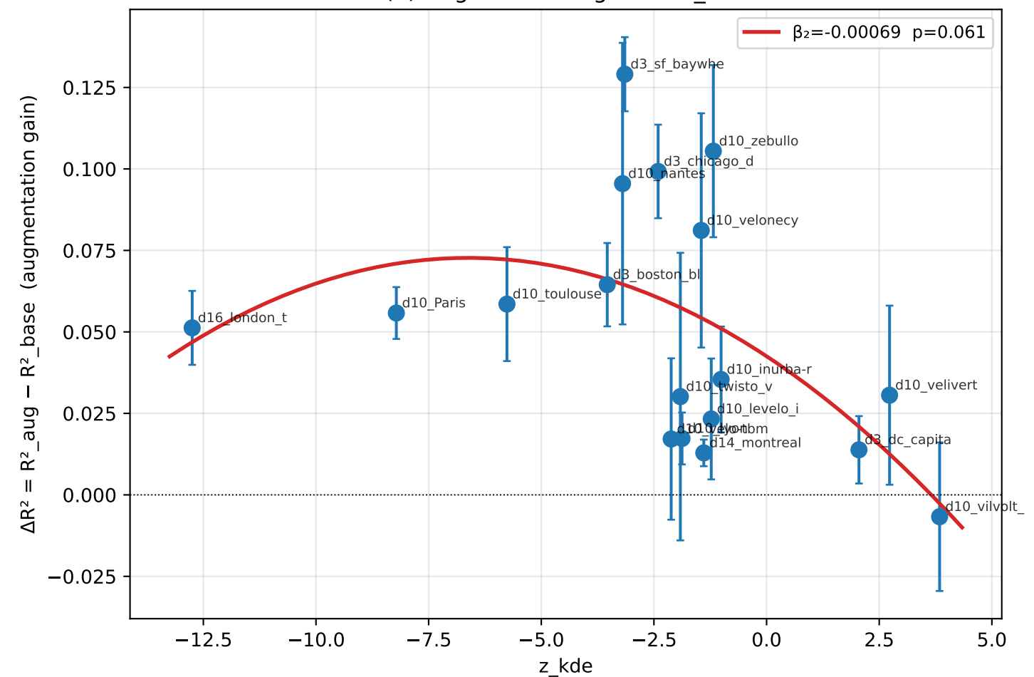
(d) Are z_{\text{kde}} and Dirichlet independent?
