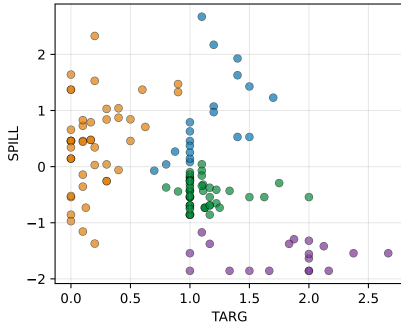
Hierarchical (Ward) silhouette=0.453
