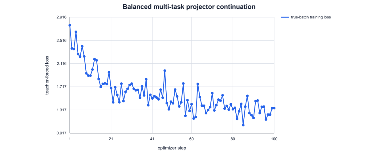
Figure 9: 一轮六任务均衡 projector continuation 的 true-batch loss。每步六项任务配额固定，不把任务采样漂移混入能力轨迹。
