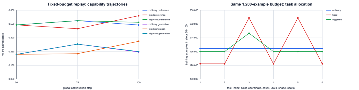
Figure 23: 左: ordinary、fixed 与 triggered 的 macro preference/generation 轨迹; 右: 同一 1,200-example 总预算内的任务分配。
