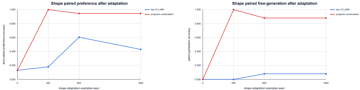
Figure 5: 左: strict paired preference; 右: 自由生成 paired accuracy. projector 续训在 400 个 shape 样本处已达到完整配对恢复, LoRA 只恢复一部分。
