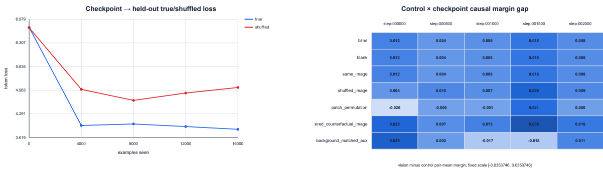
Figure 2: 左：heldout 真图与错配图 loss 轨迹；右：synthetic 控制条件相对 vision 的 correct-margin gap。
