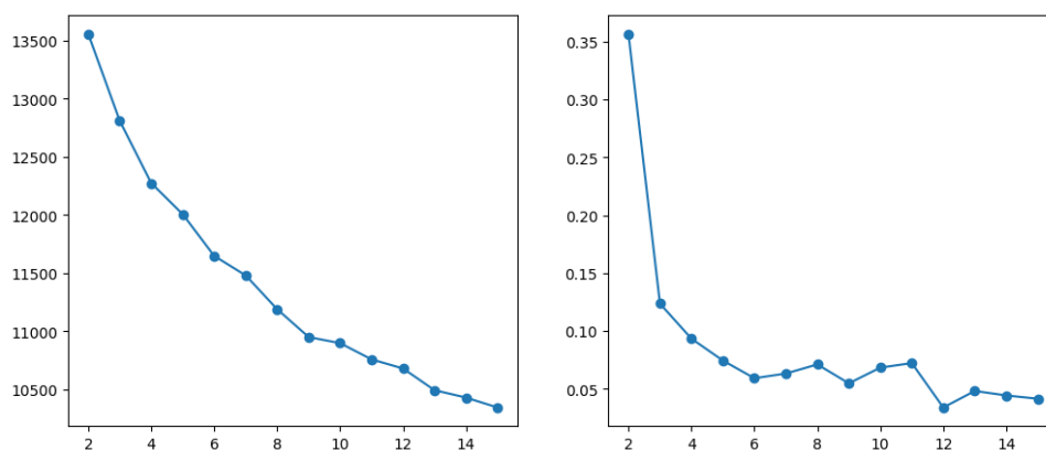
FIGURE 9.5 – Courbes WCSS et silhouette pour la sélection de k (Victor)
