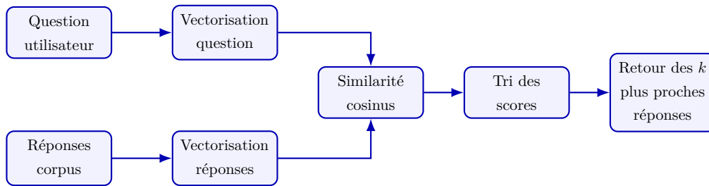
FIGURE 12.3 – Schéma de la méthode de similarité question-réponse (version 1 : recherche sur l'ensemble du corpus).
