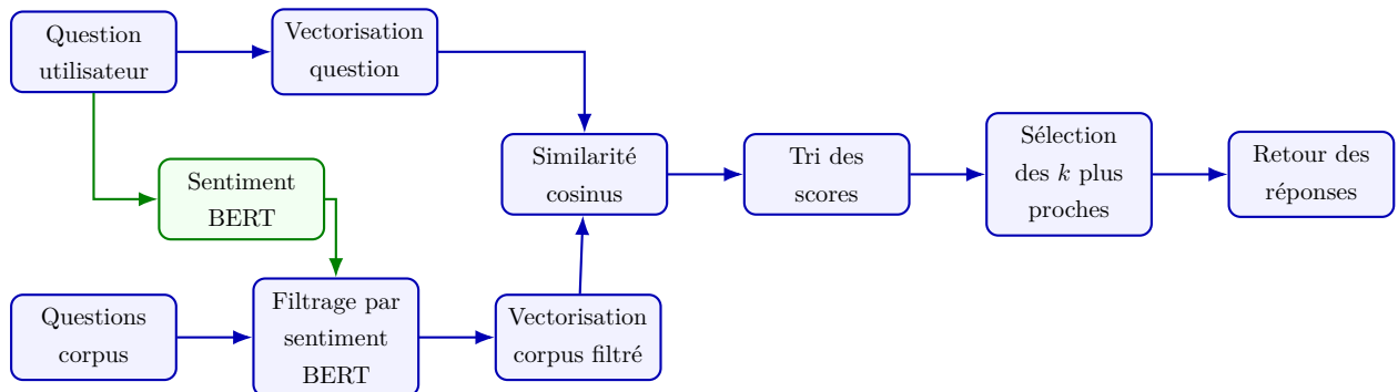
FIGURE 12.2 – Schéma de la méthode de similarité question-question (version 2 : filtrage par sentiment BERT).
