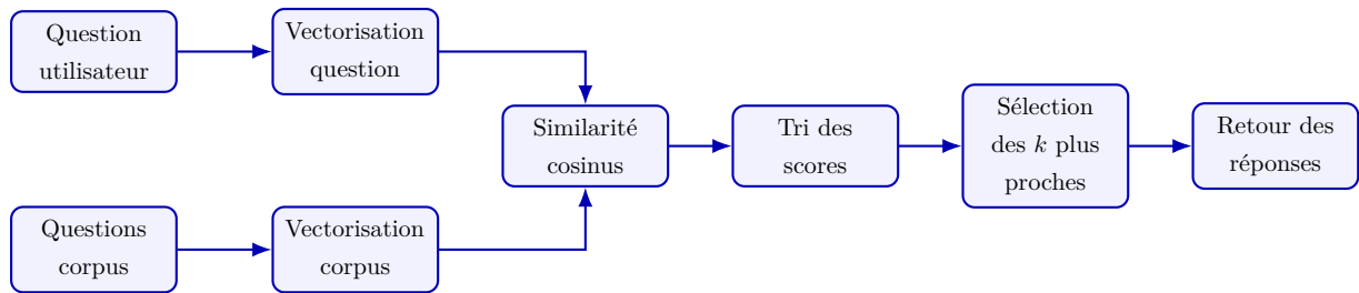
FIGURE 12.1 – Schéma de la méthode de similarité question-question (version 1 : recherche sur l'ensemble du corpus).
