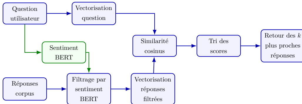
FIGURE 12.4 – Schéma de la méthode de similarité question-réponse (version 2 : filtrage par sentiment BERT).
