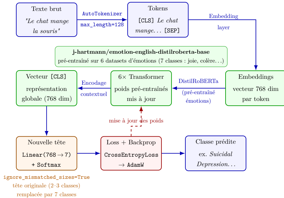
FIGURE 10.5 – Schéma du pipeline du Modèle C : DistilRoBERTa pré-entraîné sur des émotions (j-hartmann/emotion-english-distilroberta-base), tête de classification remplacée (ignore_mismatched_sizes=True) et fine-tuné sur 7 classes de santé mentale.
