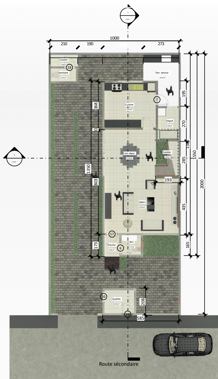
VUE EN PLAN RDC
