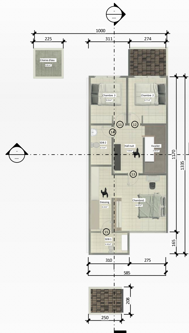
VUE EN PLAN ETAGE
