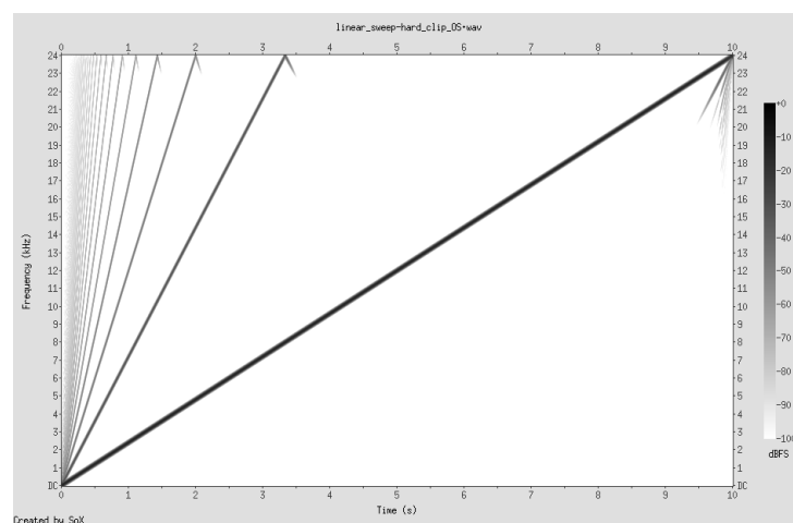
FIGURE 1.3 – Balayage sinusoidal linéaire écrêté de 3dBFS avec suréchantillonnage de facteur 8.
