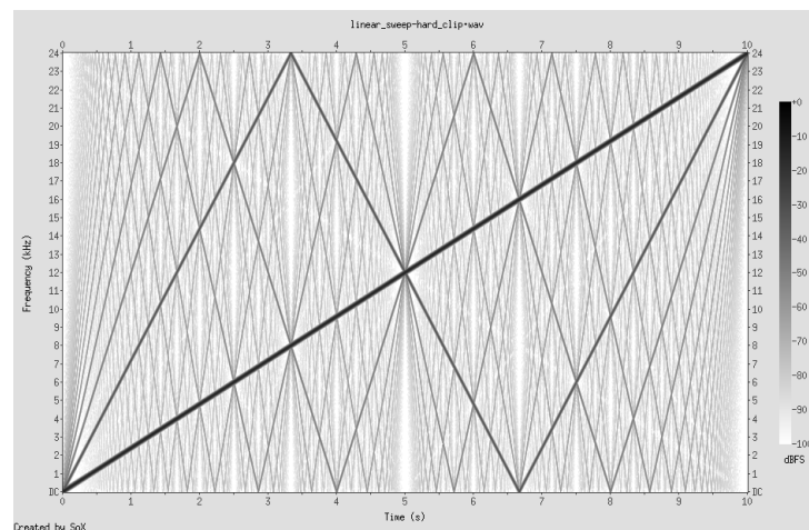
FIGURE 1.2 – Balayage sinusoidal linéaire écrêté de 3dBFS sans suréchantillonnage.
