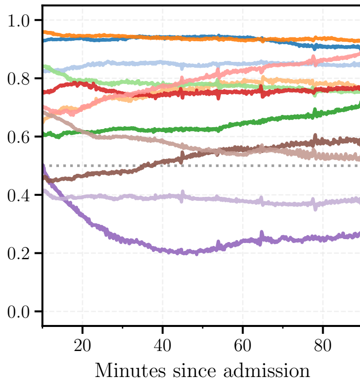
Vanilla VAE
