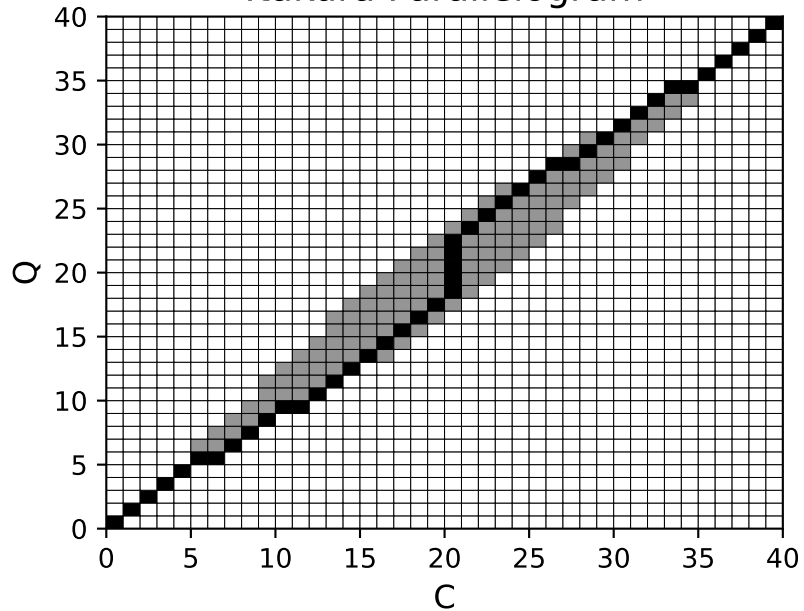
Itakura Parallelogram
