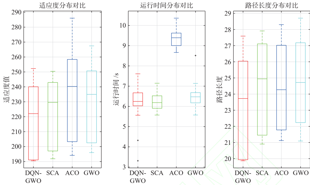
图 9 任务 2 的实验结果数据箱线图
