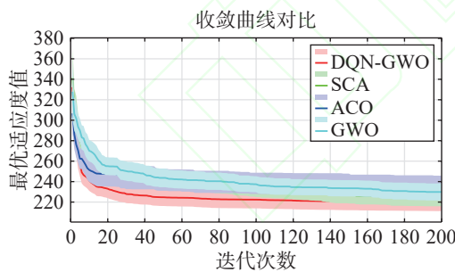
图 8 任务 2 的多算法收敛曲线比较
