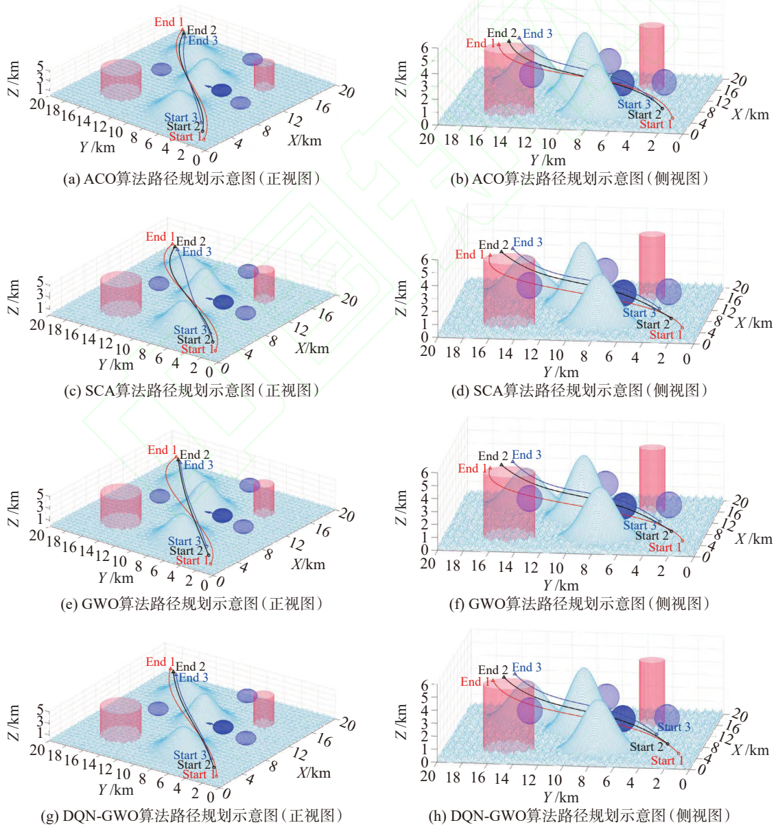
图 4 基础场景下的多起点、多目标点算法路径规划示意图
