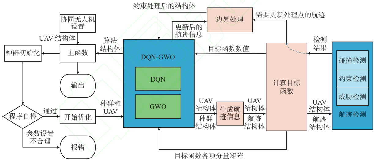
图 3 融合 DQN-GWO 算法流程图
