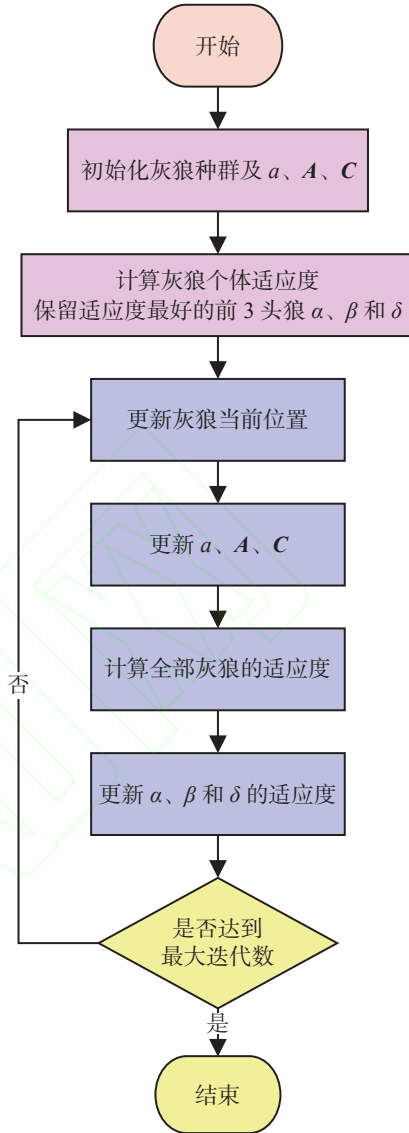
图 1 GWO 算法流程图
