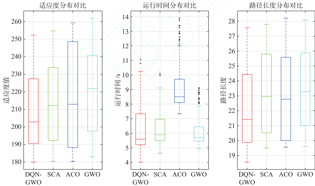
图6 任务1的实验结果数据箱线图
