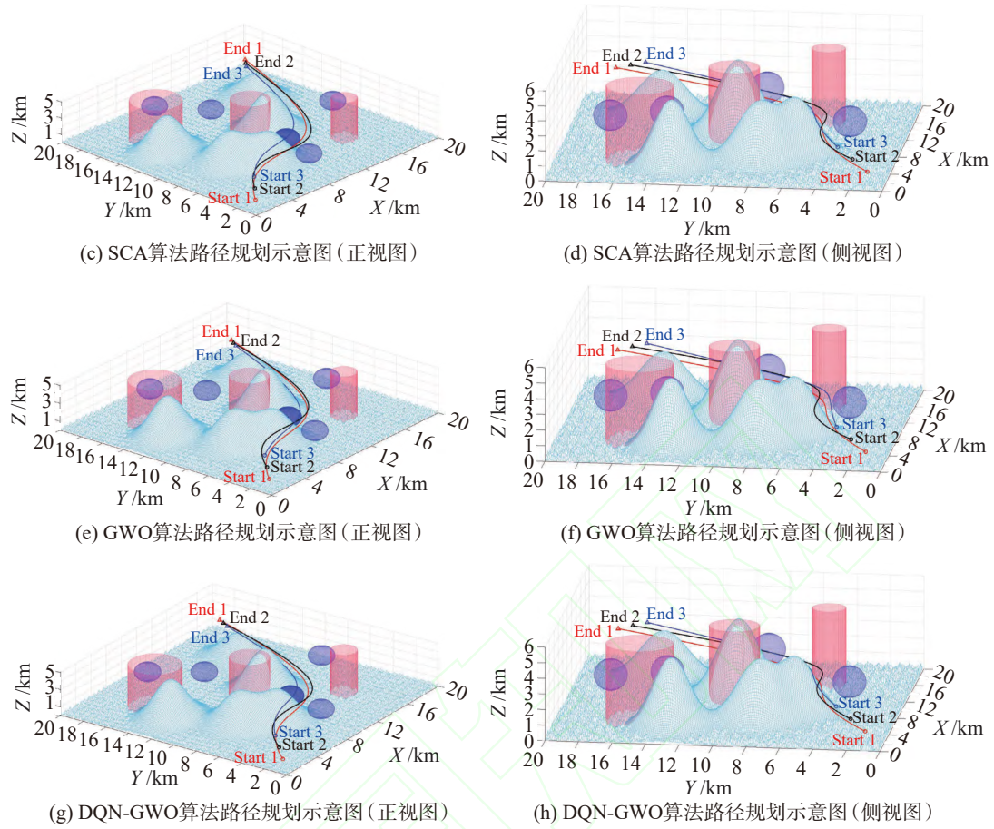
图7 复杂场景下的多起点多目标点算法路径规划示意图
