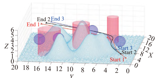
(b) ACO算法路径规划示意图(侧视图)
