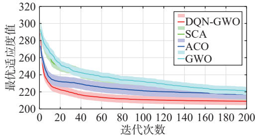
图5 任务1的多算法收敛曲线比较
