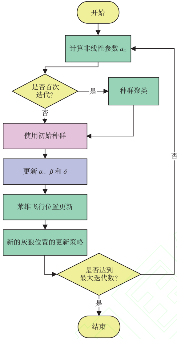
图2 改进 GWO 算法流程图
