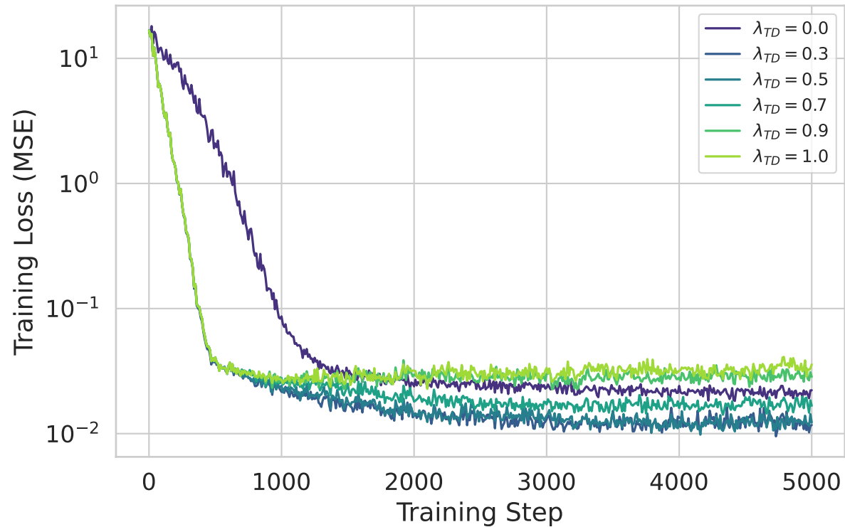
(d) Convergence at L = 8 (norm)
