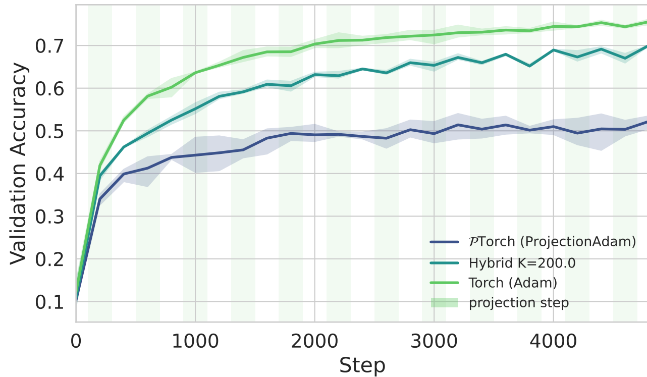
CIFAR10
