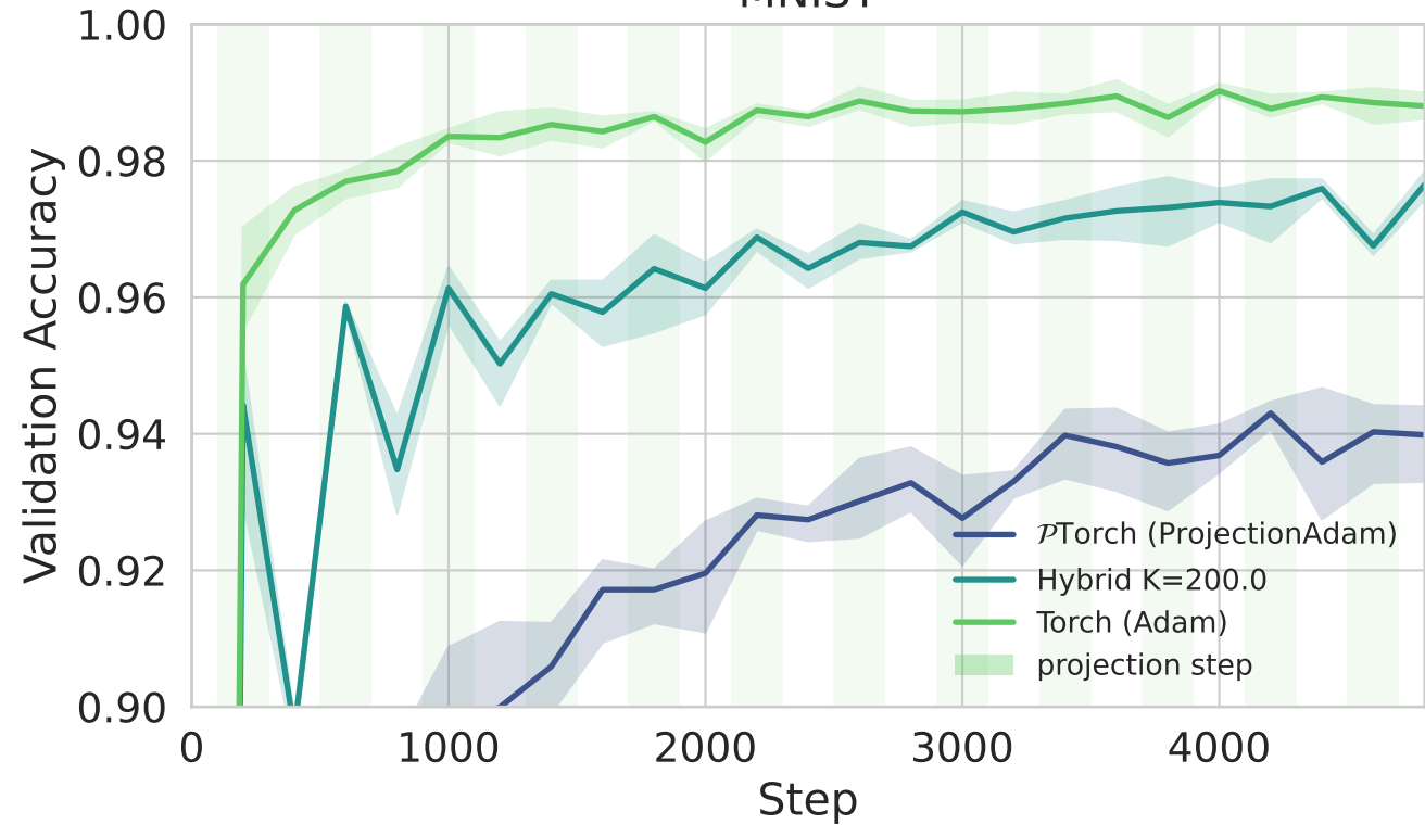
MNIST
