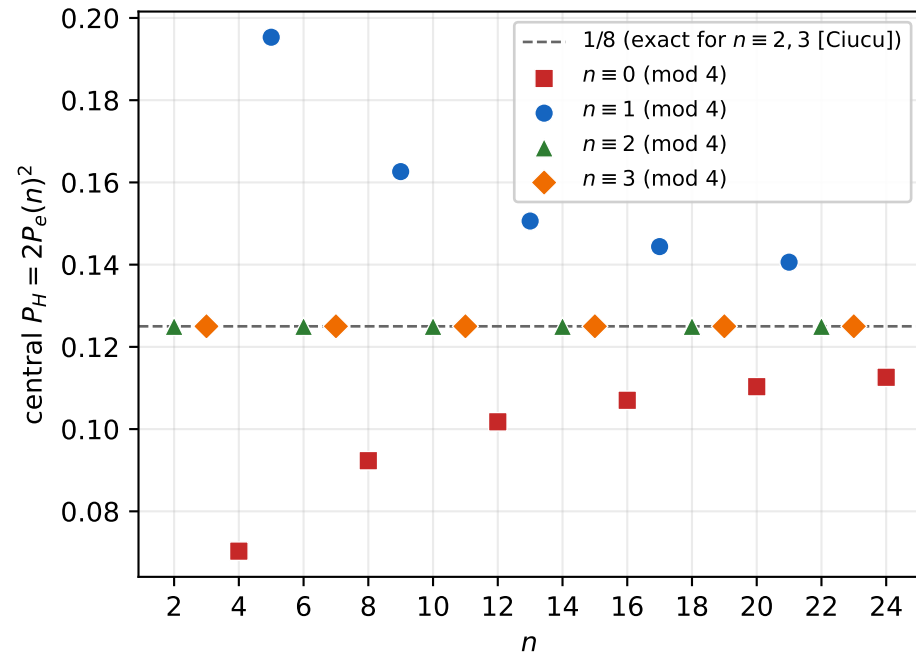
(d) Central 2 \times 2 square
