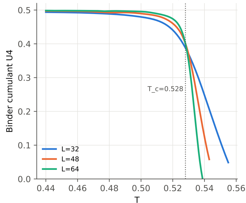
annealed bonds ( D2=1 , \mu=0 )
