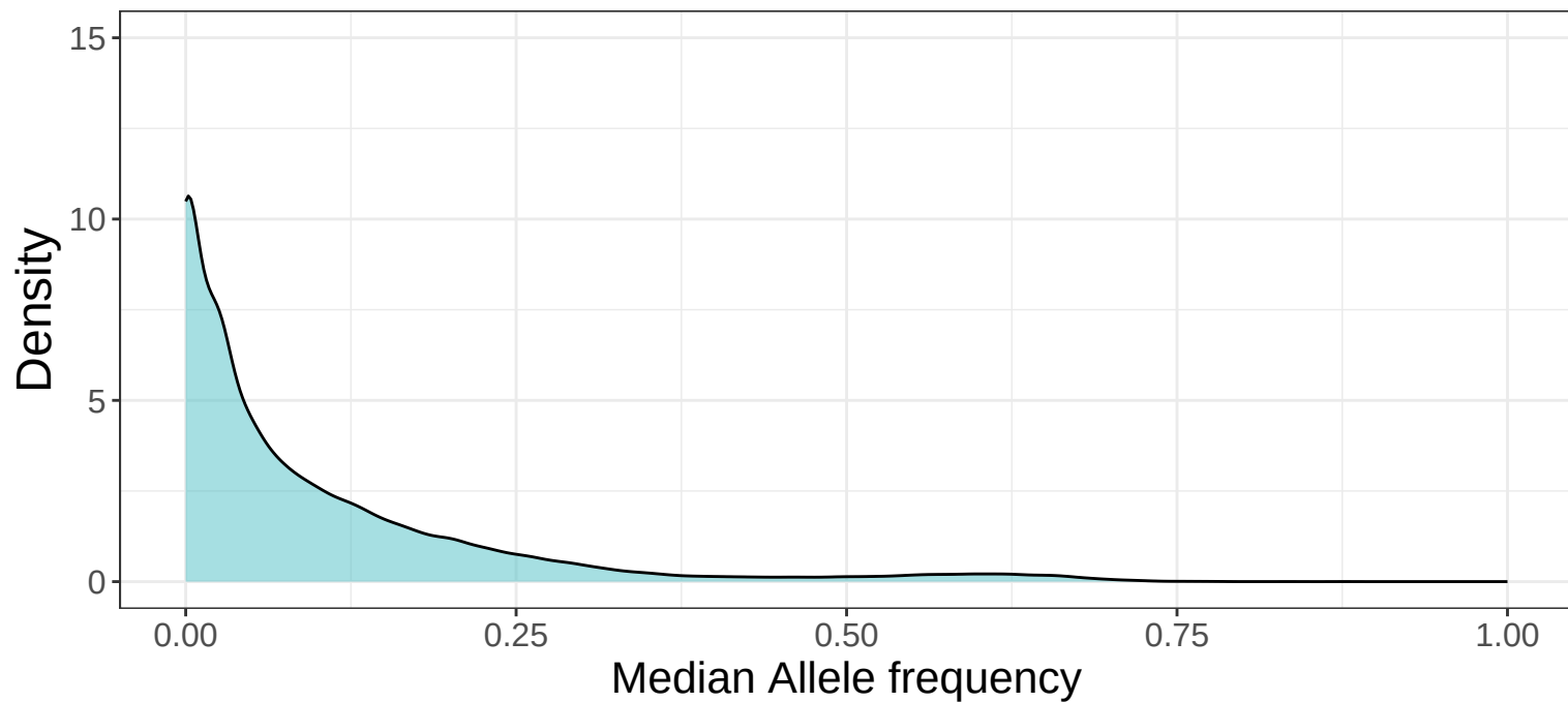
Fluc population
