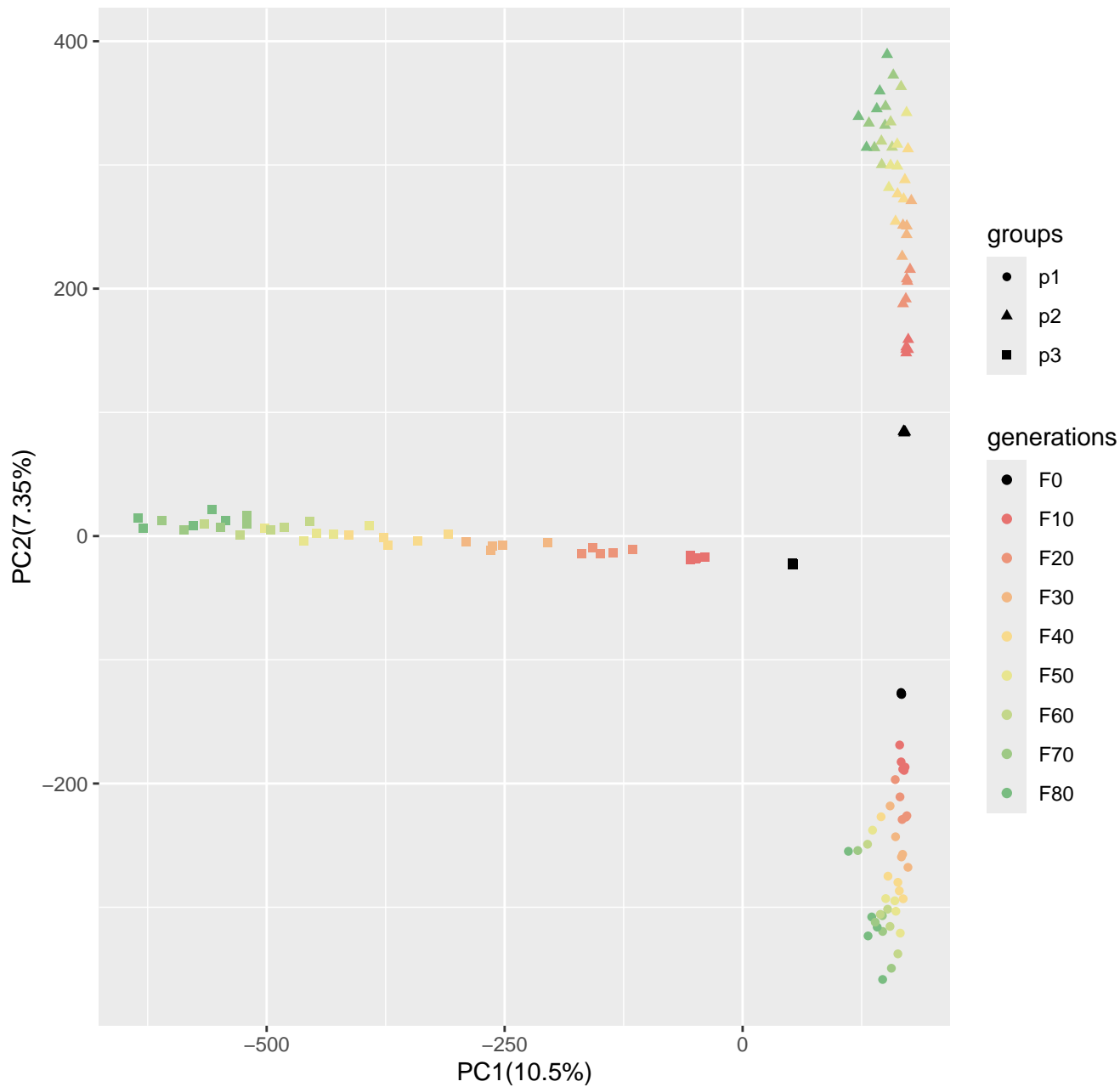
Run10_popsizel250_n400_5000loci_s50
