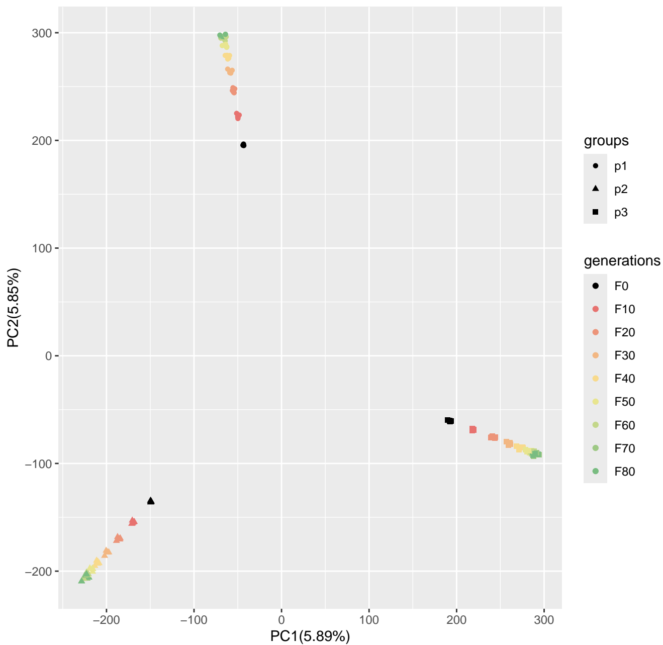
Run4_popsizel250_n400_10loci_s0
