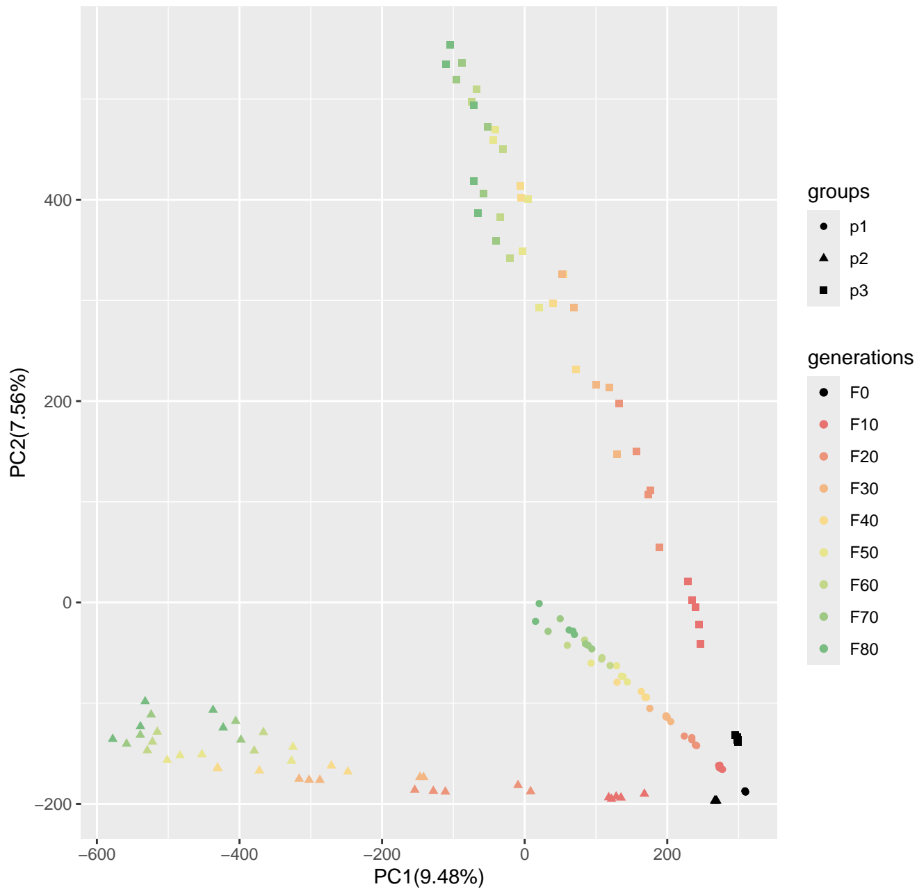
Run6_popsizel250_n800_100loci_s10
