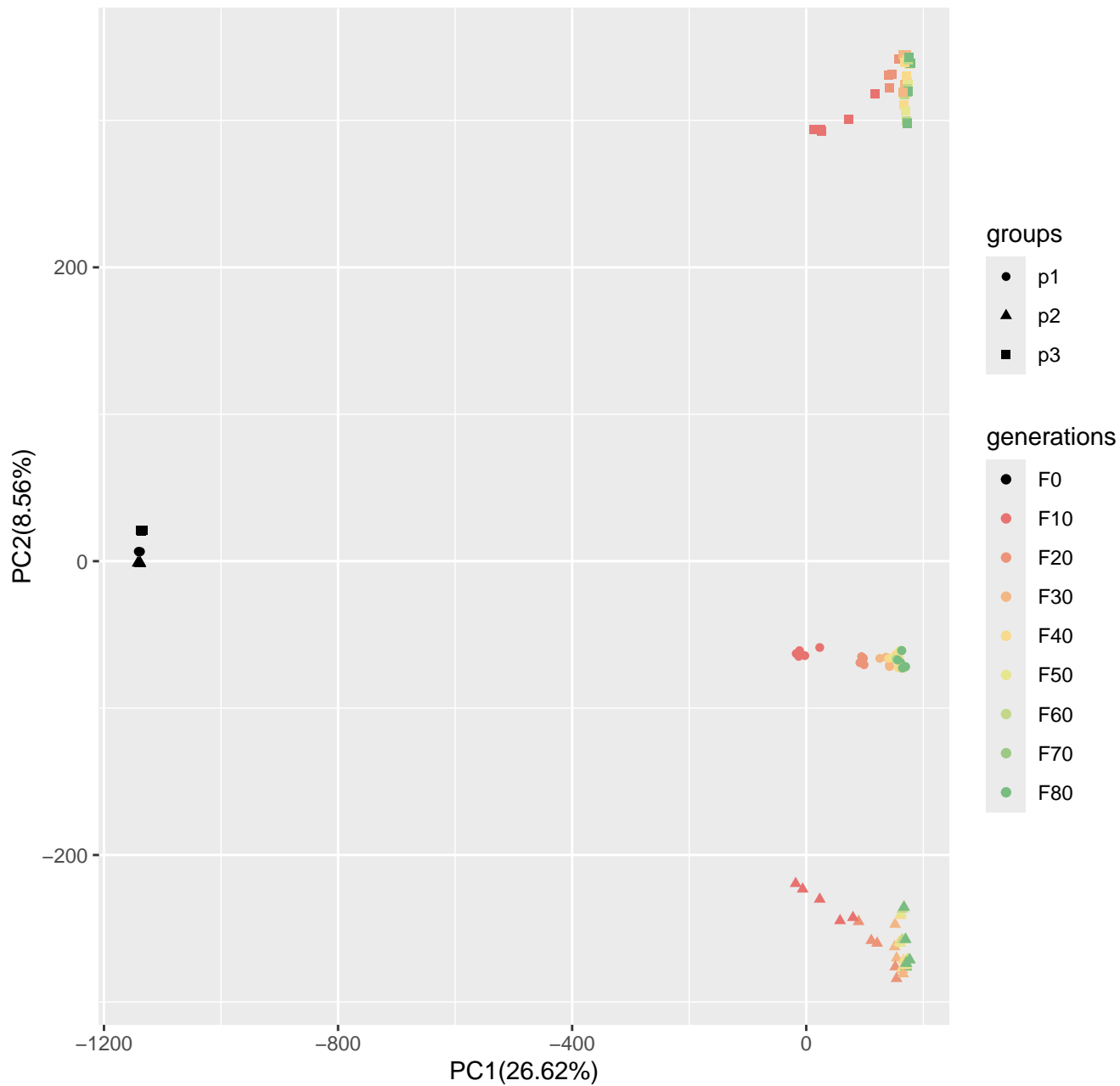
Run2_popsizel250_n400_100loci_s100
