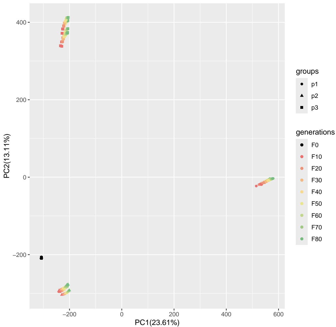
Run5_popsizel250_n400_10loci_s50
