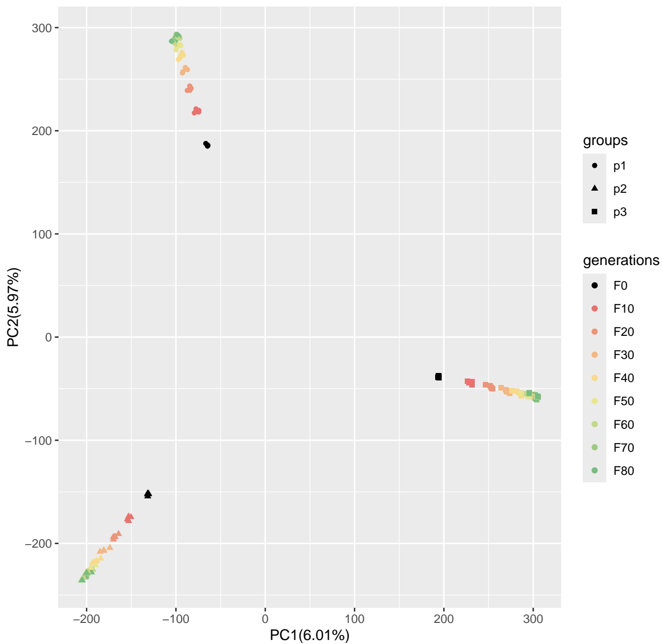
Run6_popsizel250_n400_10000loci_s50
