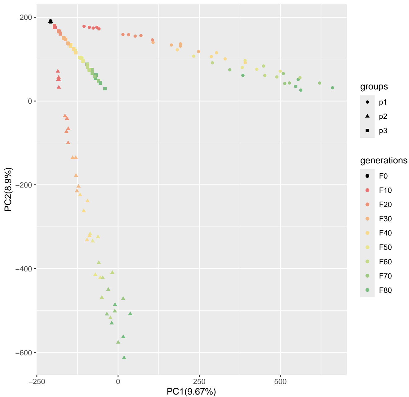
Run7_popsizel250_n400_100loci_s10
