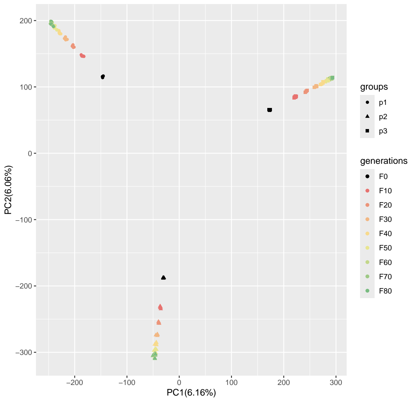
Run9_popsizel250_n400_100loci_s10
