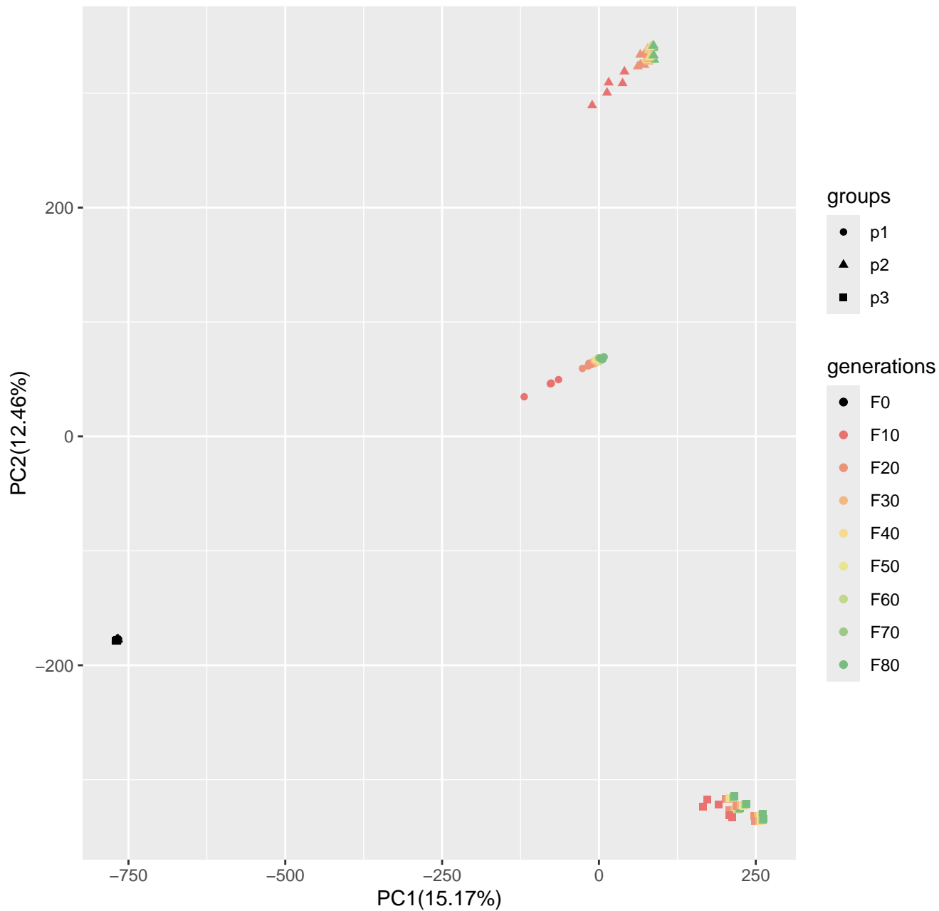
Run1_popsizel250_n400_100loci_s100
