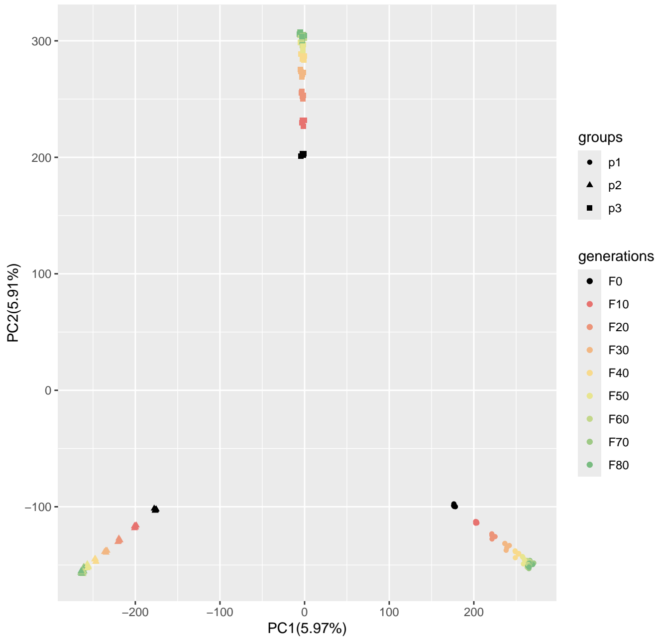
Run10_popsizel250_n400_10loci_s0
