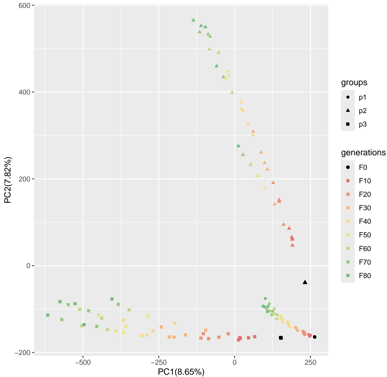
Run10_popsizel250_n400_100loci_s10
