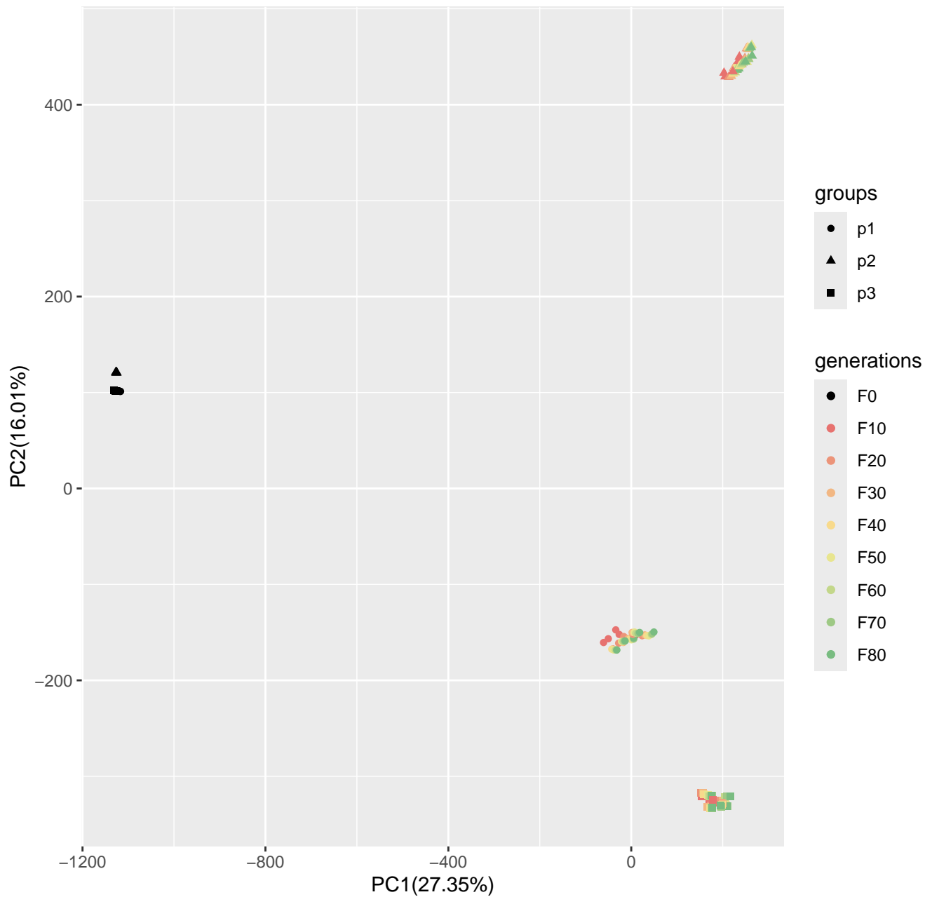
Run8_popsizel250_n400_10loci_s100
