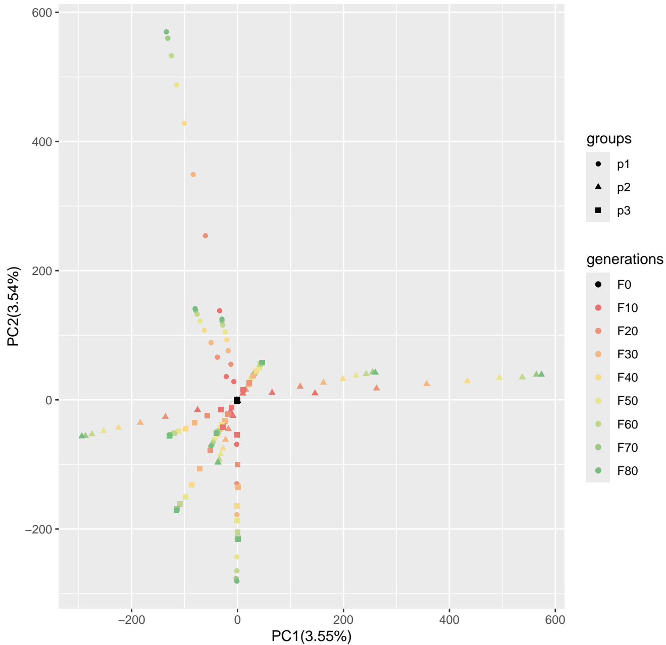
Run6_popsizel250_n400_10loci_s0
