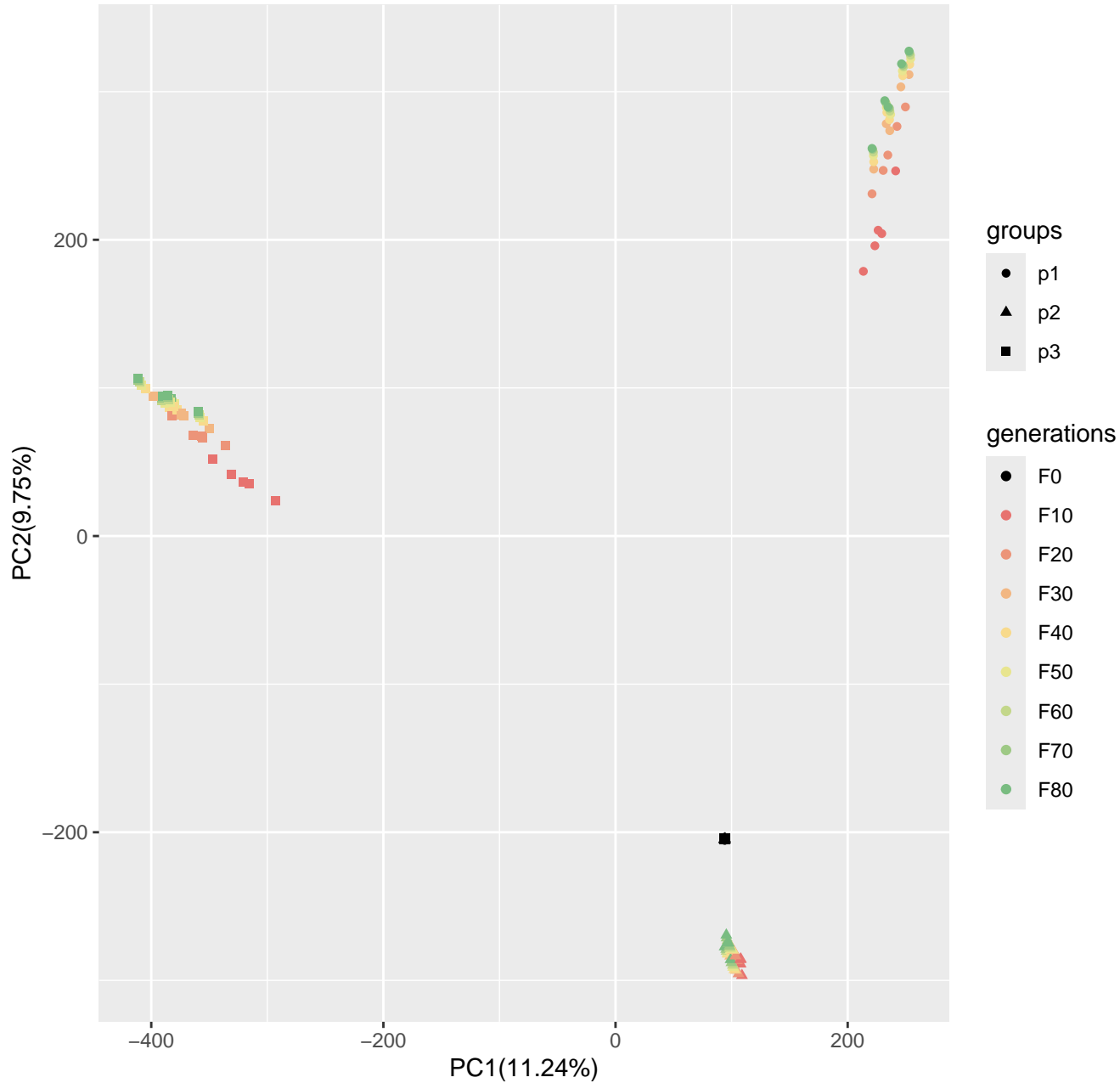
Run10_popsizel250_n400_100loci_s50
