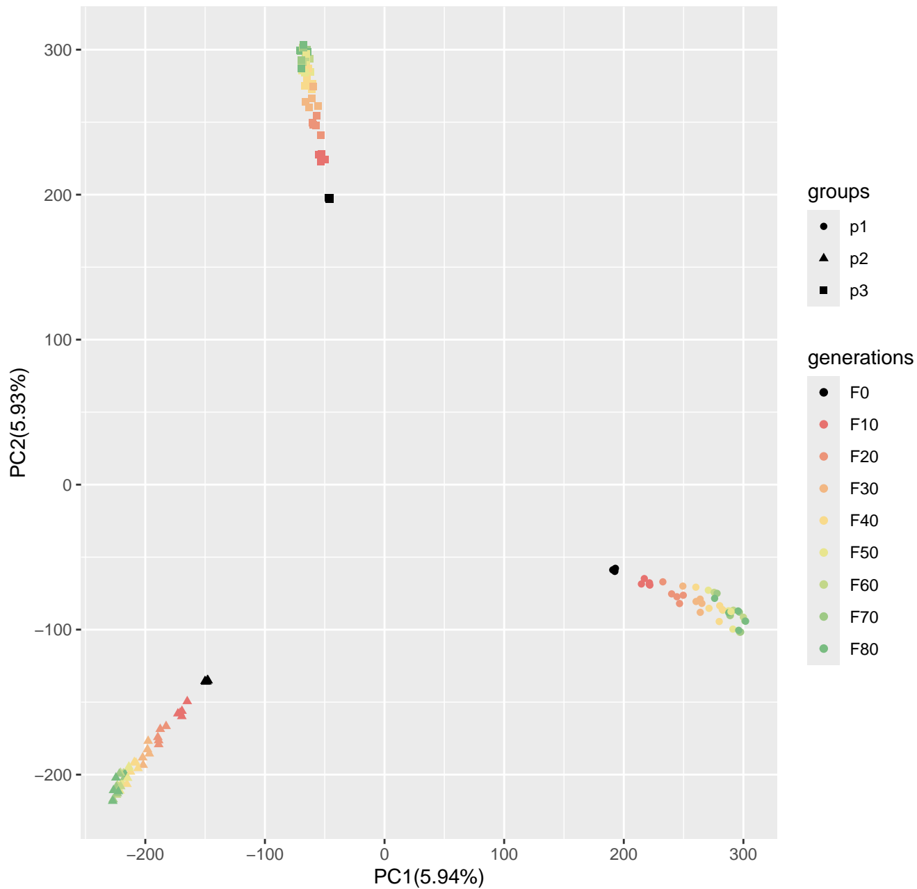
Run3_popsizel250_n400_10loci_s0
