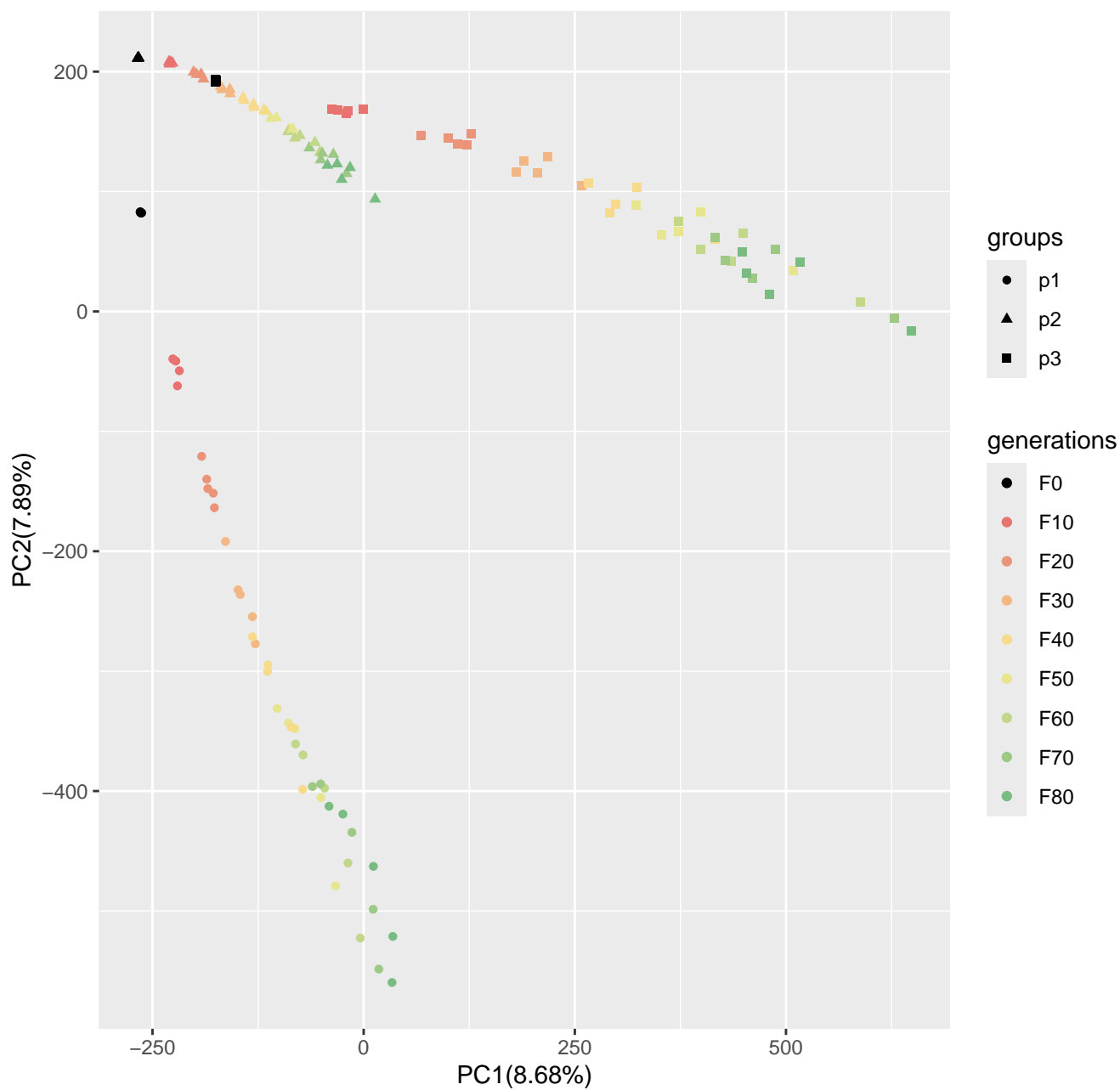
Run6_popsizel250_n400_100loci_s10
