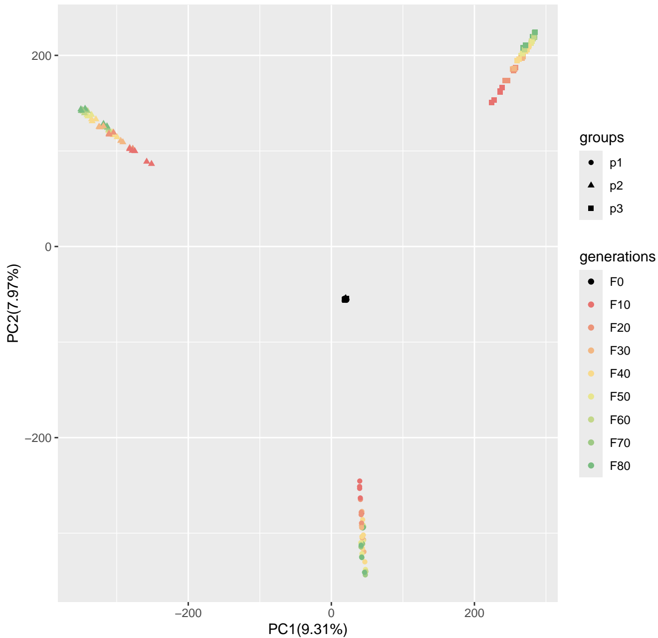
Run9_popsizel250_n400_10loci_s10
