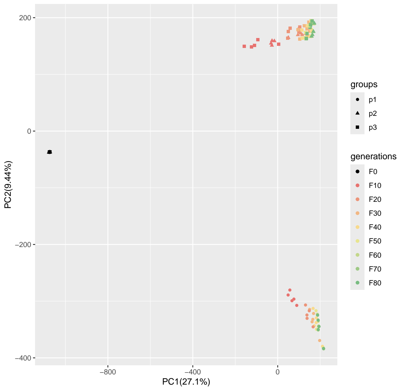
Run8_popsizel250_n400_100loci_s100
