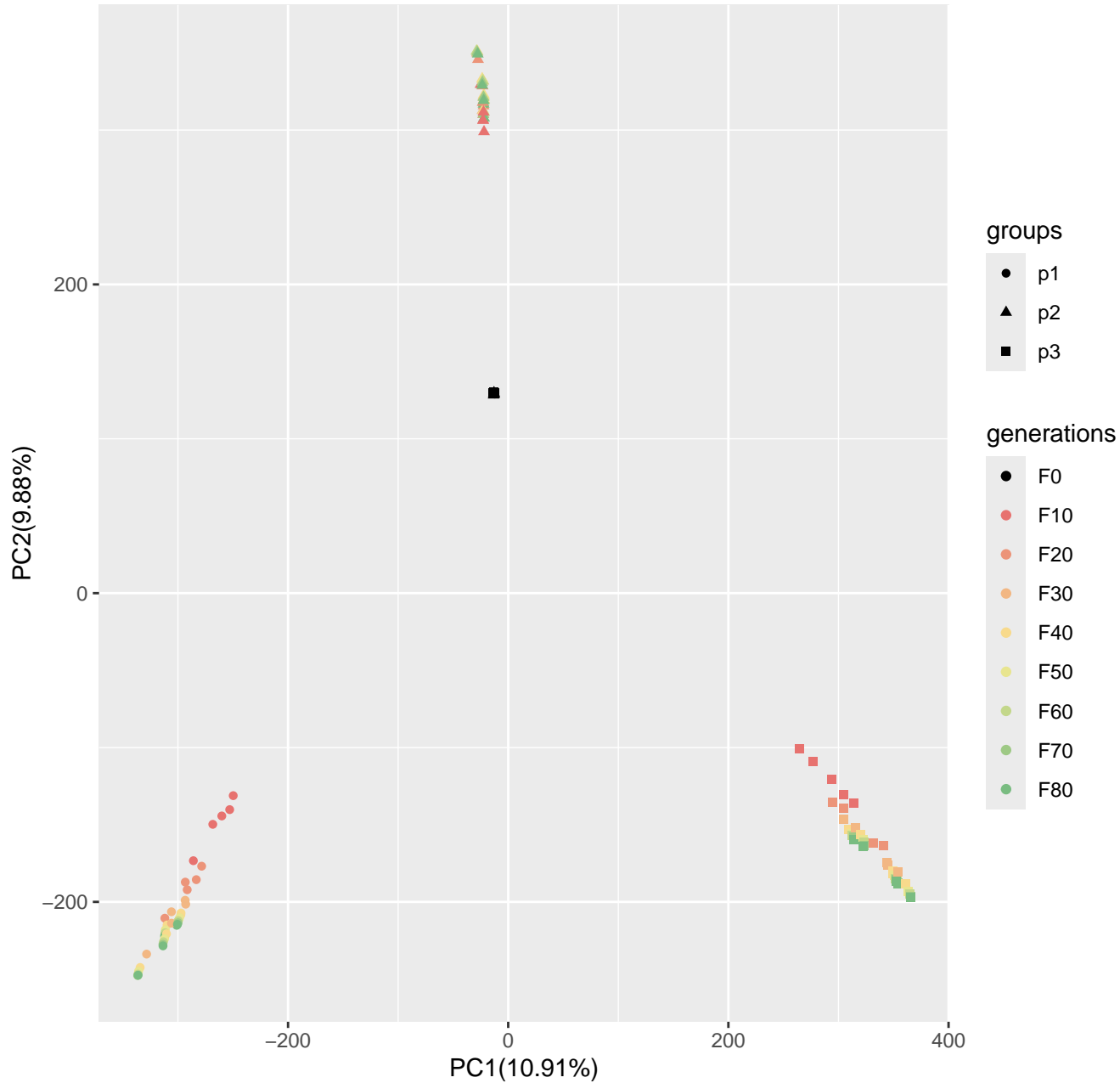
Run9_popsizel250_n400_100loci_s50
