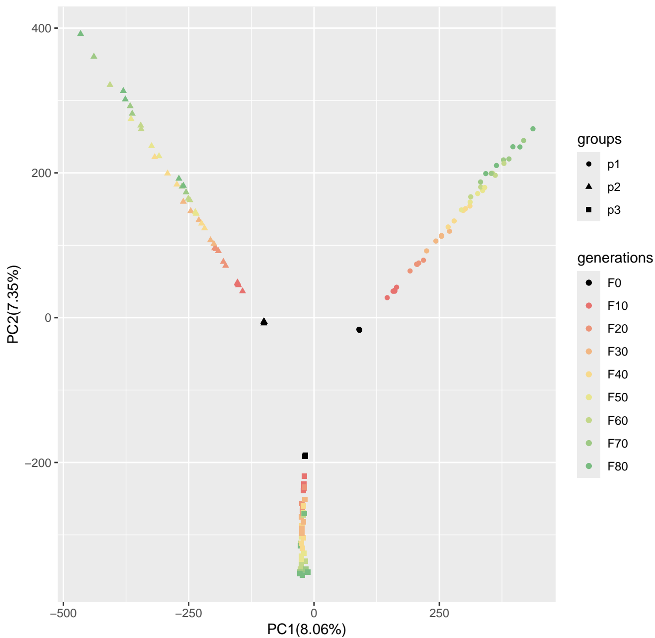
Run9_popsizel250_n400_5000loci_s50
