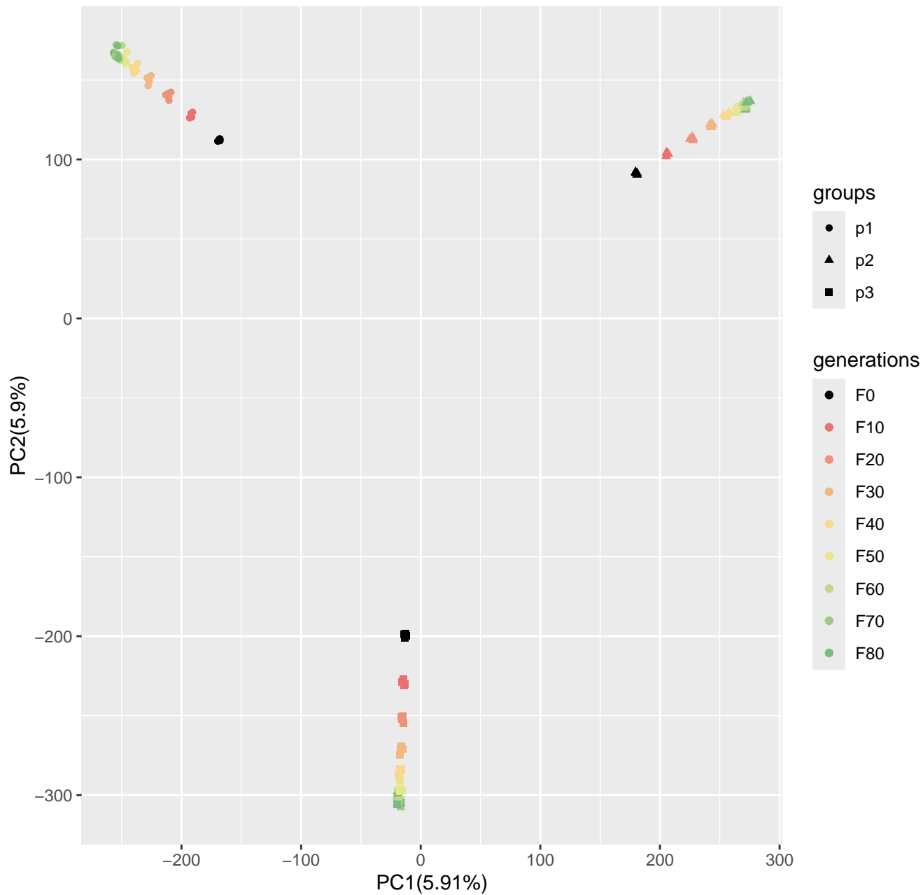
Run9_popsizel250_n400_5000loci_s10
