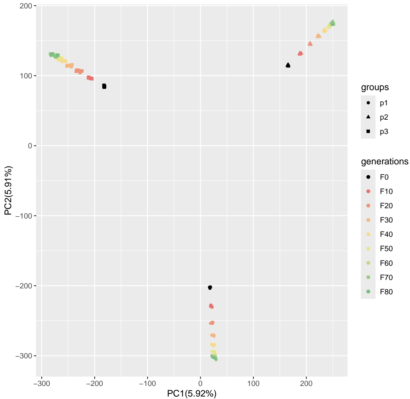
Run9_popsizel250_n400_20000loci_s10
