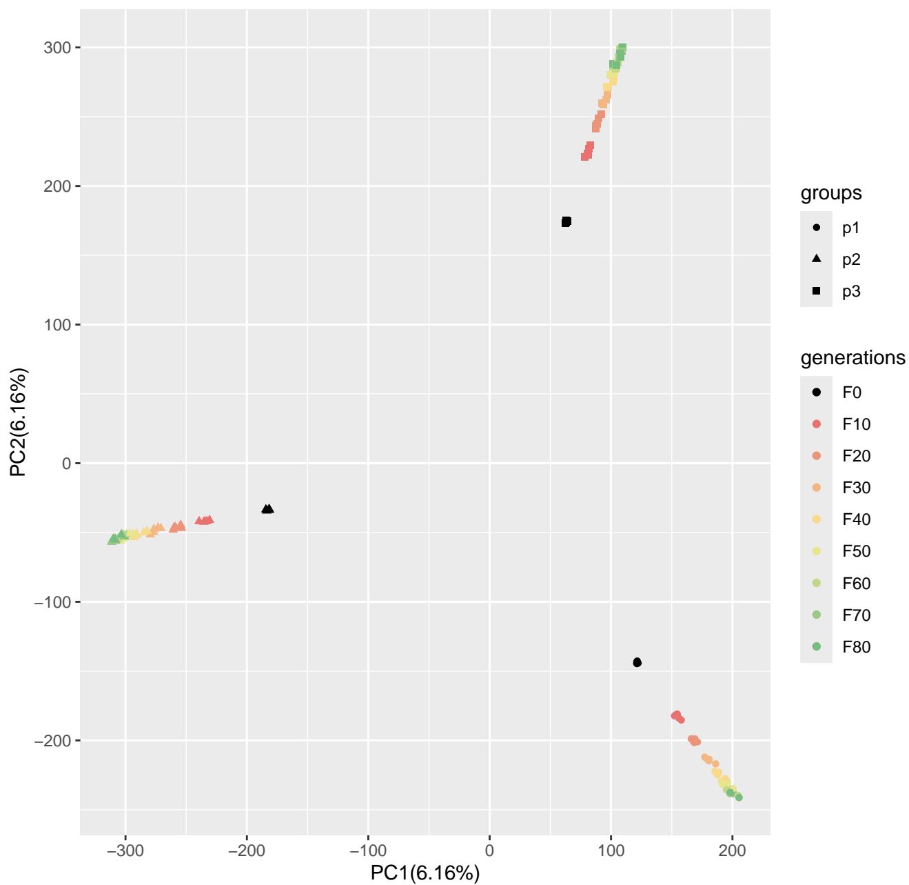
Run9_popsizel250_n400_10000loci_s100
