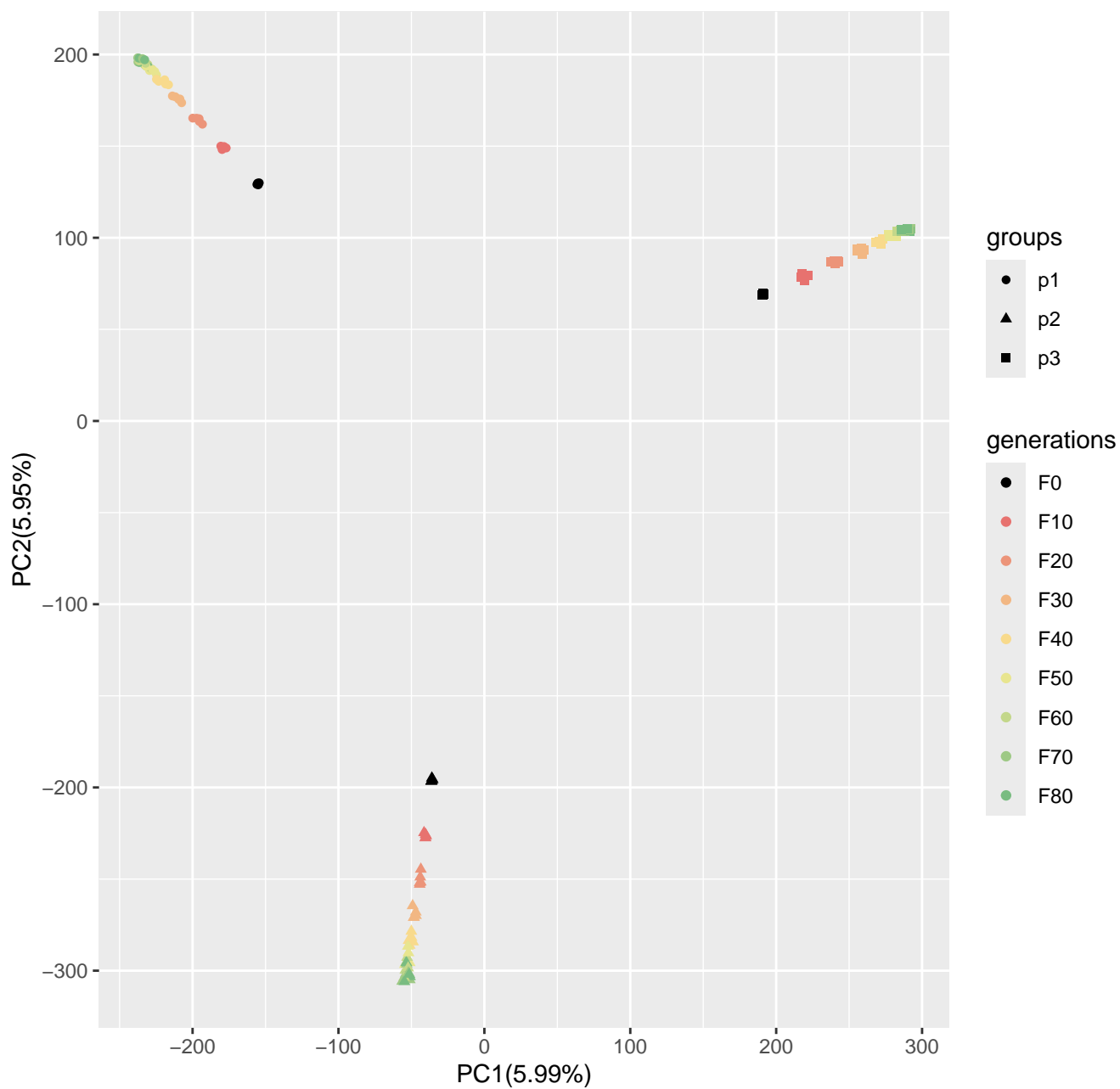
Run6_popsizel250_n400_20000loci_s50
