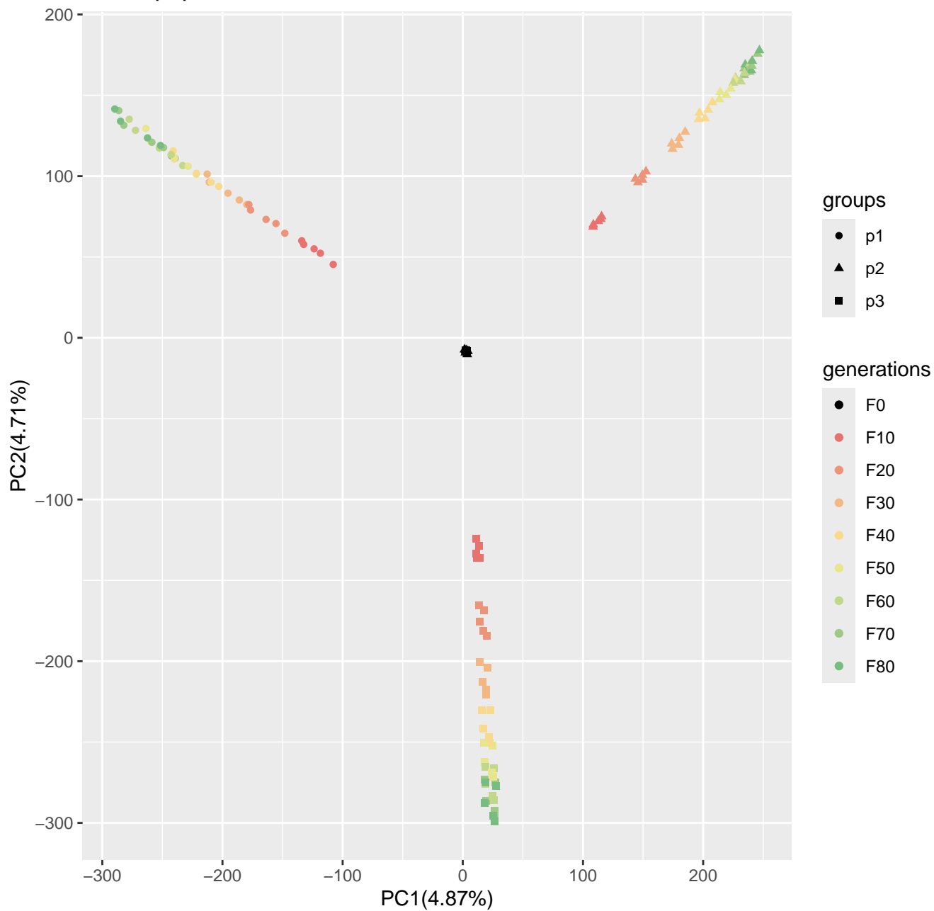
Run9_popsizel250_n400_1000loci_s50
