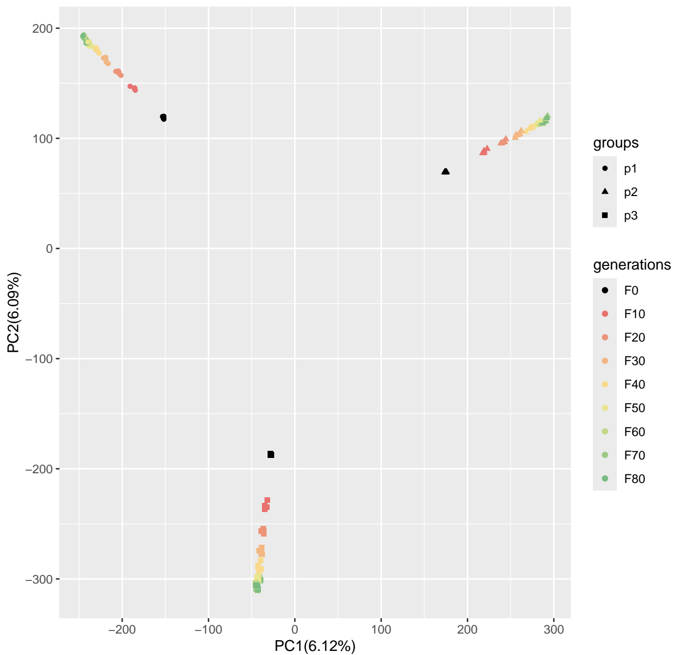
Run8_popsizel250_n400_100loci_s10
