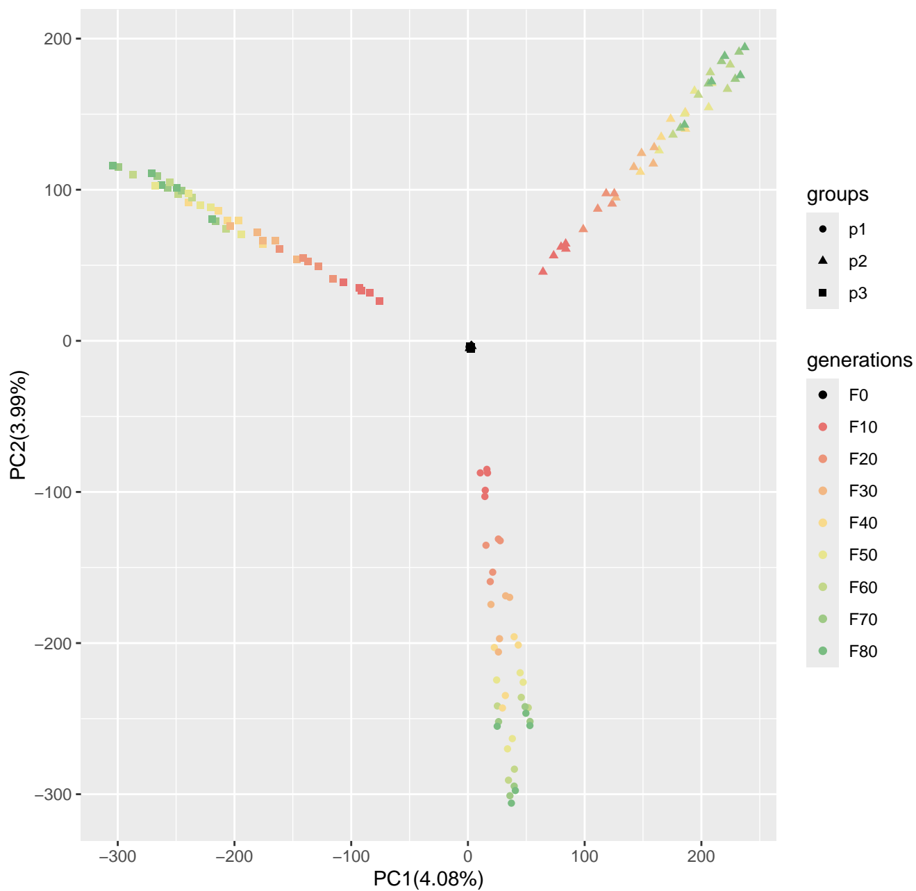
Run5_popsizel250_n400_100loci_s10
