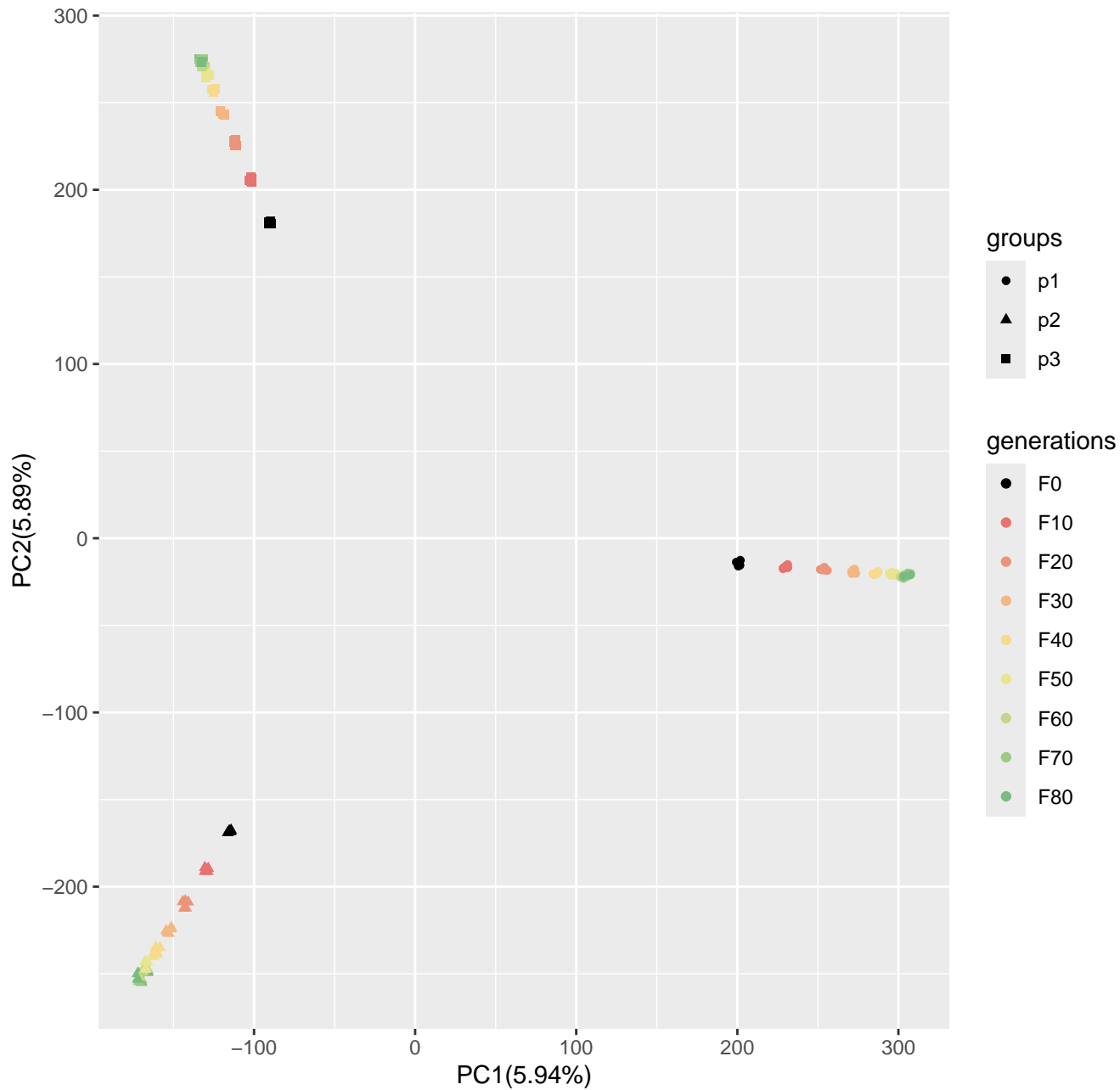
Run10_popsizel250_n400_5000loci_s10
