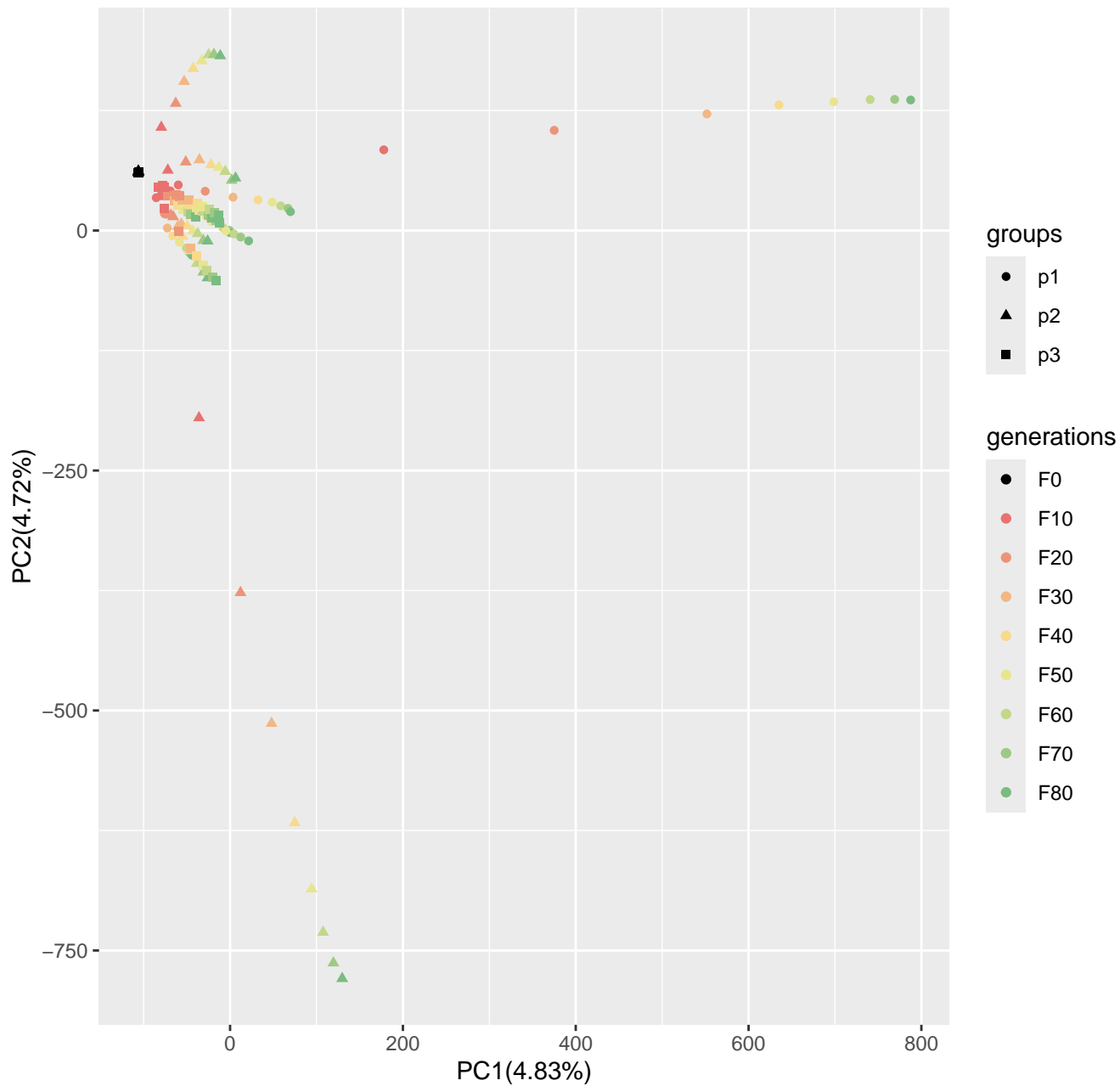
Run10_popsiz300_n400_10loci_s0
