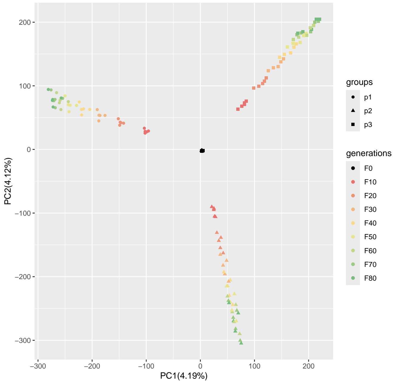
Run3_popsizel250_n400_100loci_s10
