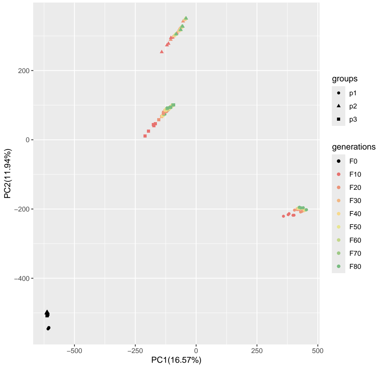
Run6_popsizel250_n400_100loci_s100
