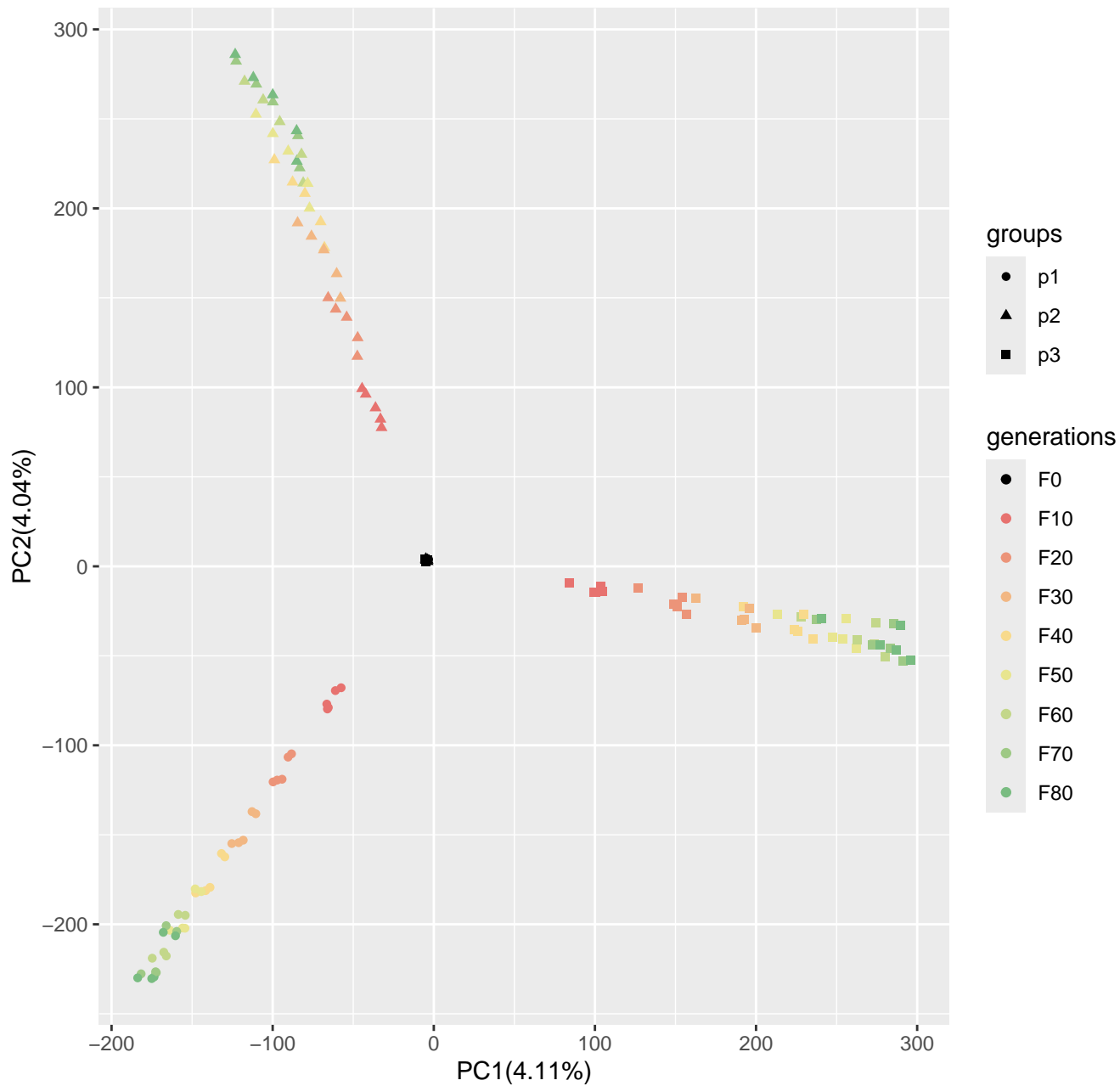
Run1_popsizel250_n400_100loci_s10
