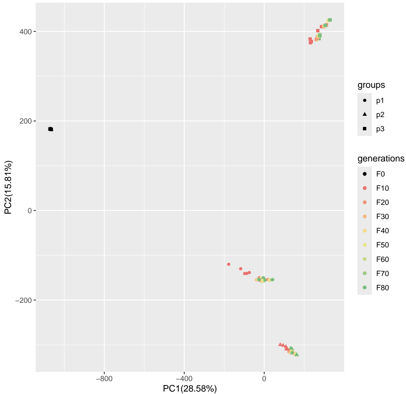
Run6_popsizel250_n400_10loci_s50
