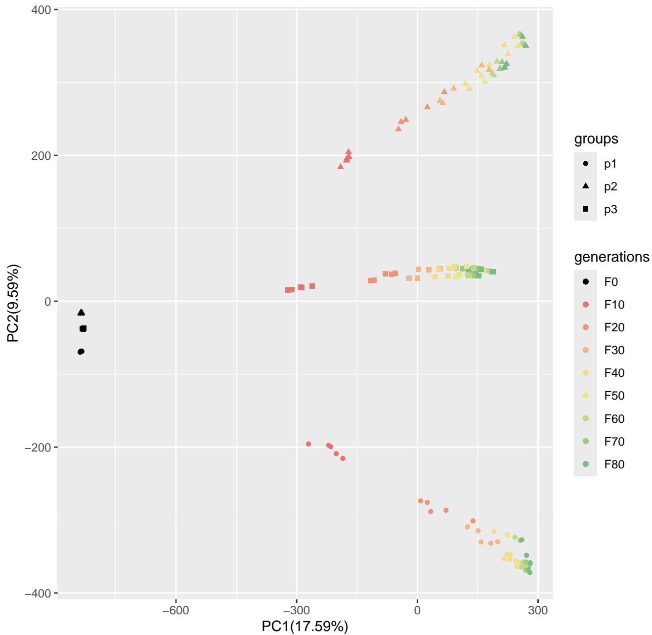
Run6_popsizel250_n400_1000loci_s100
