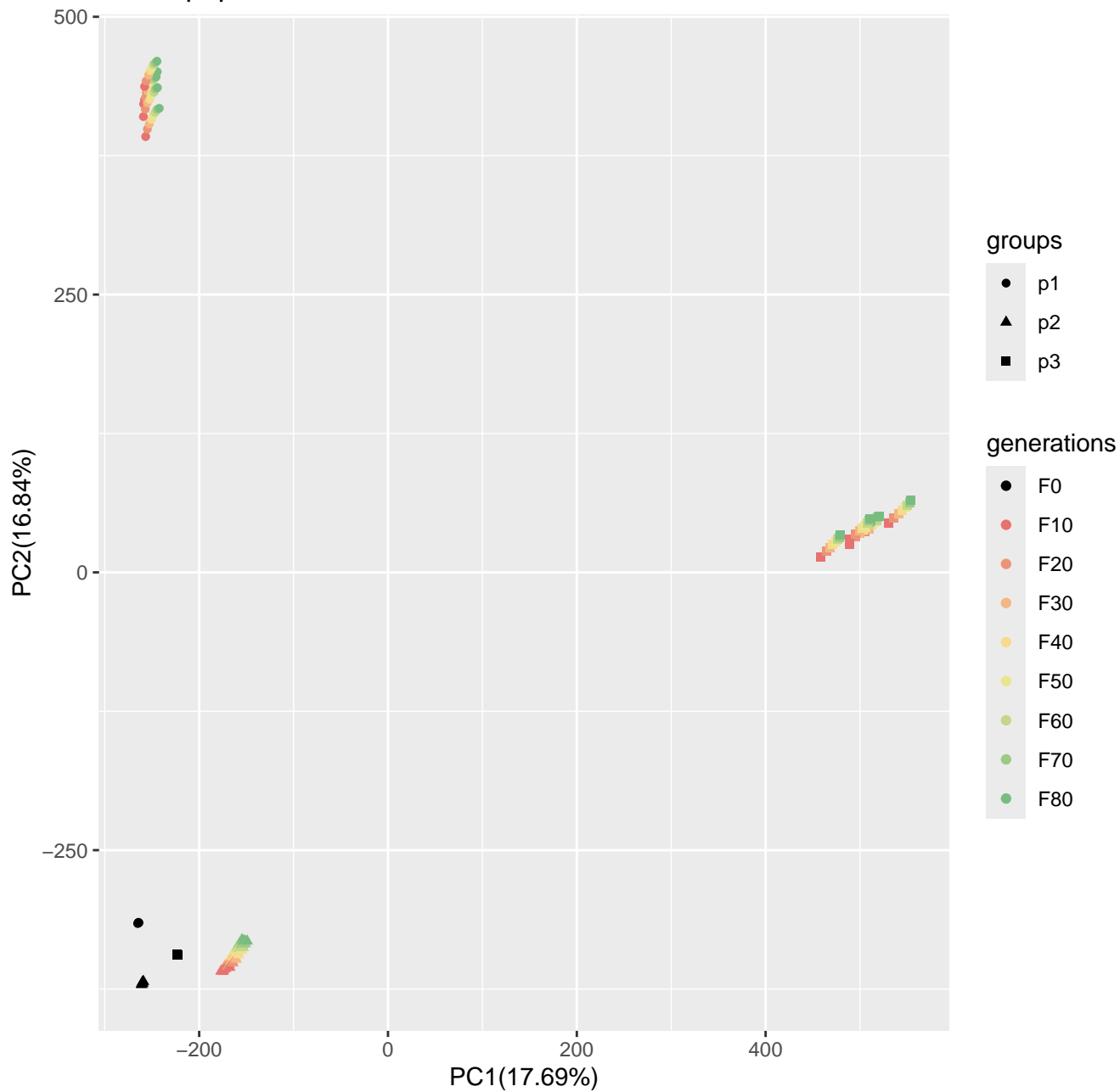
Run4_popsizel250_n400_10loci_s100
