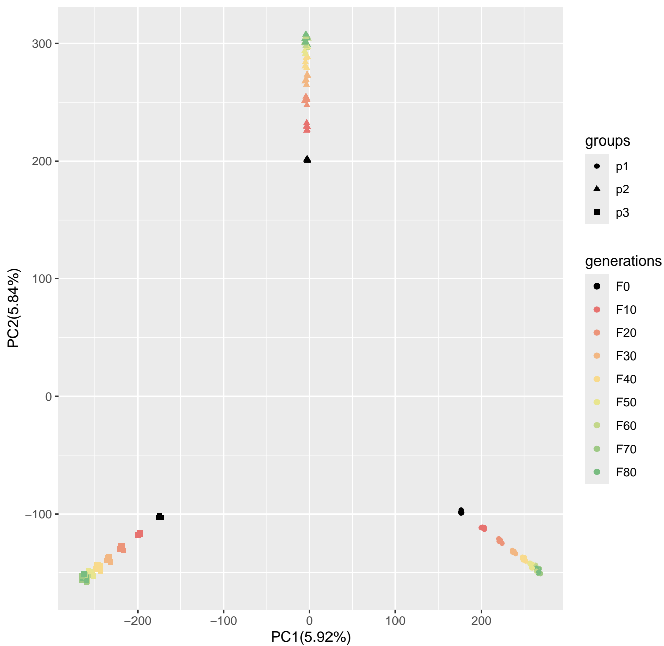
Run1_popsizel250_n400_10loci_s0
