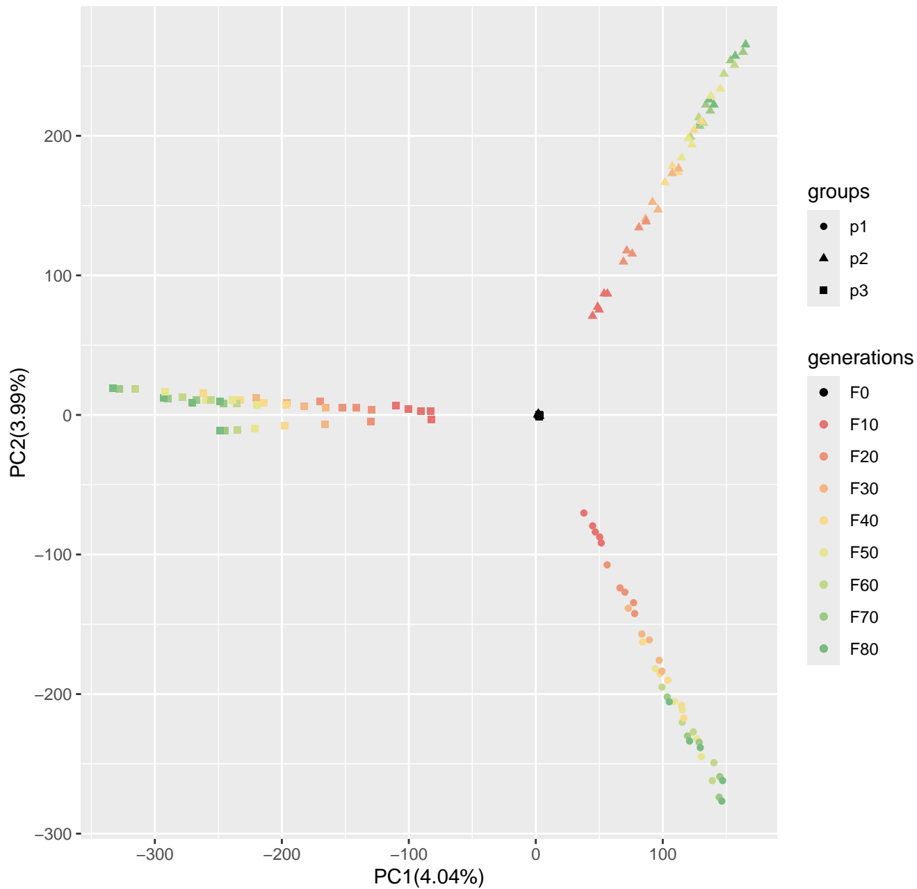
Run9_popsizel250_n400_100loci_s10
