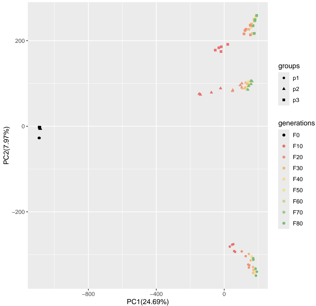
Run5_popsizel250_n400_100loci_s100
