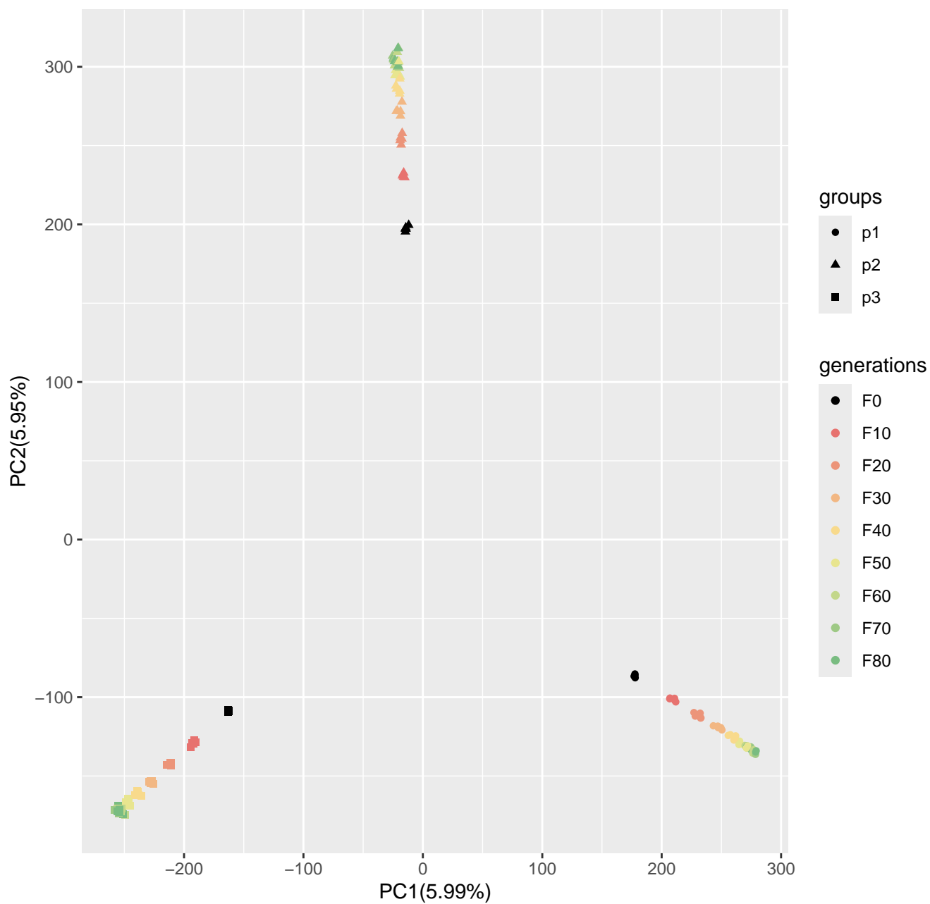
Run9_popsizel250_n400_10000loci_s50
