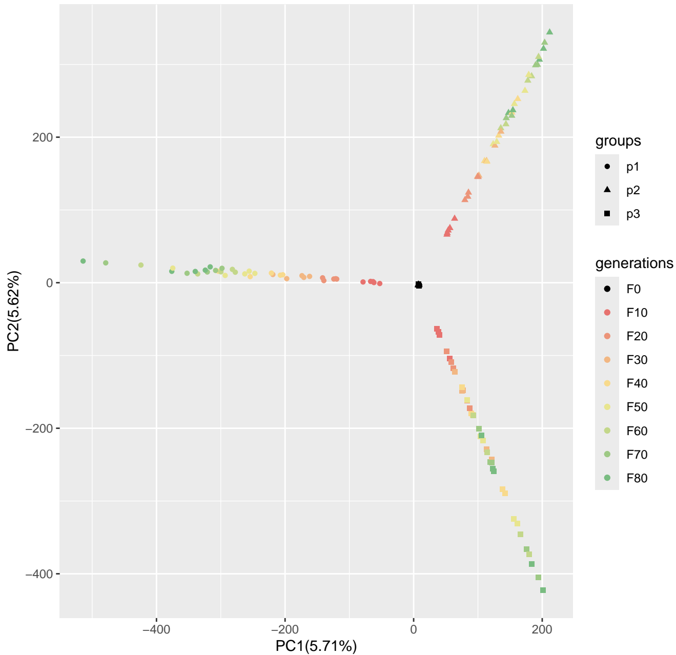
Run6_popsizel250_n400_10000loci_s50
