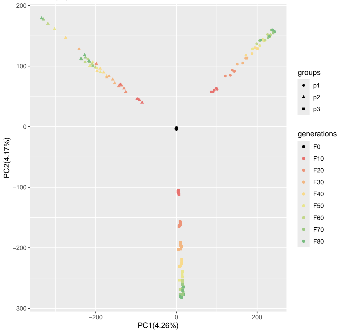
Run7_popsizel250_n400_10loci_s10
