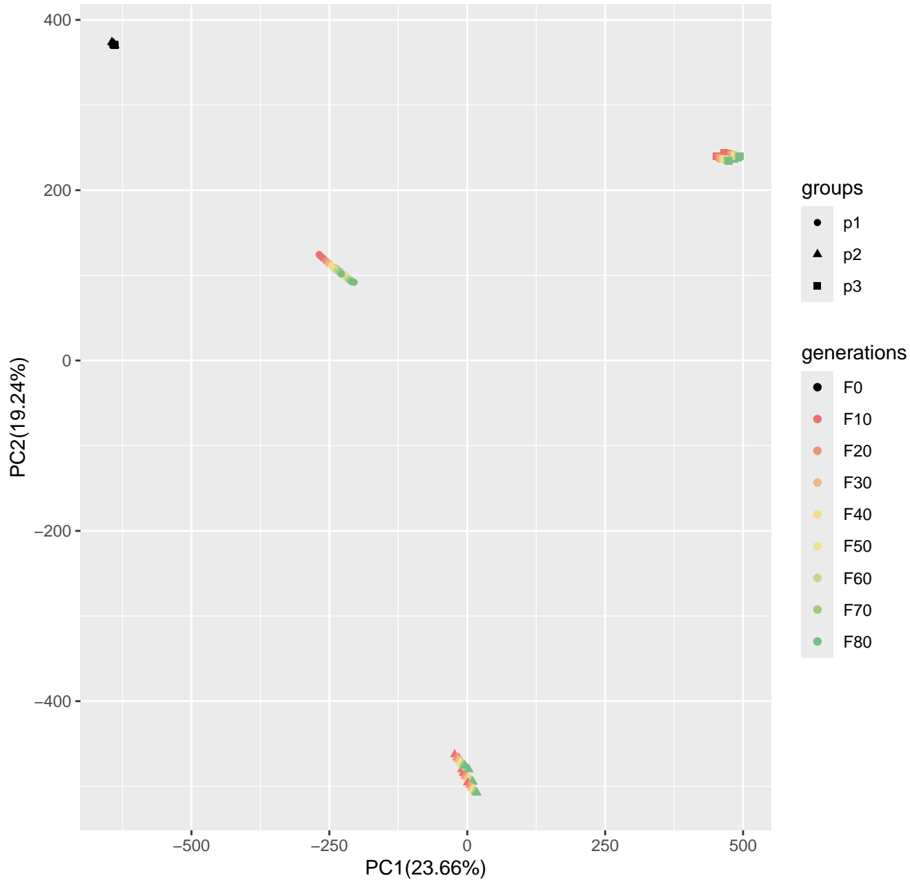
Run6_popsizel250_n400_10loci_s100
