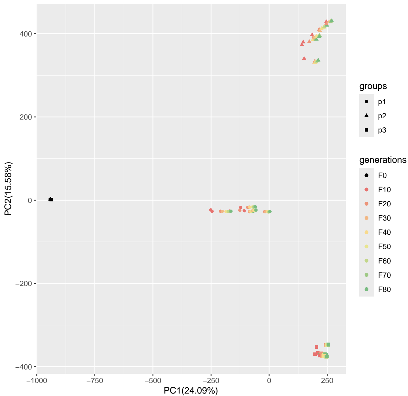
Run4_popsizel250_n400_10loci_s100
