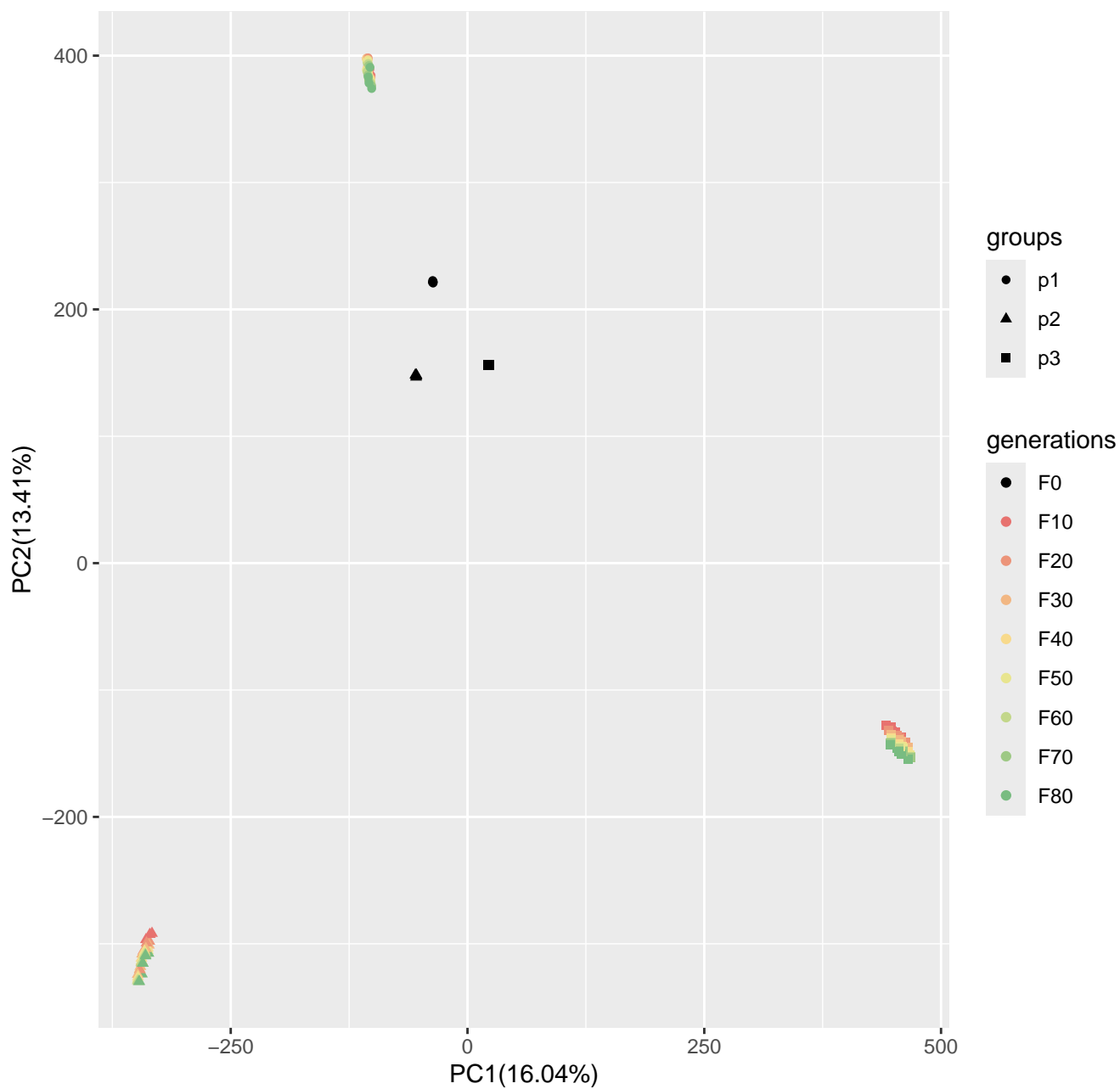
Run9_popsizel250_n400_10loci_s50
