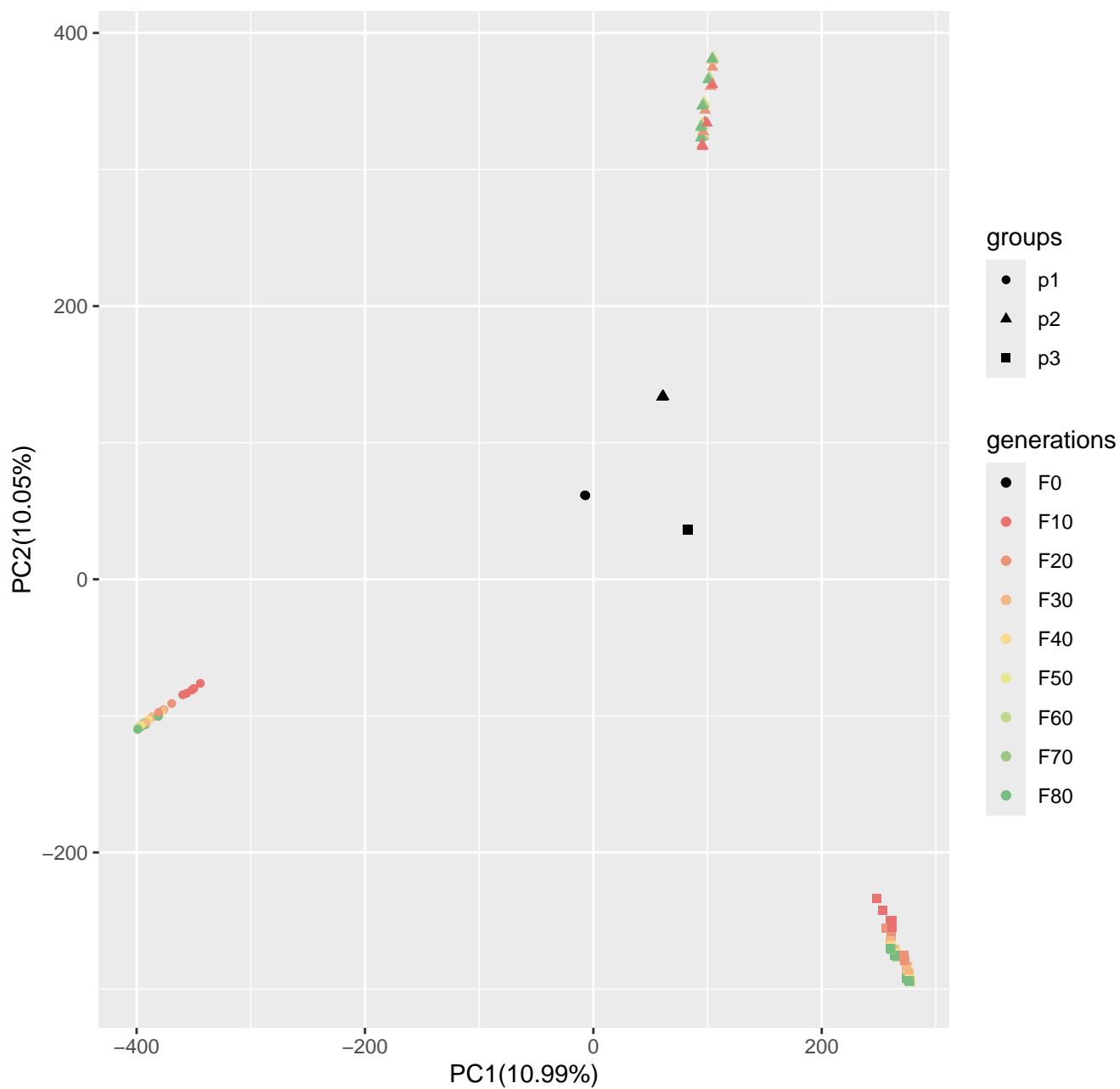
Run3_popsizel250_n400_100loci_s50
