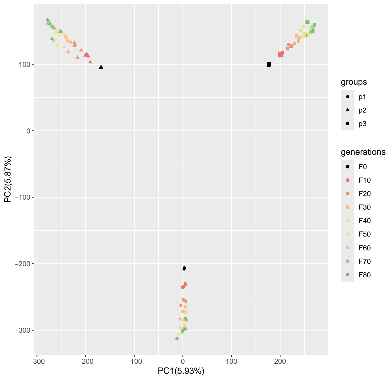
Run6_popsizel250_n400_10loci_s0
