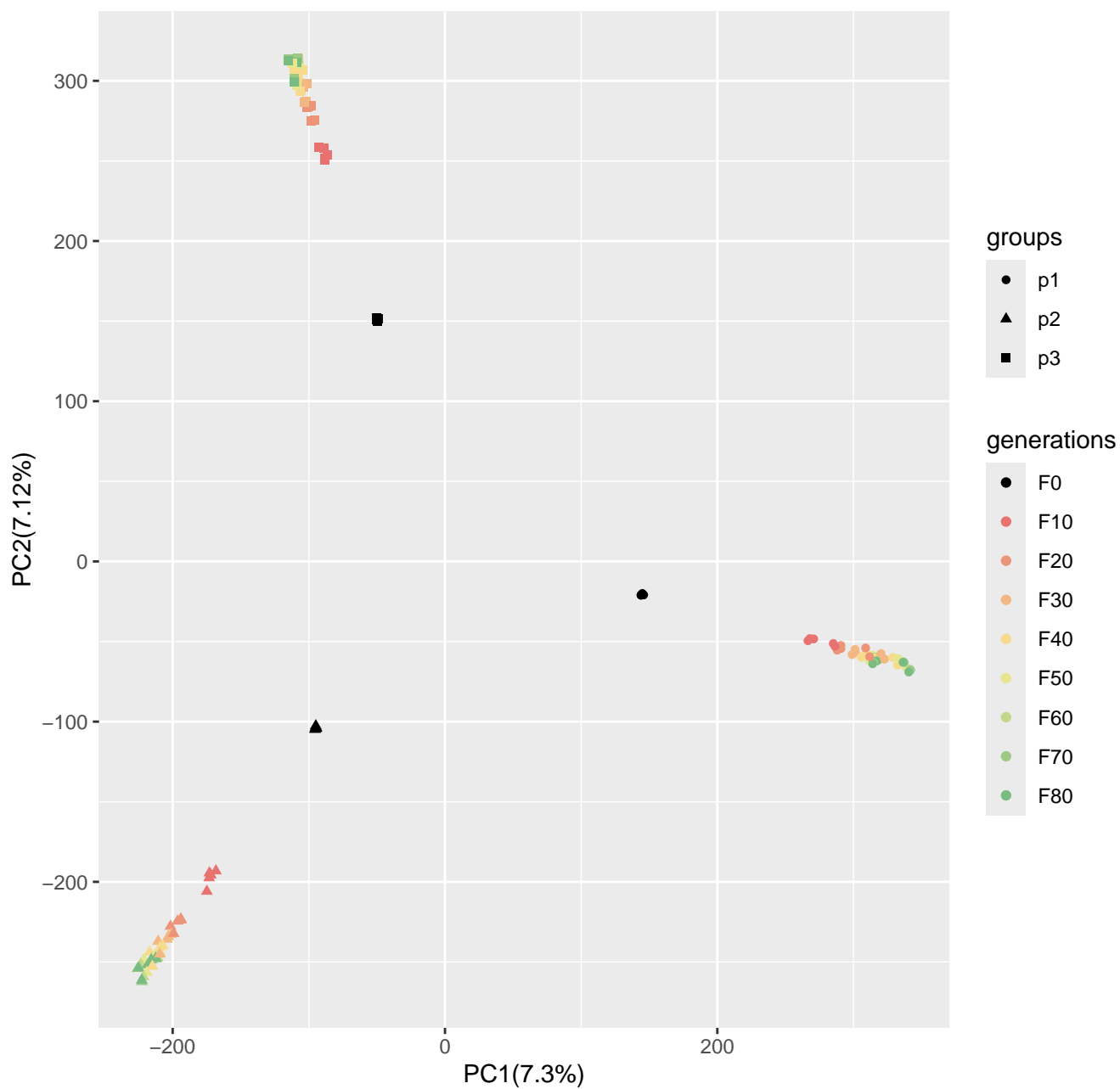
Run5_popsizel250_n400_10loci_s10
