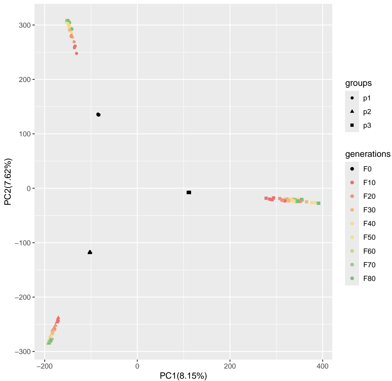
Run4_popsizel250_n400_10loci_s10
