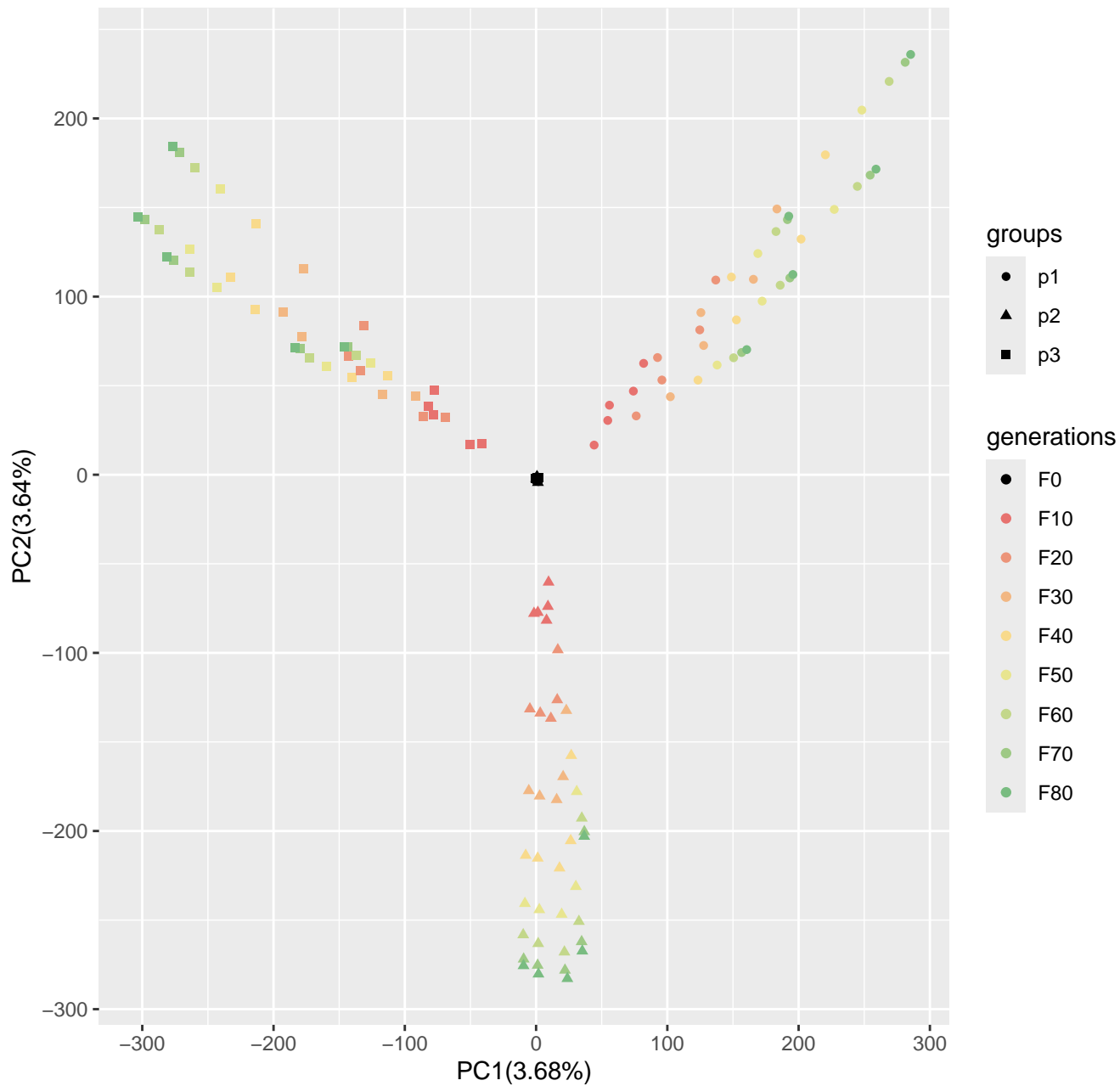
Run9_popsizel250_n400_10000loci_s50
