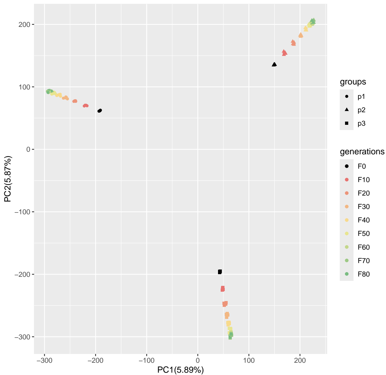
Run9_popsizel250_n400_10000loci_s10
