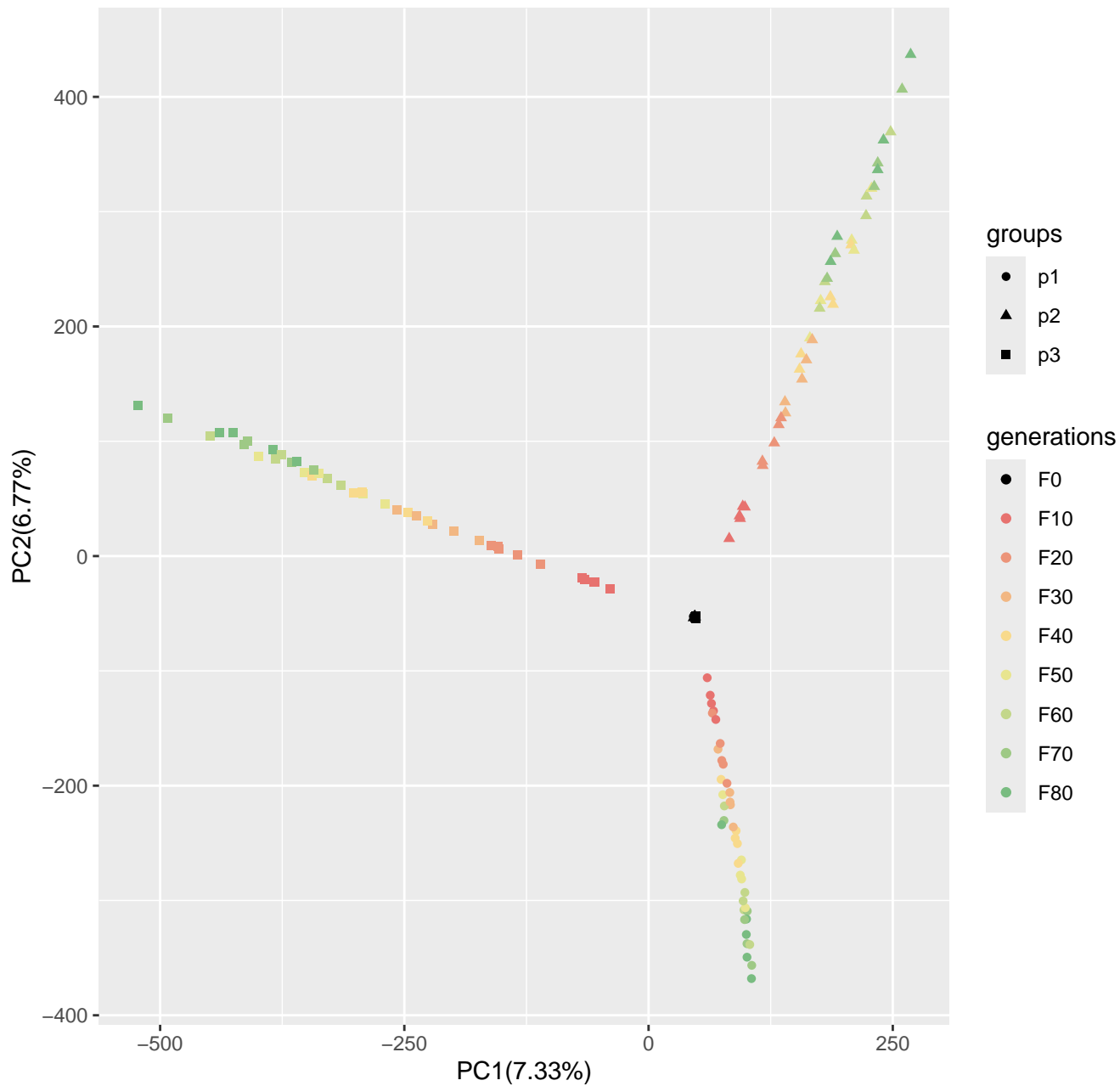
Run9_popsizel250_n400_5000loci_s50
