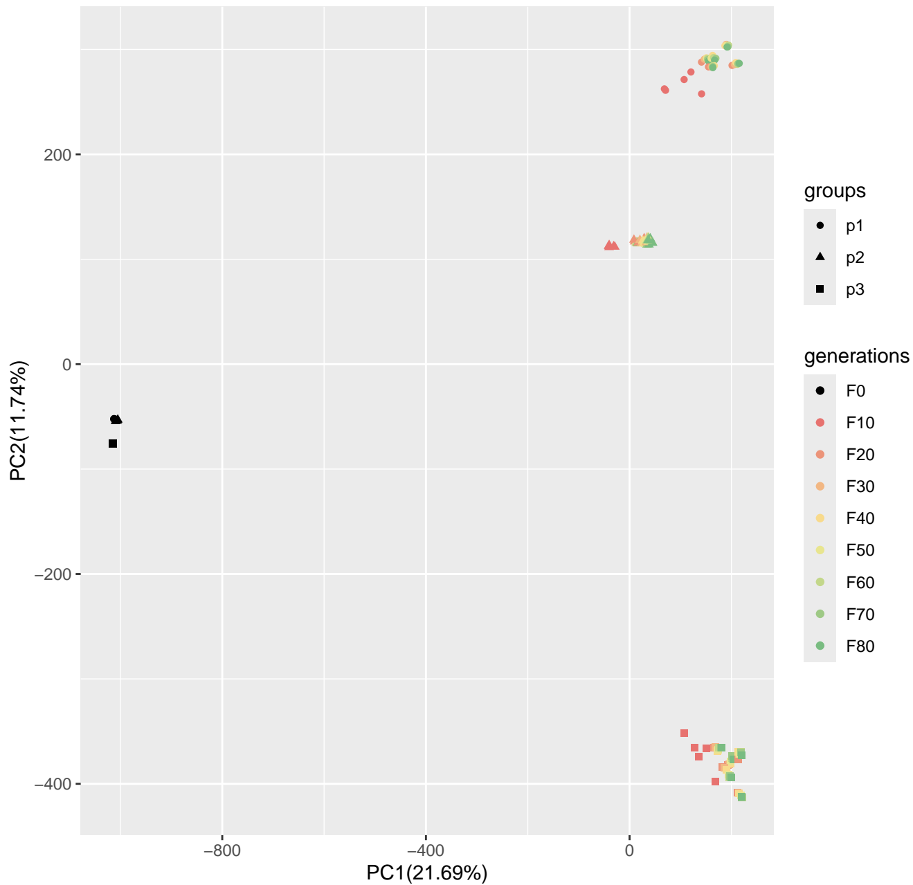
Run3_popsizel250_n400_10loci_s100
