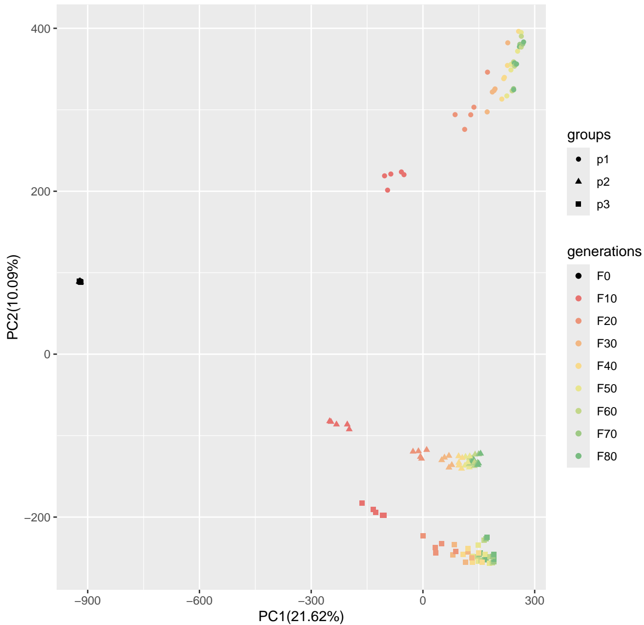
Run10_popsizel250_n400_100loci_s50
