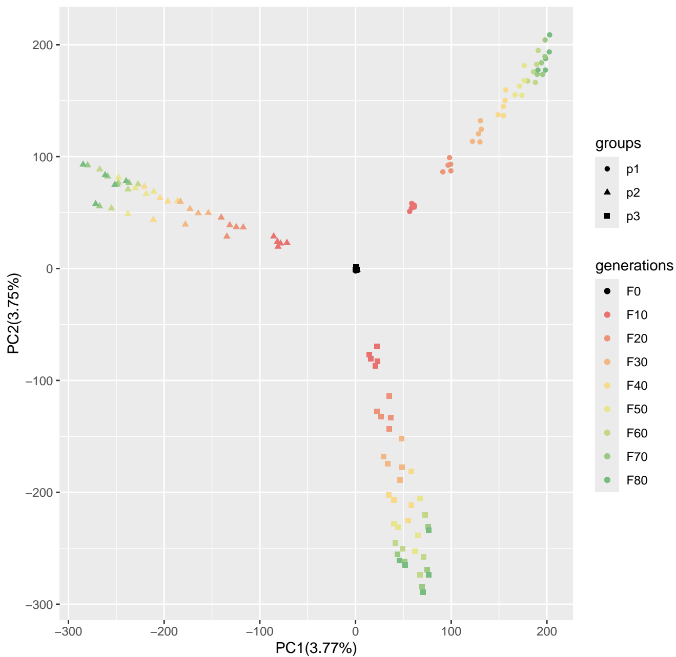
Run10_popsizel250_n400_5000loci_s50
