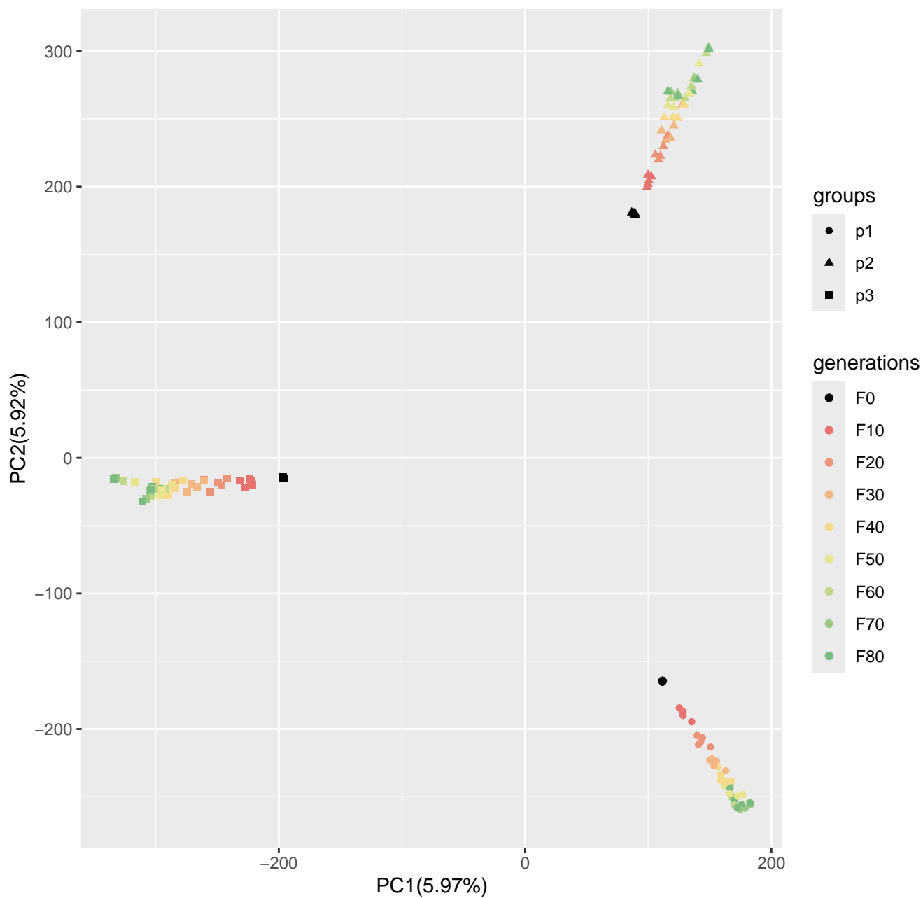
Run6_popsizel250_n400_5000loci_s10
