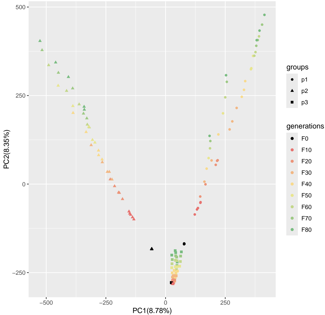
Run9_popsizel250_n400_10000loci_s100
