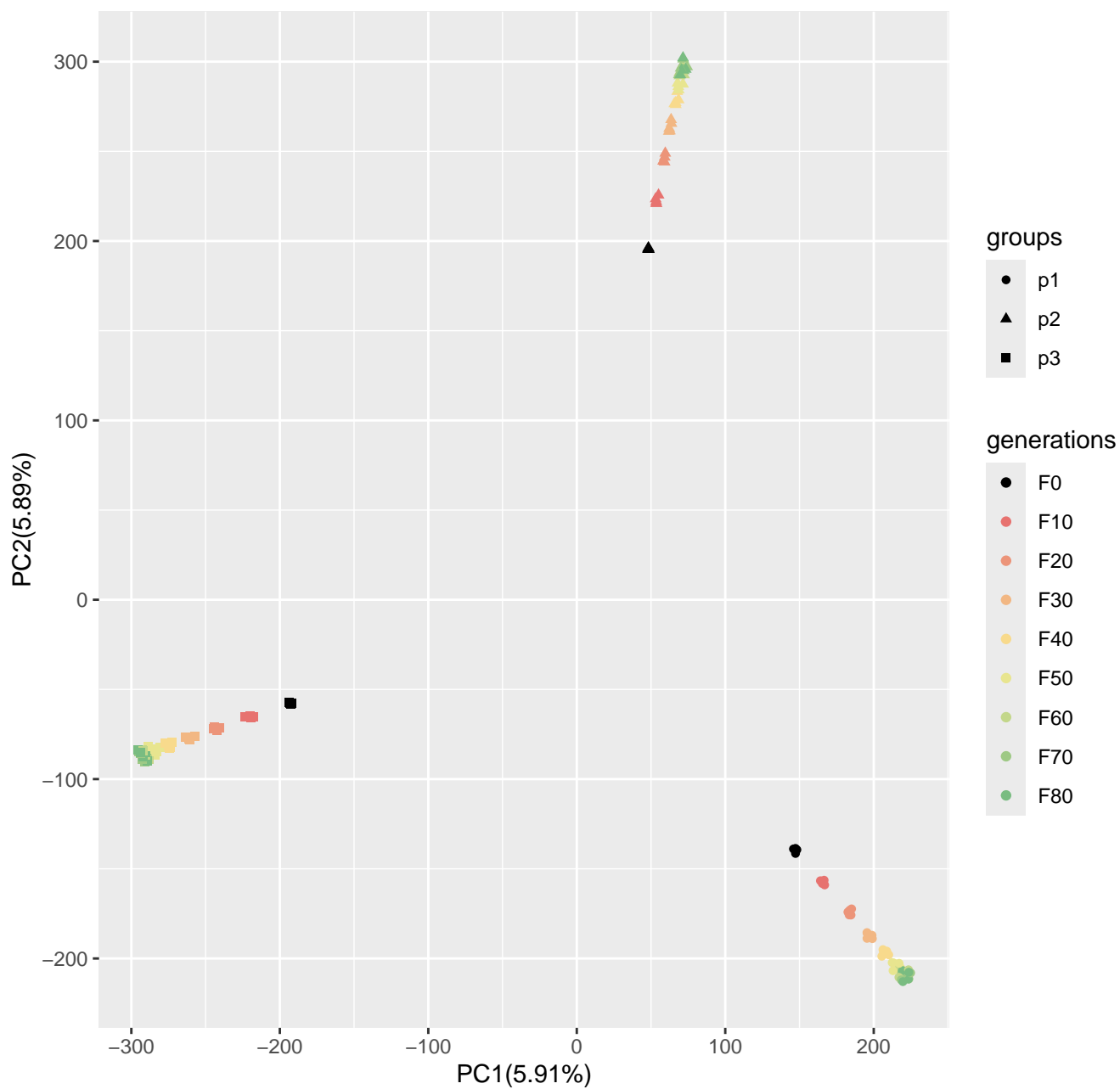
Run5_popsizel250_n400_10loci_s0
