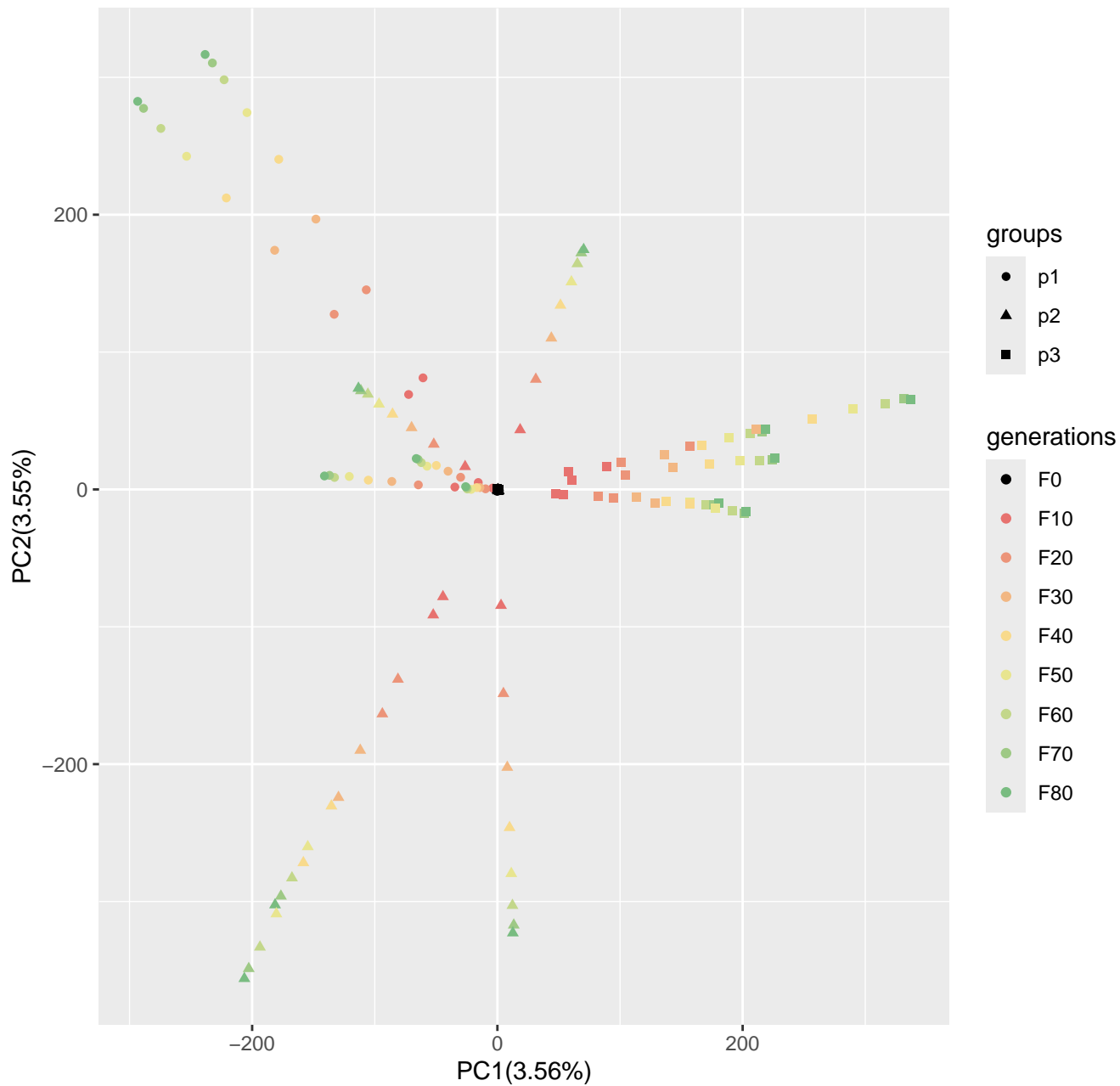
Run6_popsizel250_n400_1000loci_s10
