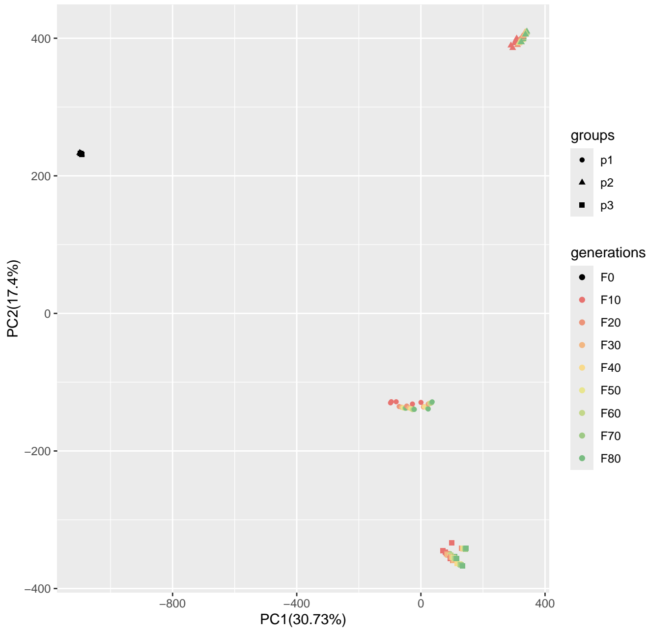
Run1_popsizel250_n400_10loci_s100
