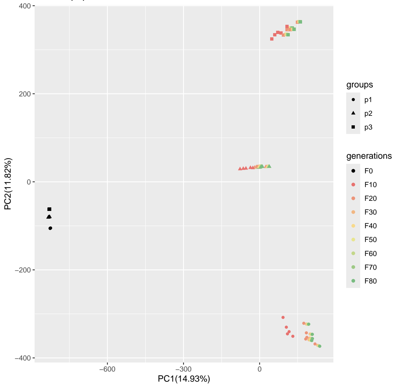
Run10_popsizel250_n400_100loci_s100
