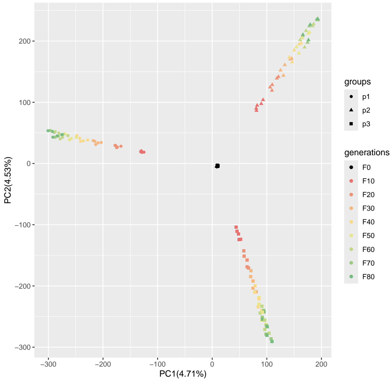
Run3_popsizel250_n400_5000loci_s100
