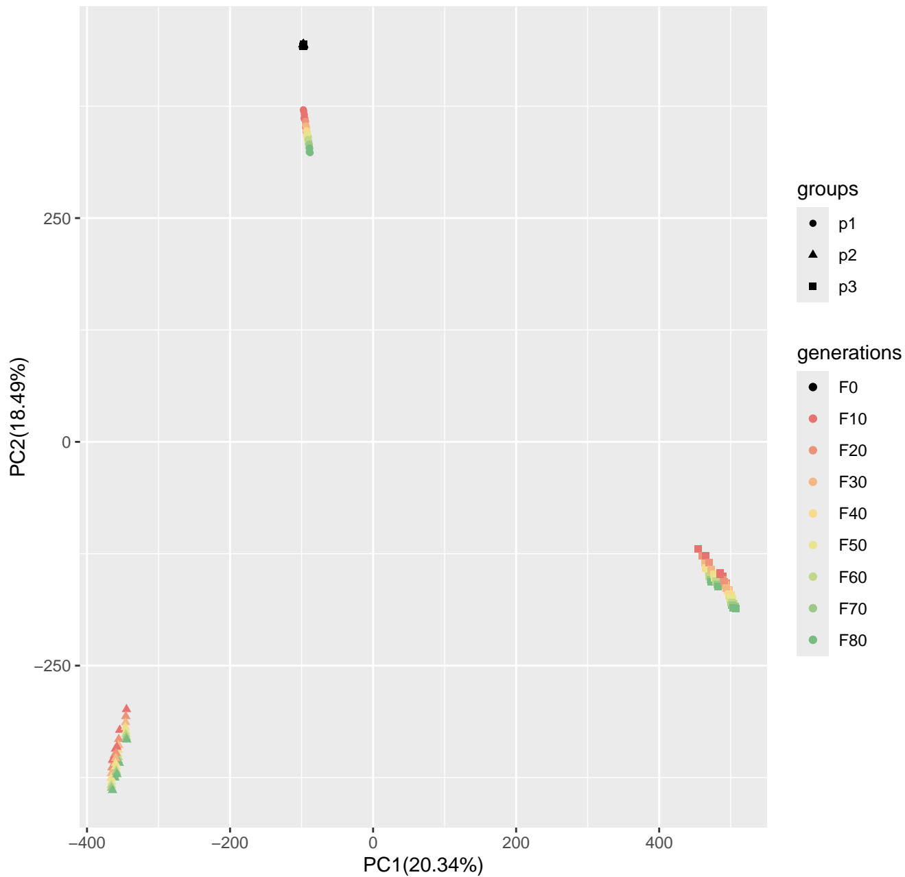
Run9_popsizel250_n400_10loci_s50
