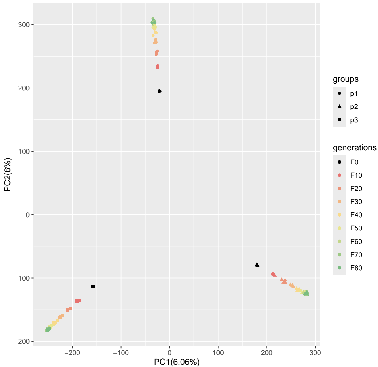
Run6_popsizel250_n400_5000loci_s50
