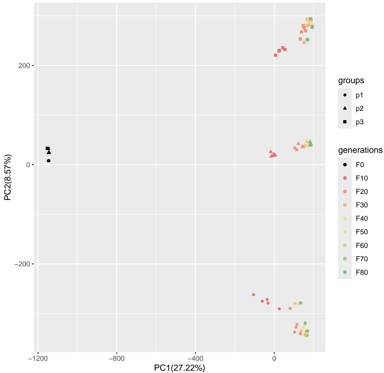
Run4_popsizel250_n400_100loci_s100
