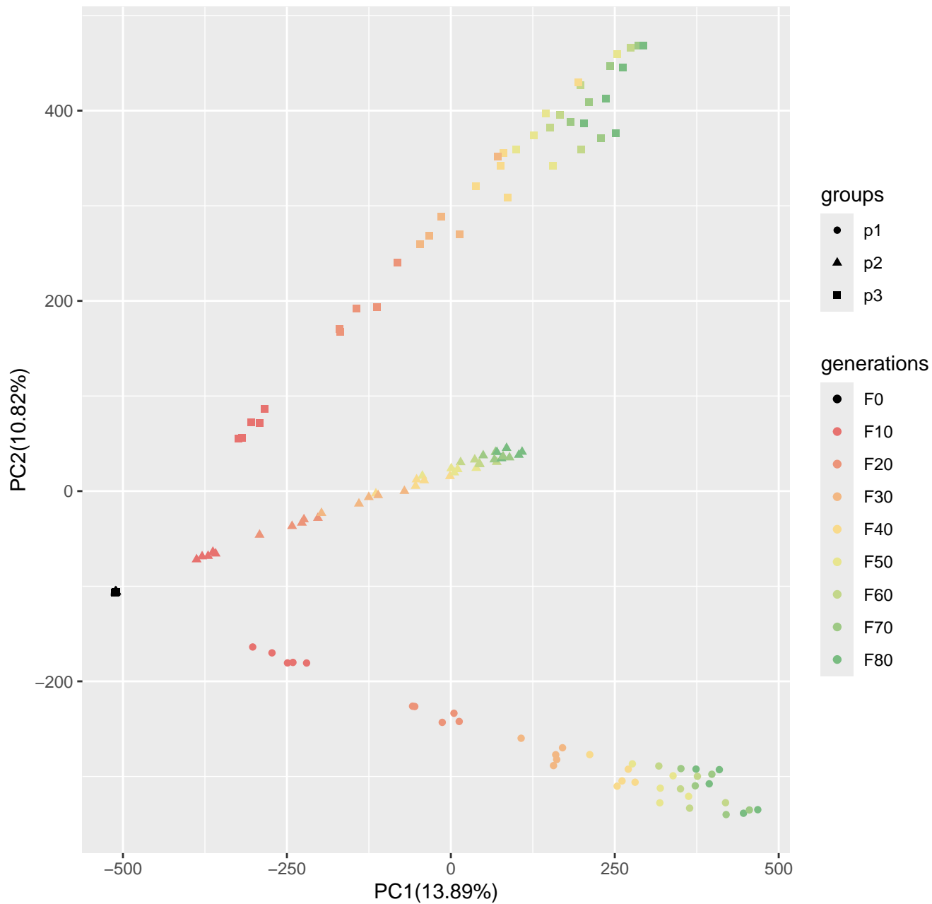
Run6_popsizel250_n400_1000loci_s50
