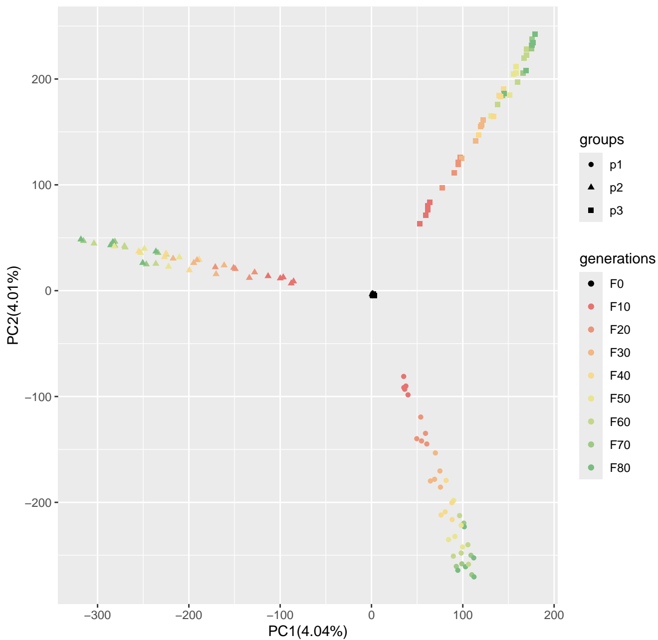
Run6_popsizel250_n400_10000loci_s100
