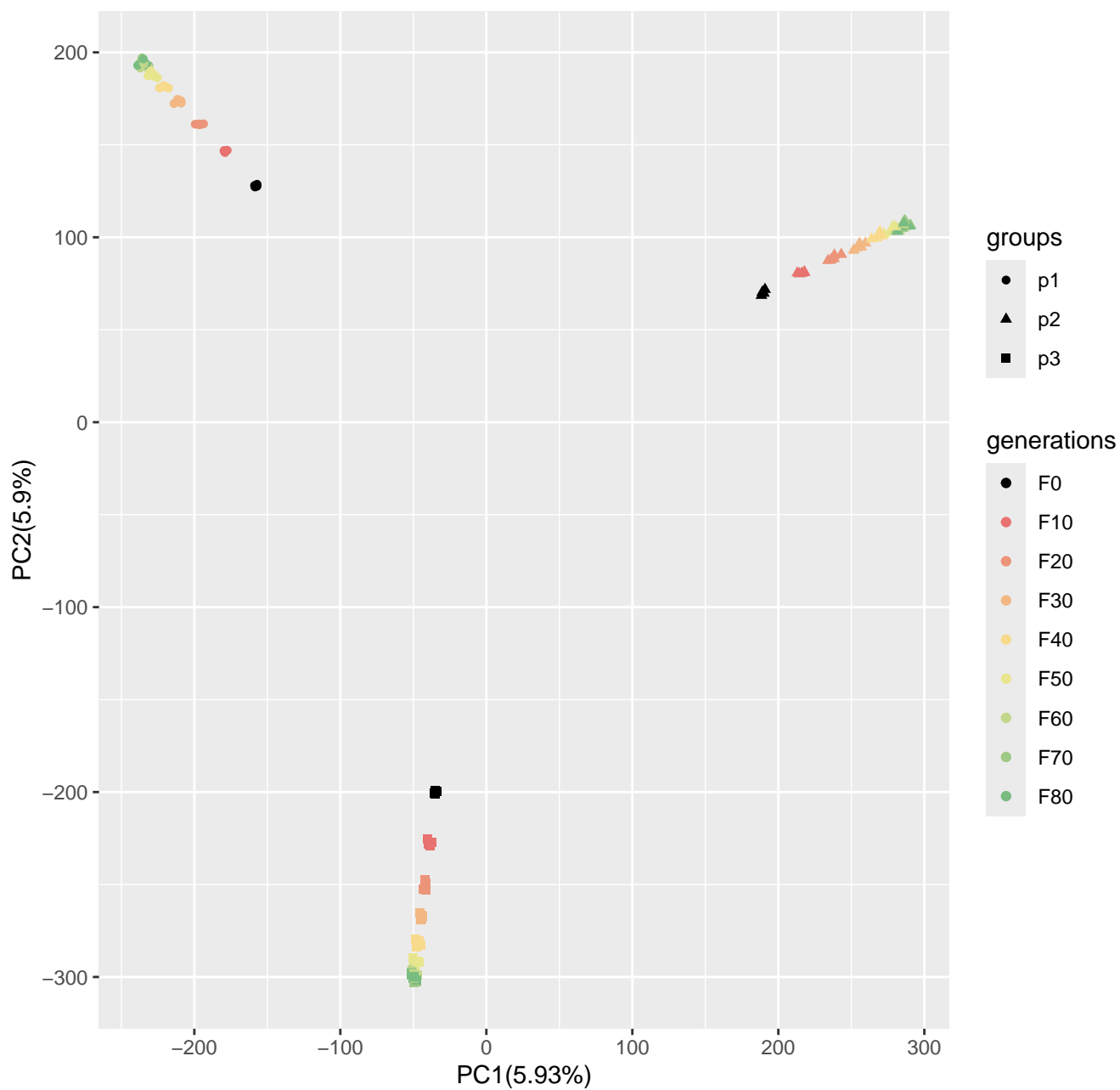
Run6_popsizel250_n400_10000loci_s10
