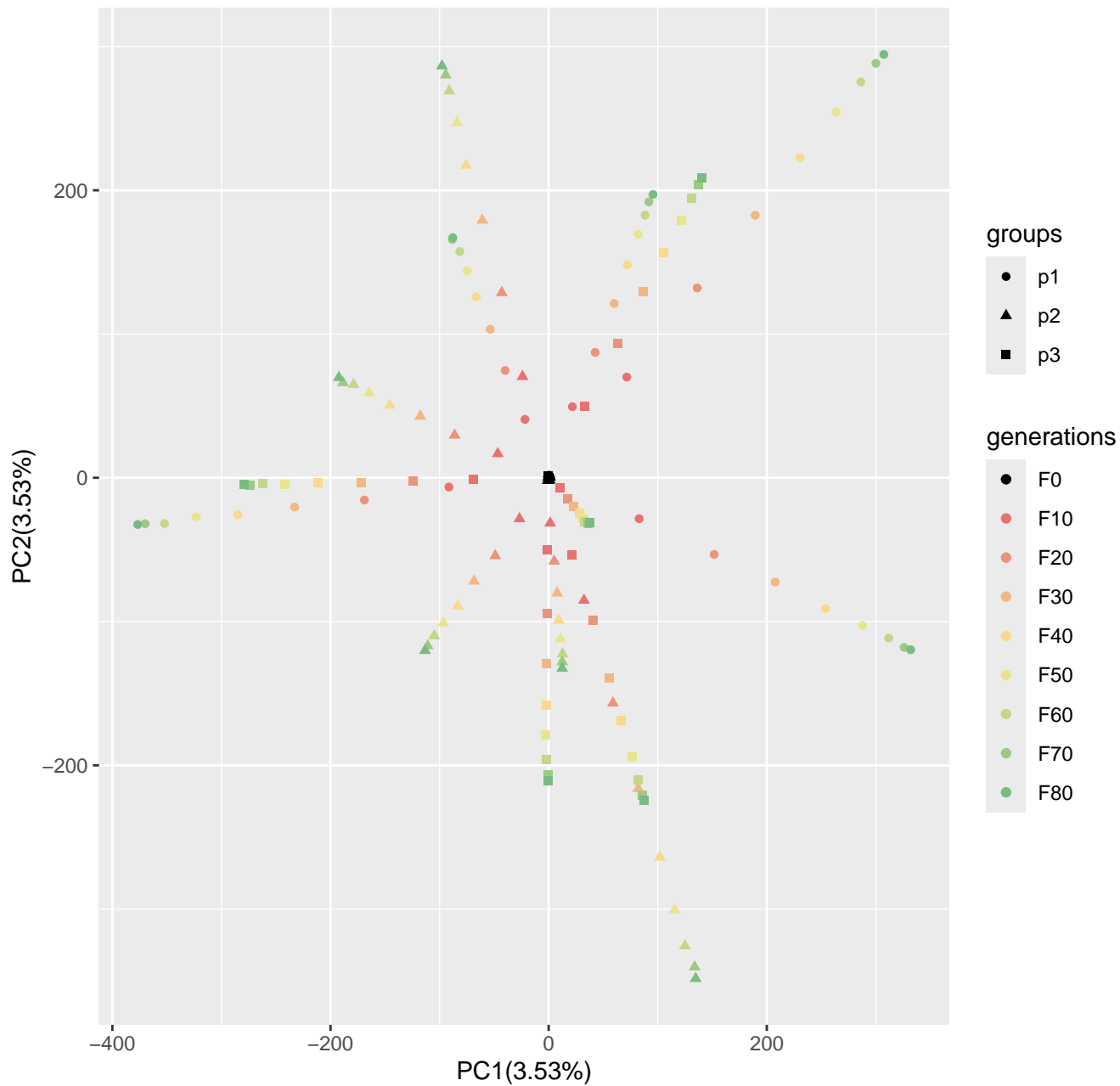
Run3_popsizel250_n400_5000loci_s10
