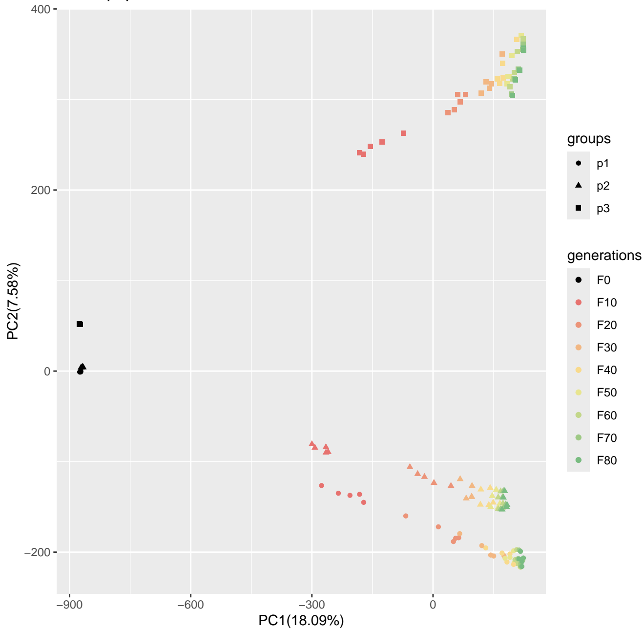
Run7_popsizel250_n400_100loci_s50
