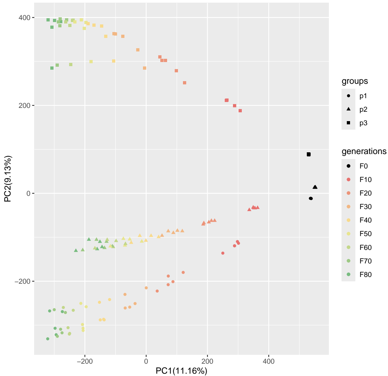
Run10_popsizel250_n400_1000loci_s50
