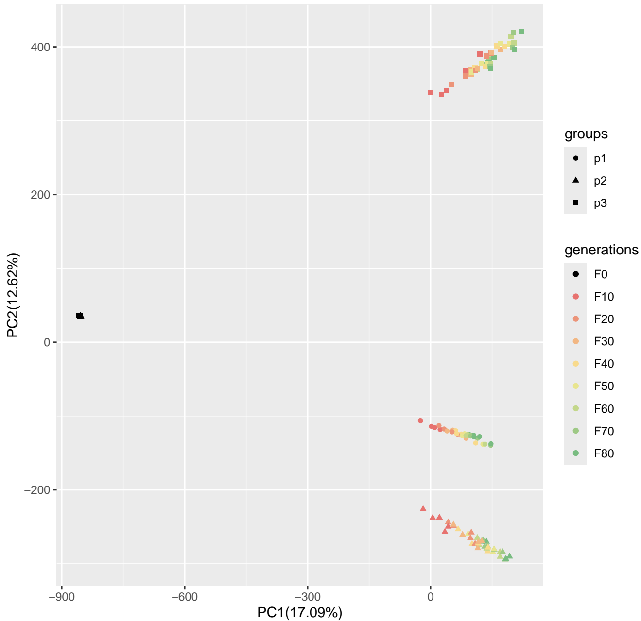
Run7_popsizel250_n400_10loci_s50
