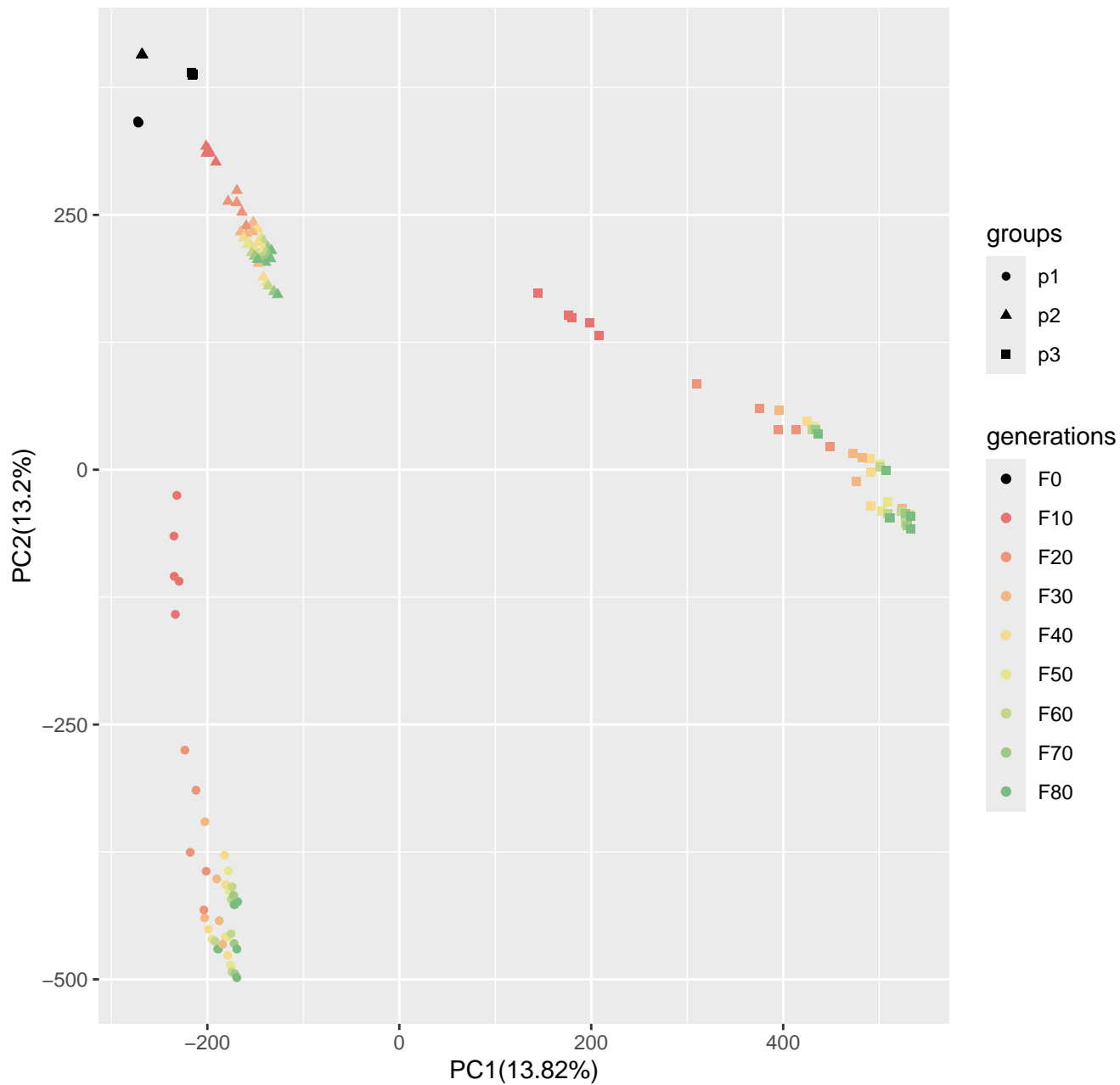
Run4_popsizel250_n400_10loci_s10
