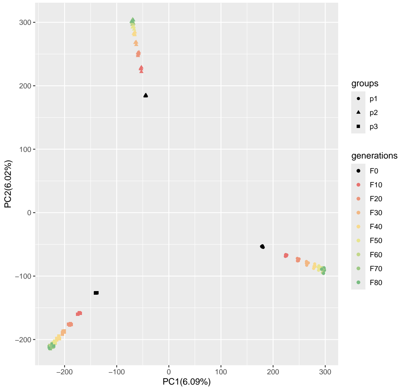
Run7_popsizel250_n400_100loci_s10
