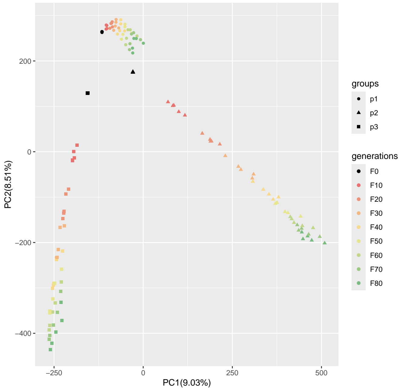
Run10_popsizel250_n400_100loci_s10
