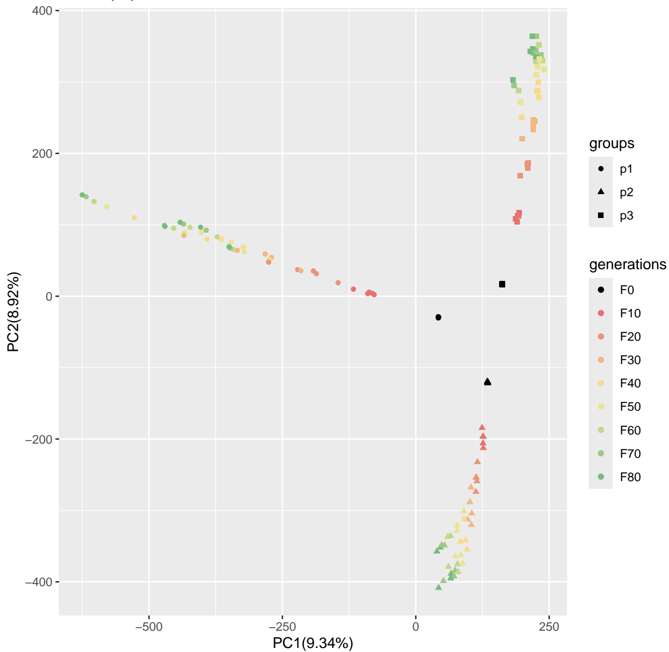
Run3_popsizel250_n400_100loci_s10
