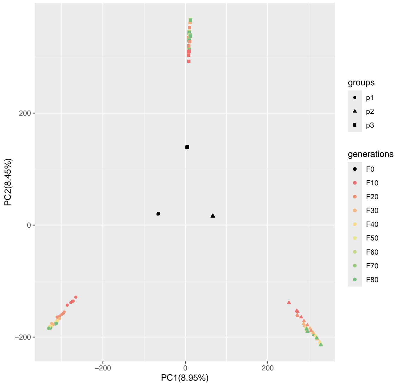
Run8_popsizel250_n400_100loci_s50
