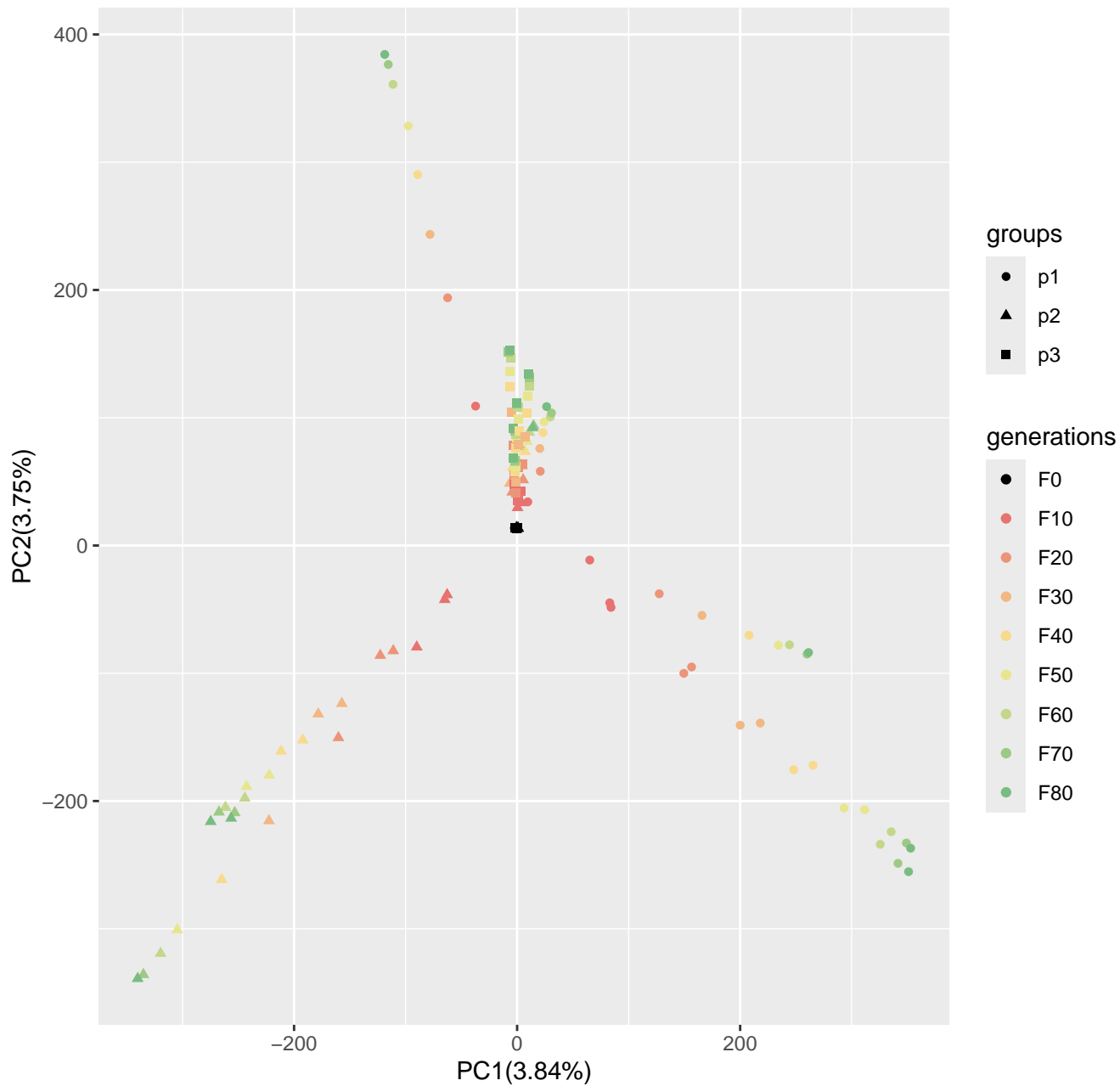
Run6_popsizel250_n400_10000loci_s10
