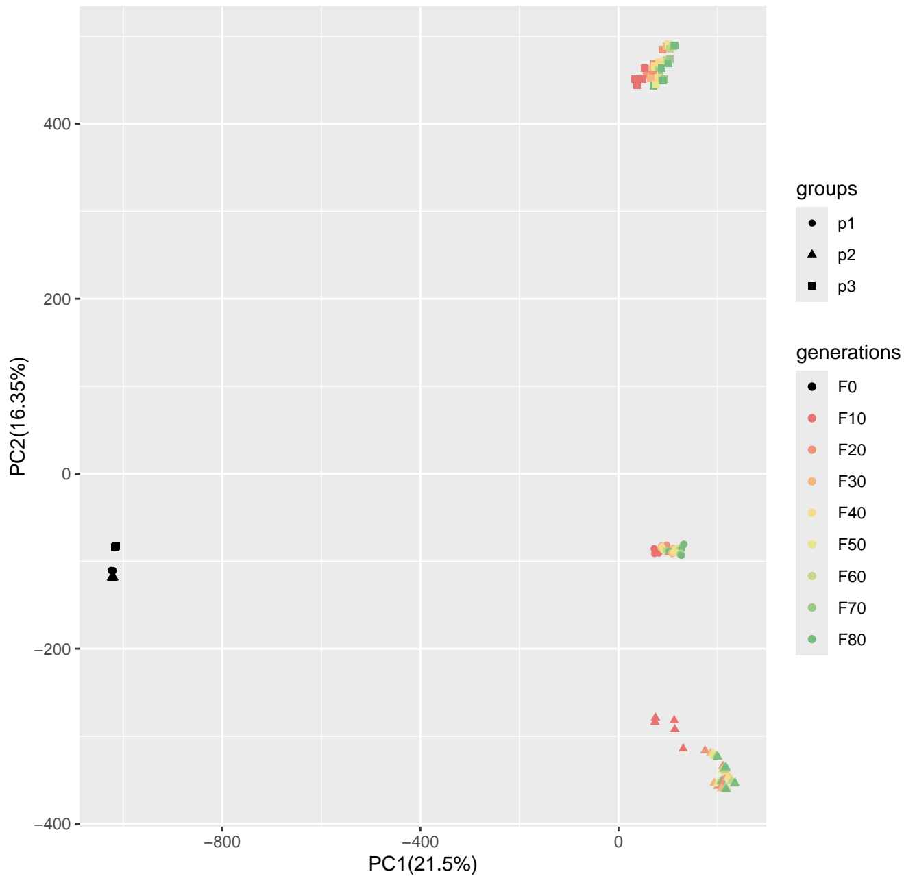
Run2_popsizel250_n400_10loci_s50
