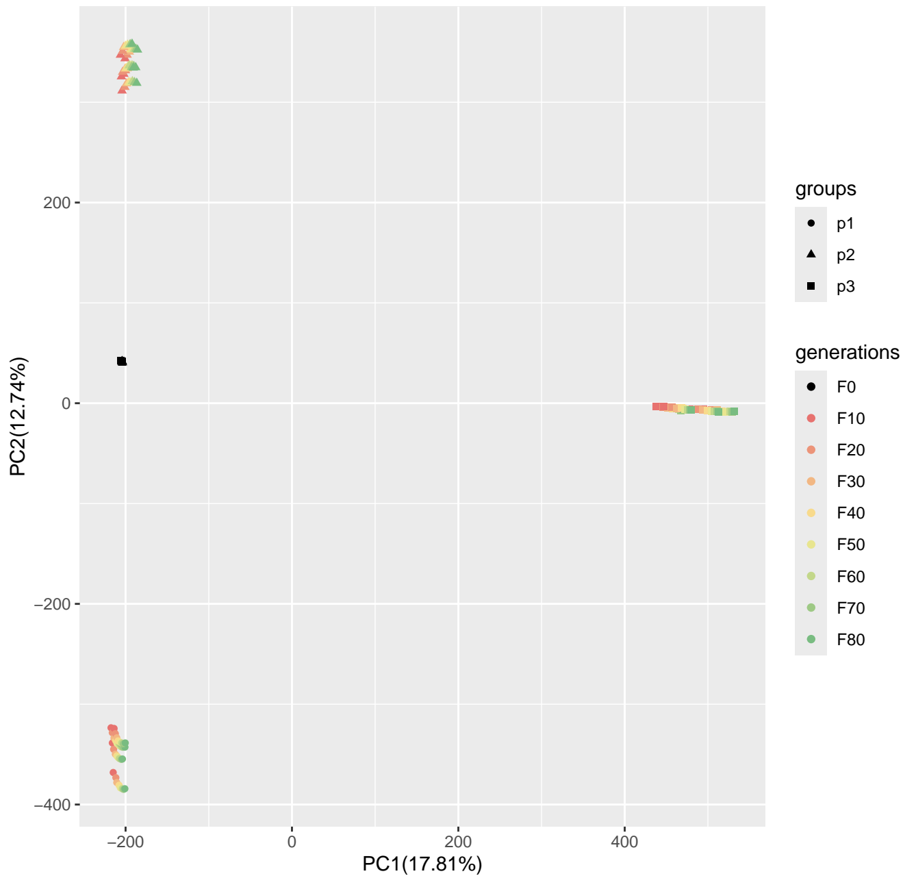
Run3_popsizel250_n400_10loci_s50
