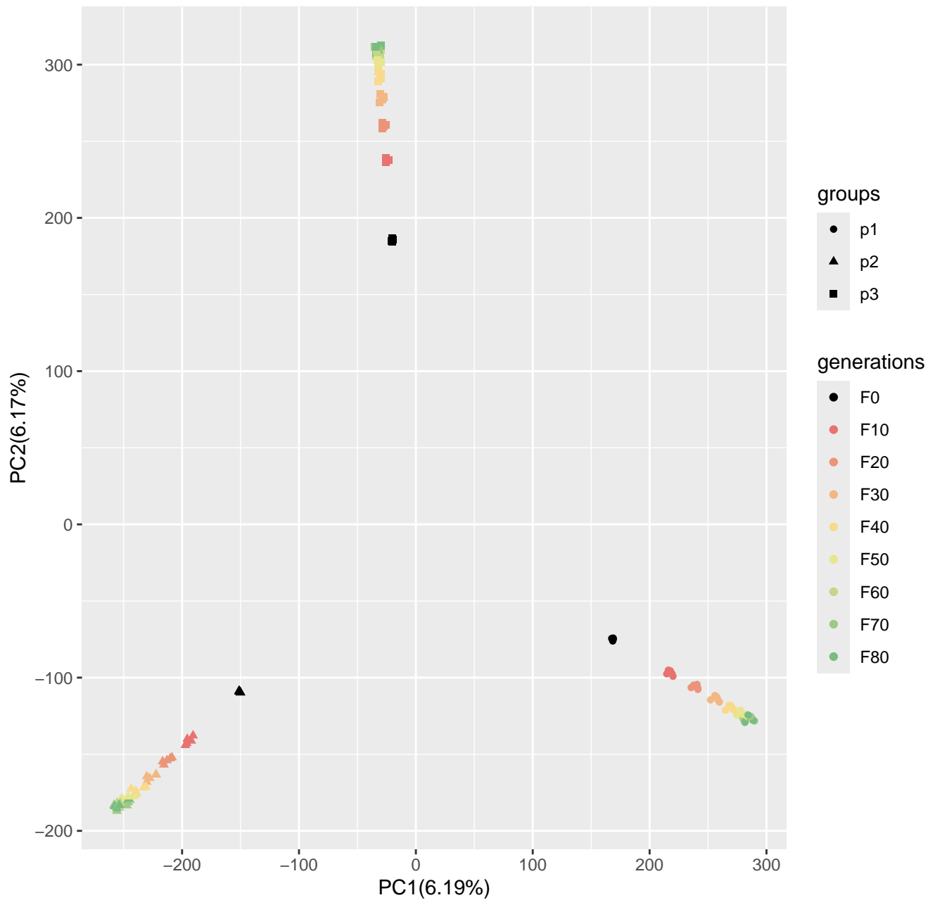
Run2_popsizel250_n400_100loci_s10
