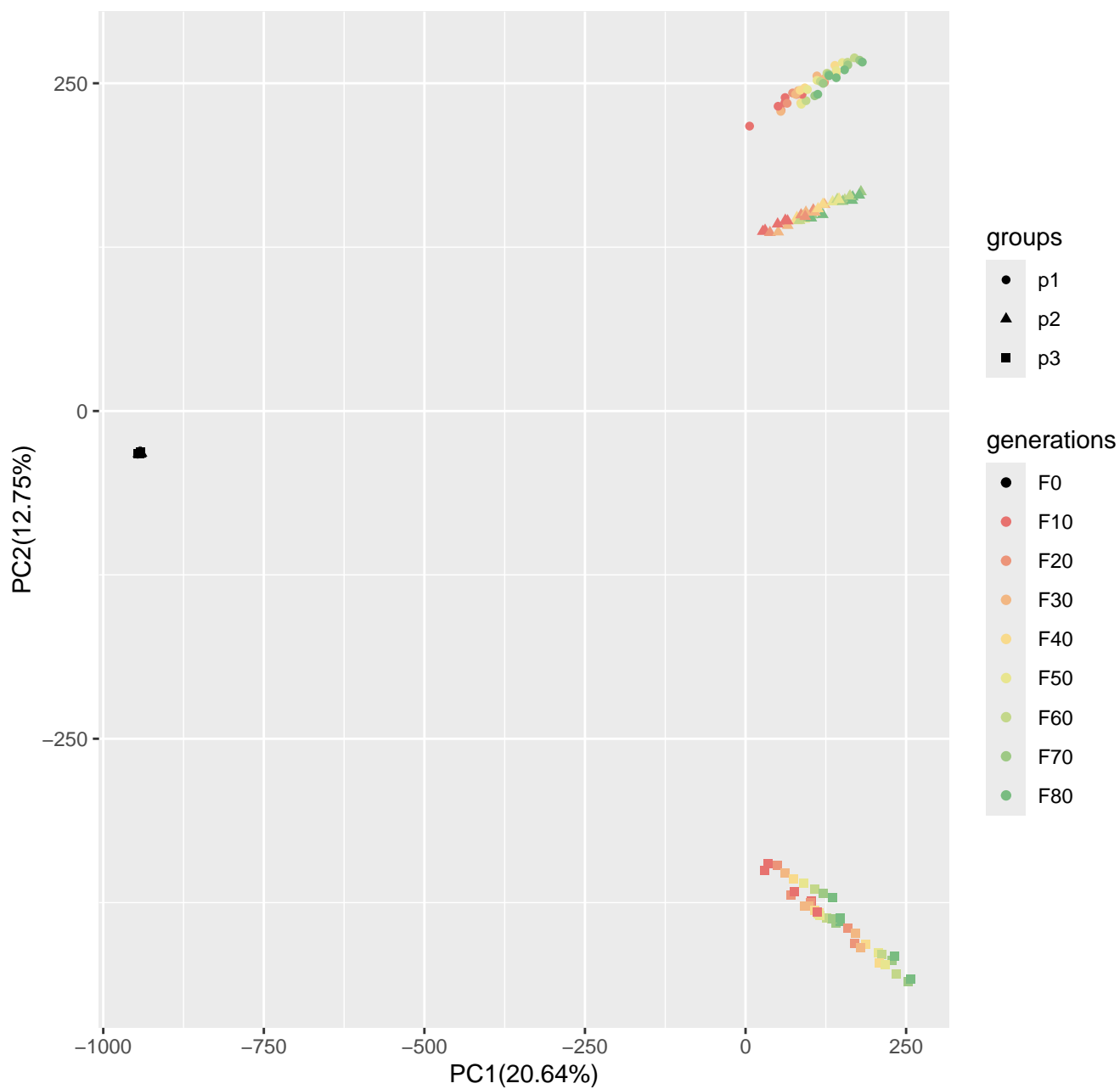
Run7_popsizel250_n400_10loci_s100
