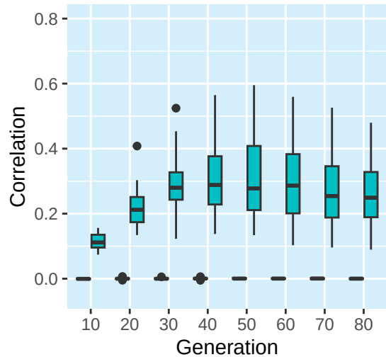
100loci_s10(sc=0.1)
