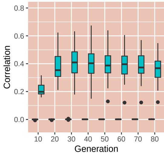
5000loci_s100(sc=0.02)
