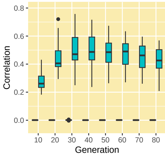
1000loci_s50(sc=0.05)
