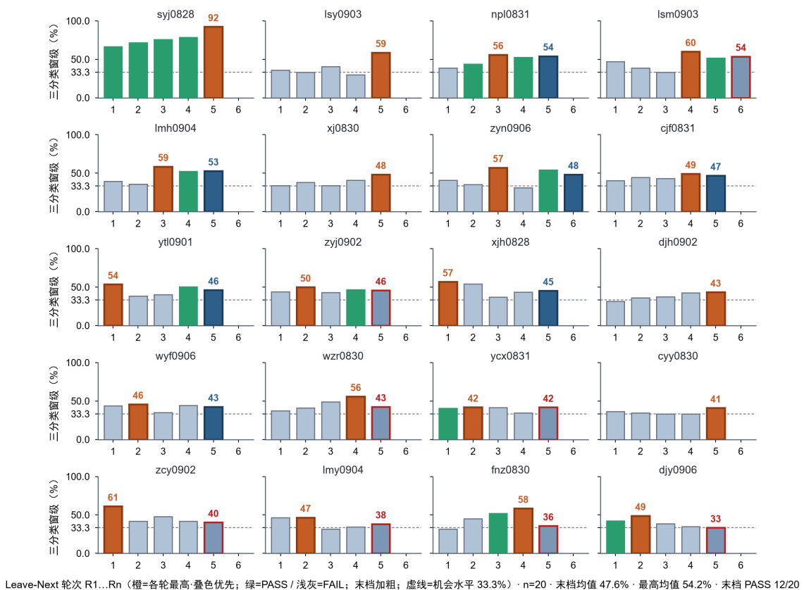
图 15 真人被试 Leave-Next 逐轮微调三分类窗级（小倍数柱状）。每面板一名被试，横轴为 Leave-Next 轮次 R1...Rn，纵轴为保留评测三分类窗级准确率（因果平滑，%）；橙色=该被试各轮最高（与 PASS 绿/末档主色重叠时优先用橙），绿=该轮门控 PASS，浅灰=FAIL，末档另加粗（非最高
