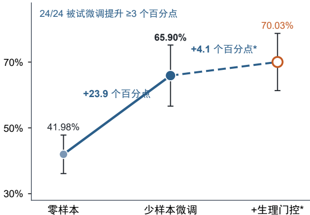
试次级三分类准确率
