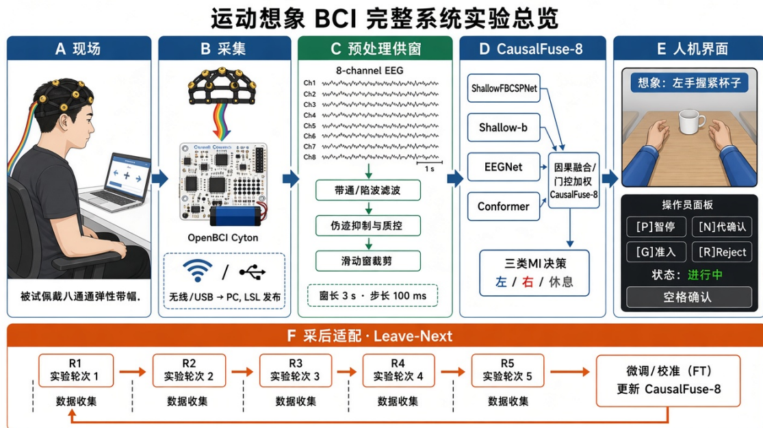
图 1 运动想象 BCI 完整系统实验总览。左起五栏为实时主链路（A 实验现场 → B 信号采集 → C 预处理与供窗 → D CausalFuse-8 解码 → E 人机交互界面），底栏 F 为实时路径外的采后适配（落盘 → Leave-Next 微调 → 门控晋升）。图面为按实物硬件与界面绘制的示意图（不嵌实拍缩略图）；操作台为示意，实拍波形/概率界面见演示视频；硬件特写、佩戴与游戏界面局部见图 2 - 图 4。
