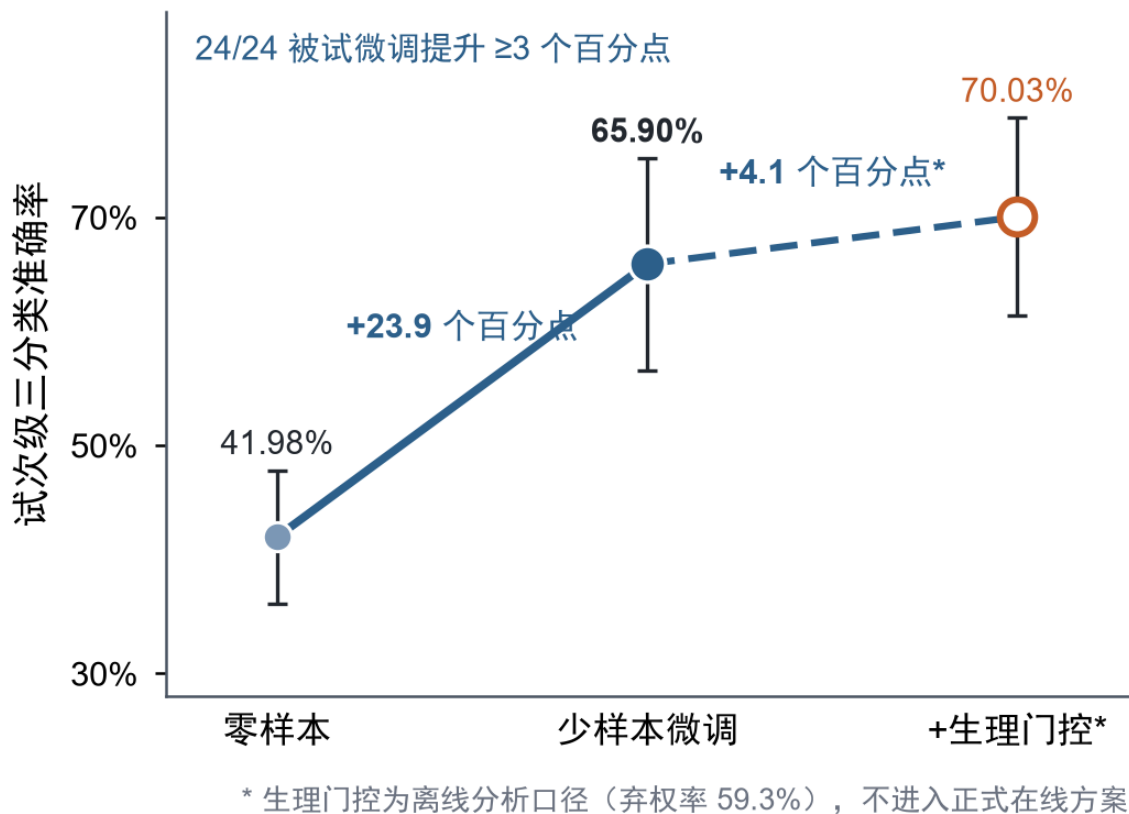
图 12 Stieger 跨库伪在线（24 人子集）。前半会话训练、后半评测。生理门控为离线旁路（弃权 59.3%），不进入正式在线方案。
