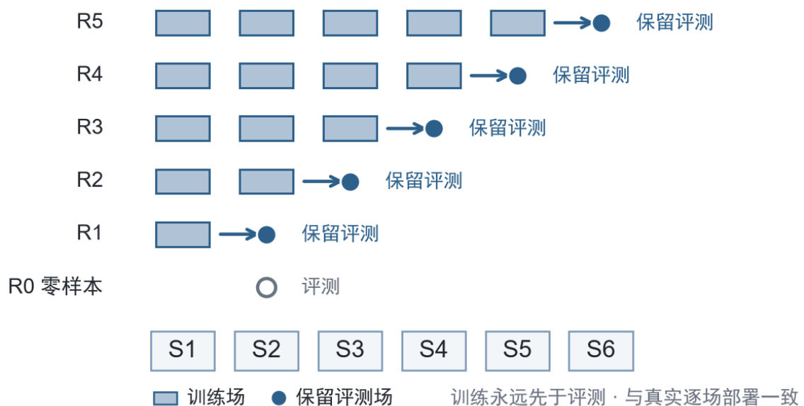
图 13 Leave-Next（逐场次采后微调）方案示意。第 r 轮以已完成场次为训练集、紧邻下一场为保留评测；R0（第 0 轮）为零样本底座直接推断。训练永远先于评测，与真实部署的逐场晋升一致，
