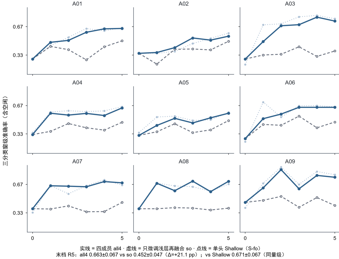
图 14 BCI2a (A01 - A09) Leave-Next 仿真的逐被试适配轨迹（源域回放 10%）。实线 = 四成员全量微调 (CausalFuse-8FT)；虚线 = 仅微调浅层成员、其余成员冻结后再融合；点线 = 浅层单模型直接微调基线。末轮（第 6 轮）：四成员全量微调 66.30\% \pm 6.70\% ，对仅微调浅层单成员 45.20\% \pm 4.70\% ( \Delta = +21.1 个百分点，配对显著)；浅层单模型基线 67.10\% \pm 6.70\% （与四成员同量级）。曲线随轮次上升支撑 Leave-Next 方案；四成员全量微调相对仅微调浅层单成员的大幅提升支撑全成员微调范围。
