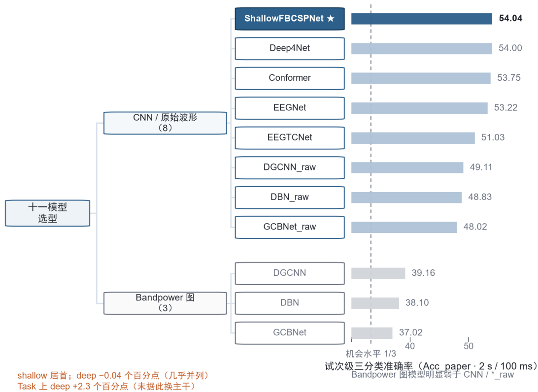
图 9 OpenBMI 统一评测方案下十一模型选型树 (2 s / 100 ms • Acc_paper)。左为分层树：CNN/原始波形 (8) 与 Bandpower 图模型 (3)；右为试次级三分类准确率条 (数字标在条外，避免与标记重叠)。深蓝条 + ★ = 采纳主干 ShallowFBCSPNet (54.04%)；Deep4Net (54.00%) 几乎并列。虚线为机会水平 1/3。数据锁自 5060 正式汇总表 (与正文表前四行一致)。
