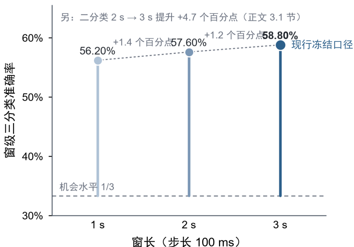
图 8 窗长消融（OpenBMI，统一评测方案）。窗级三分类准确率随窗长变化，3 s 窗最优并冻结为现行口径（步长 100 ms）；虚线为机会水平。点估计，折间波动见正文；纵轴自 0.30 起。注意：十一模型对比在另线 2 s 口径下完成，与本图窗长消融正交。
