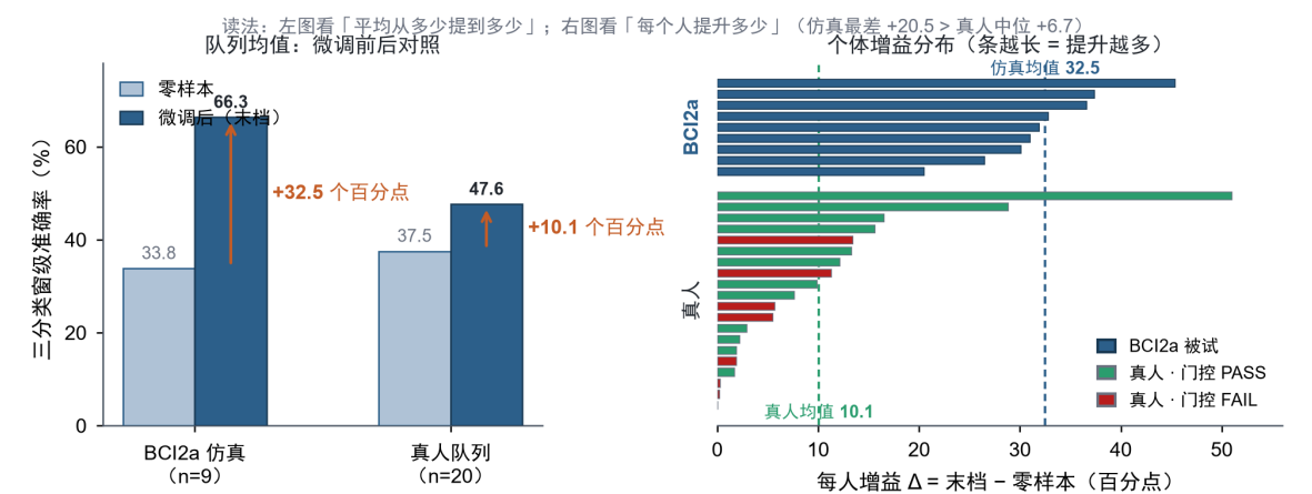
图 16 BCI2a 仿真与真人队列的适配增益对照（n=9 对 n=20，三分类窗级，末档口径）。左为队列均值抬升（仿真 +32.5、真人 +10.1 个百分点）；右为每人增益 \Delta （蓝=BCI2a，绿/红=真人 PASS/FAIL）。仿真最差个体（+20.5）仍高于真人中位数（+6.7）。
