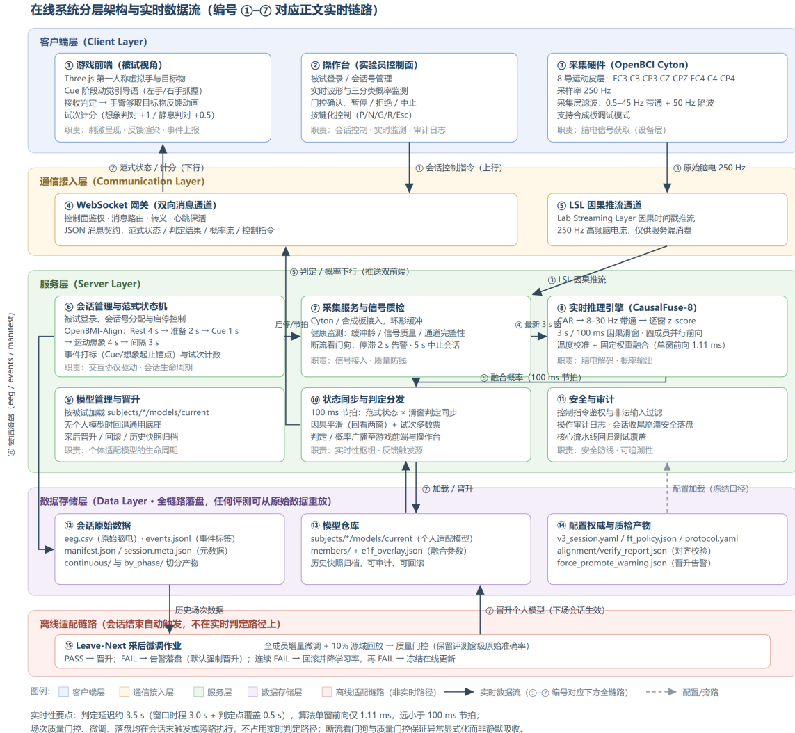
图 5 在线系统分层架构与实时数据流。客户端层（游戏前端/操作台/采集硬件）经 WebSocket 网关与 LSL 通道接入服务层；服务层以 100 ms 节拍完成“供窗—推理—分发”闭环；会话数据全量落盘；操作台启动采后微调后，晋升的个人模型可在下一会话加载。编号 ① - ⑦ 对应正文实时链路；硬件实物连接见图 2。
