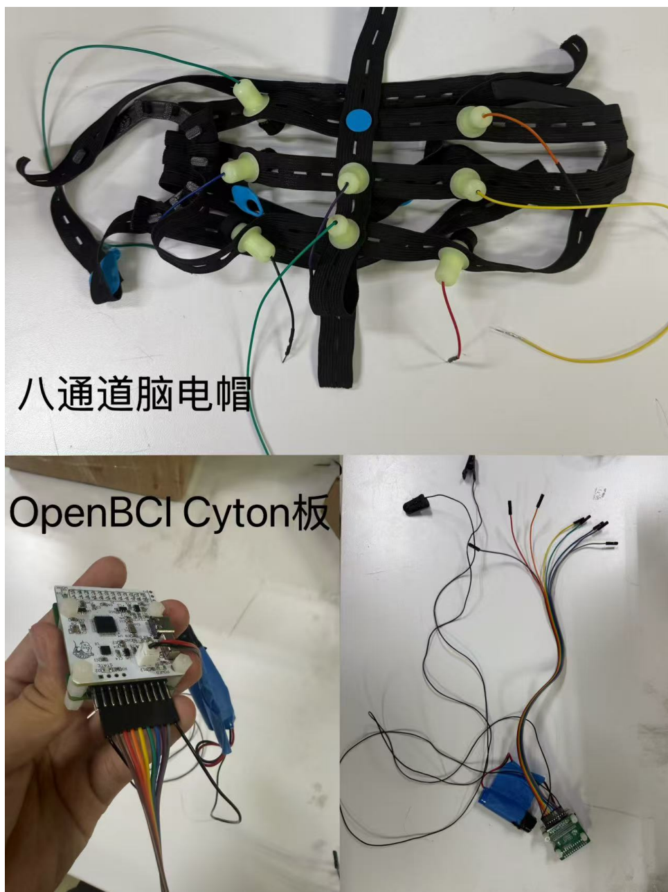
图 2 系统采集硬件实物。上：八通道干电极脑电帽（10 - 20 系统运动皮层位点）；下左：手持 OpenBCI Cyton 板；下右：Cyton 与电池组及跳线组装。信号链路为电极帽 → Cyton（250 Hz 采样；板载带通/陷波关闭，输出原始采样）→ 采集主机（BrainFlow / LSL）→ WebSocket 网关 → 游戏前端/操作台；频带滤波在主机软件预处理完成（见 2.3 节），分层软件架构见图 5。
