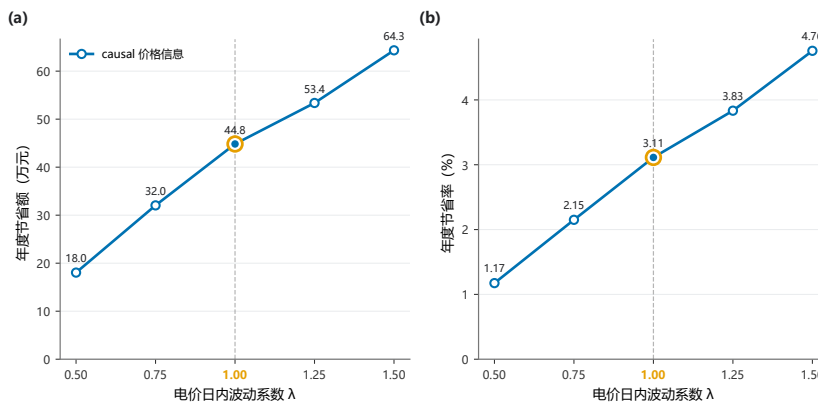
图 7 不同电价波动情形下滚动策略的节约效果
