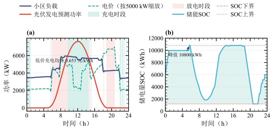
图 2 问题一供需曲线与储能调控轨迹
