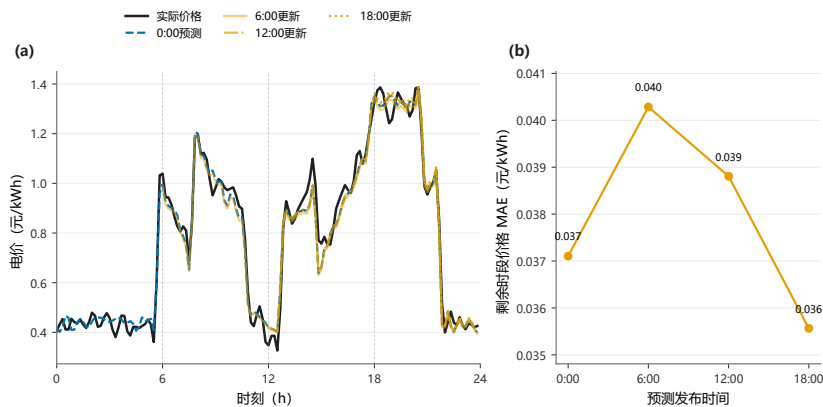
图 6 实际电价与各发布时间的预测对比
