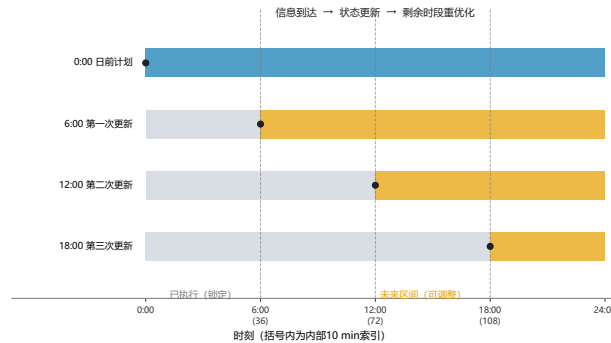
图 5 0 时制定原计划，6、12、18 时用新预报和实测储电量优化当日剩余时段；每段采用最近一次可用计划。
