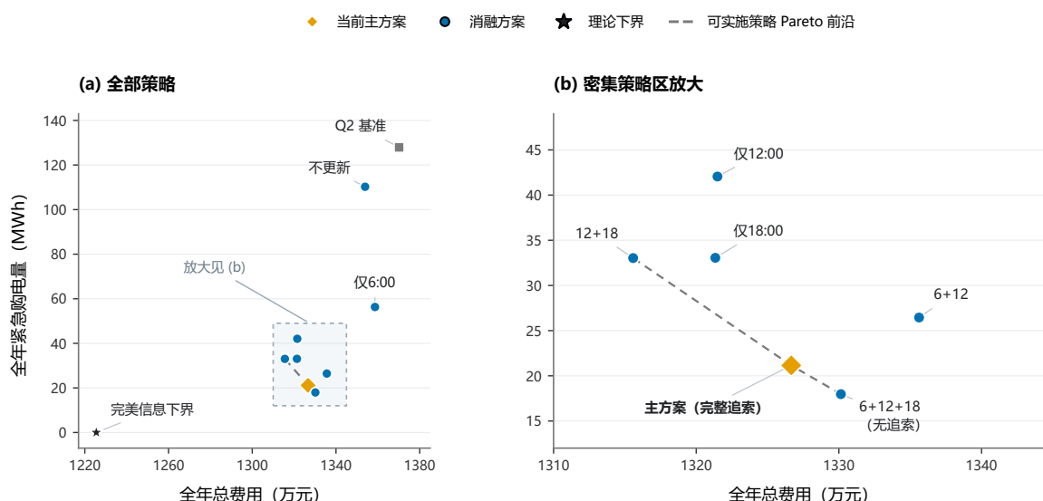
图 10 滚动方案的费用与紧急购电量比较
