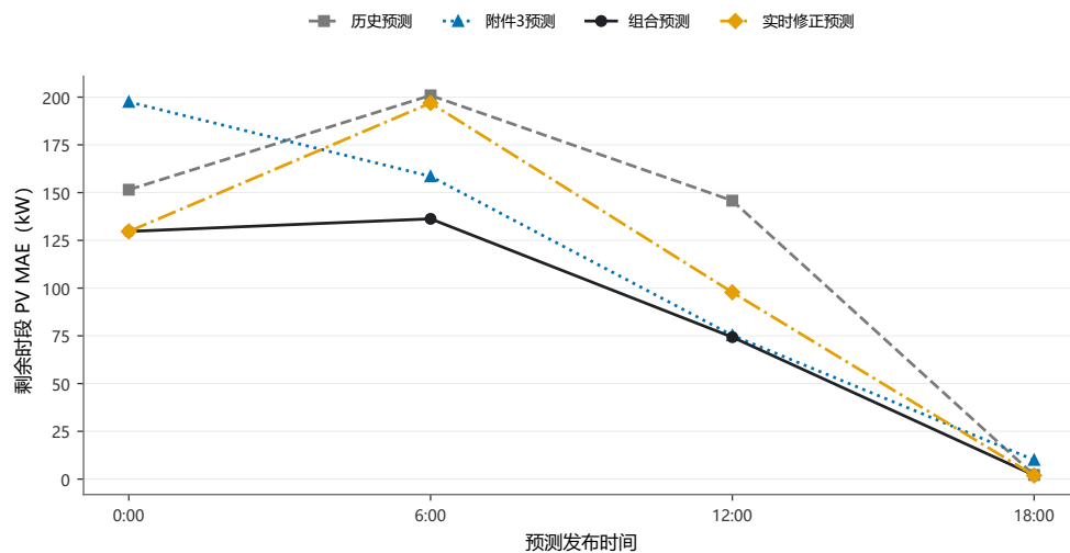
图 9 各发布时间的的光伏预测误差
