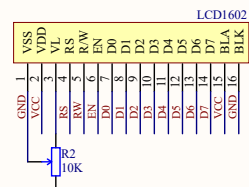
LCD1602液晶显示电路
