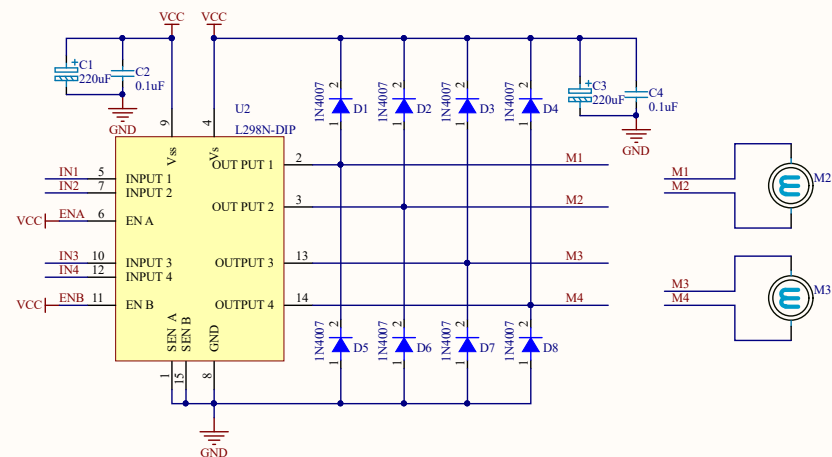
L298N电机驱动芯片电路
