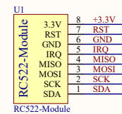
RC522模块电路
