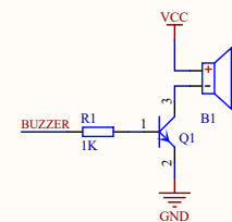
蜂鸣器电路
