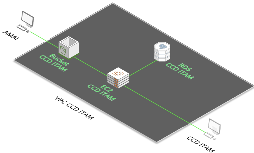
Figura 3.3. Diagrama de servicios de AWS utilizados por el CCD del ITAM para el proyecto
