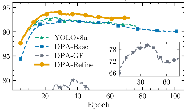
mAP@0.5 (%)
