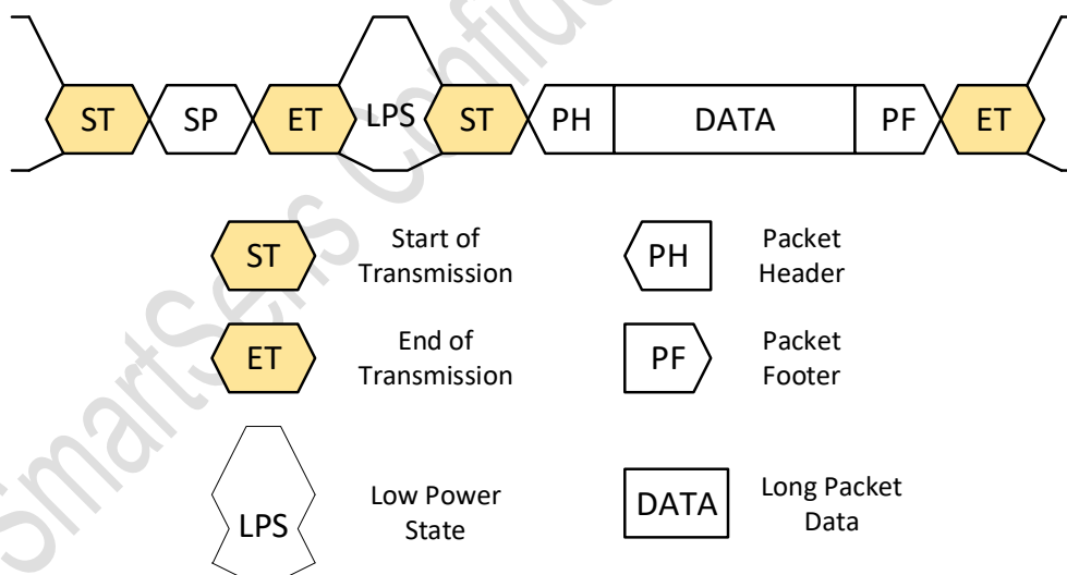
图 1-12 MIPI 底层数据包示意图
