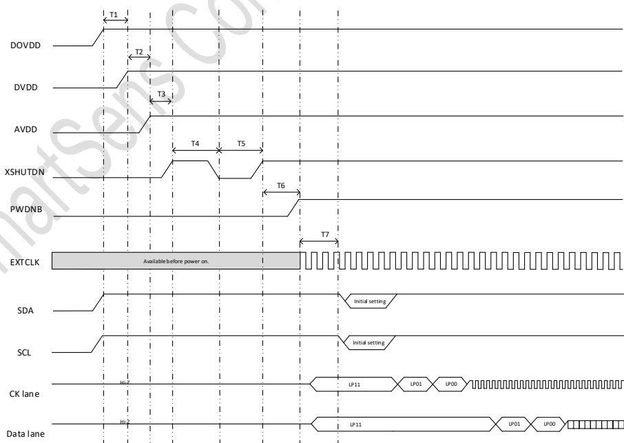
图 1-7 上电时序图(COB)
