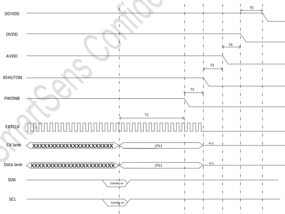
图 1-9 下电时序图(COB)
