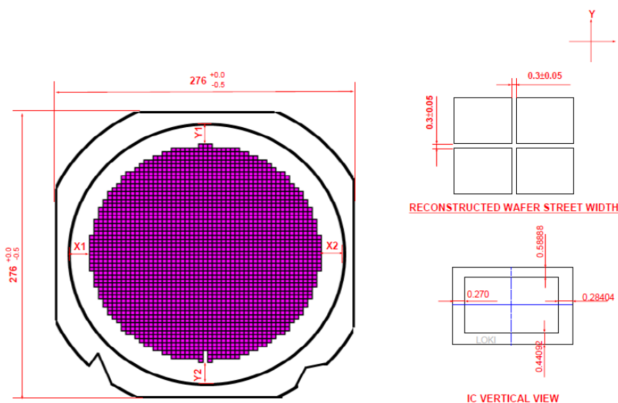
图 5-2 RW 尺寸示意图
