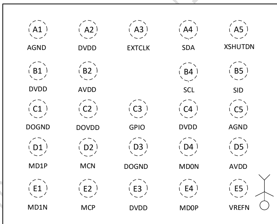
图 1-5 封装引脚图(CSP)
