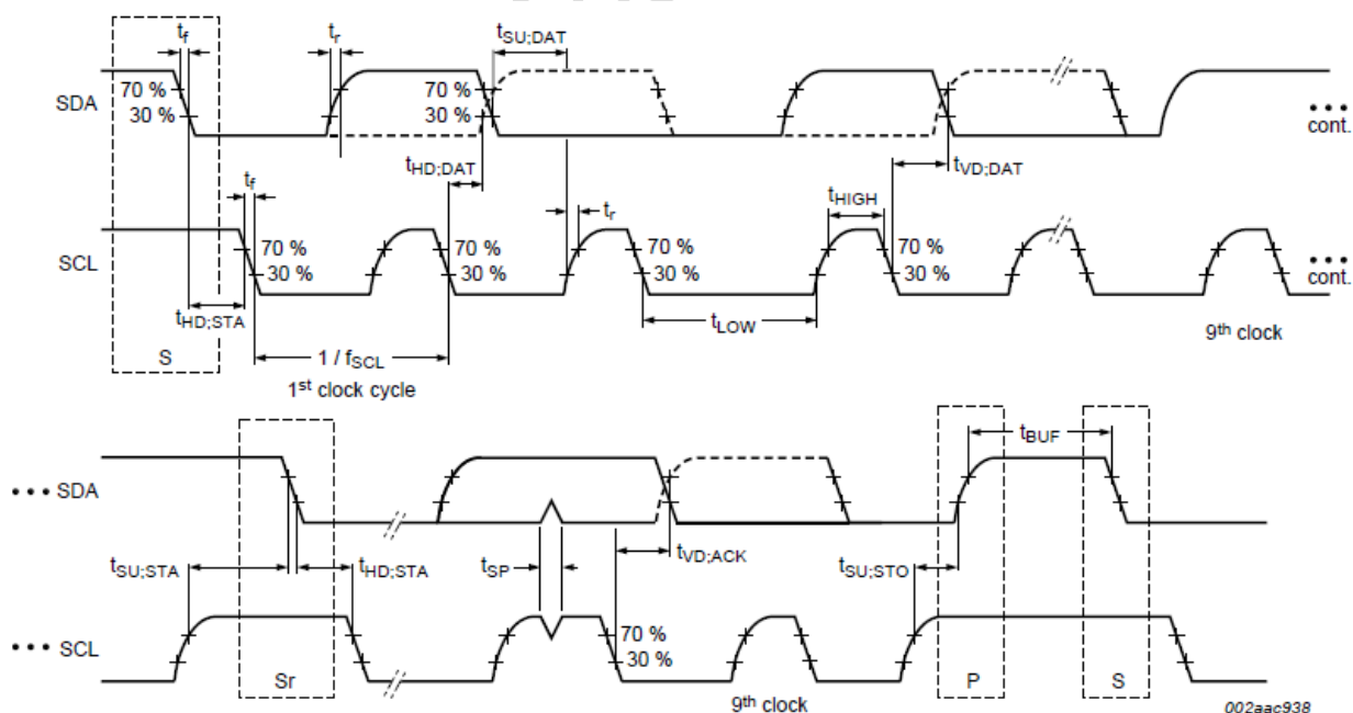
图 1-10 I2C 接口时序
