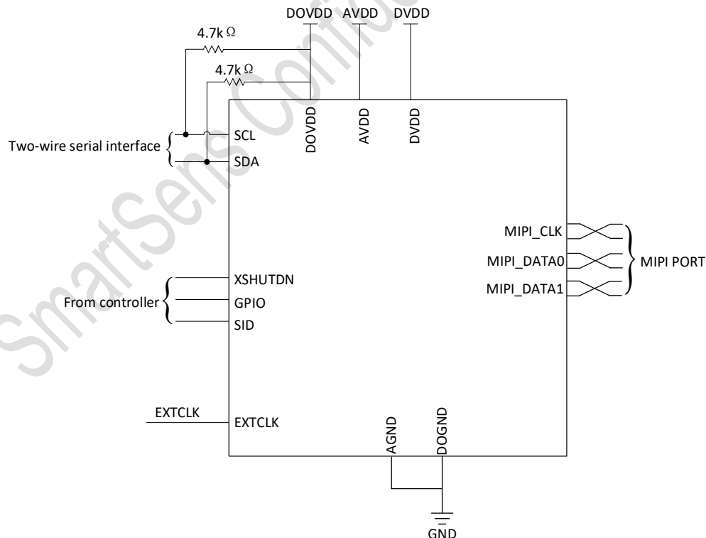
图 1-3 典型应用示意图(CSP)
