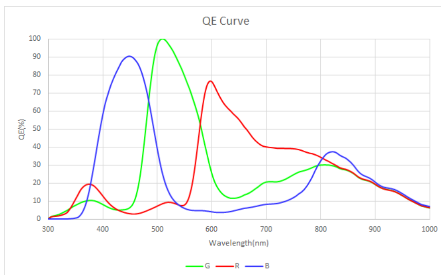
图 4-1 QE 曲线
