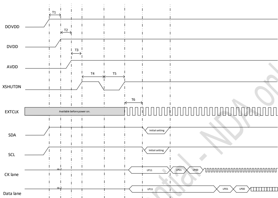
图 1-6 上电时序图(CSP)
