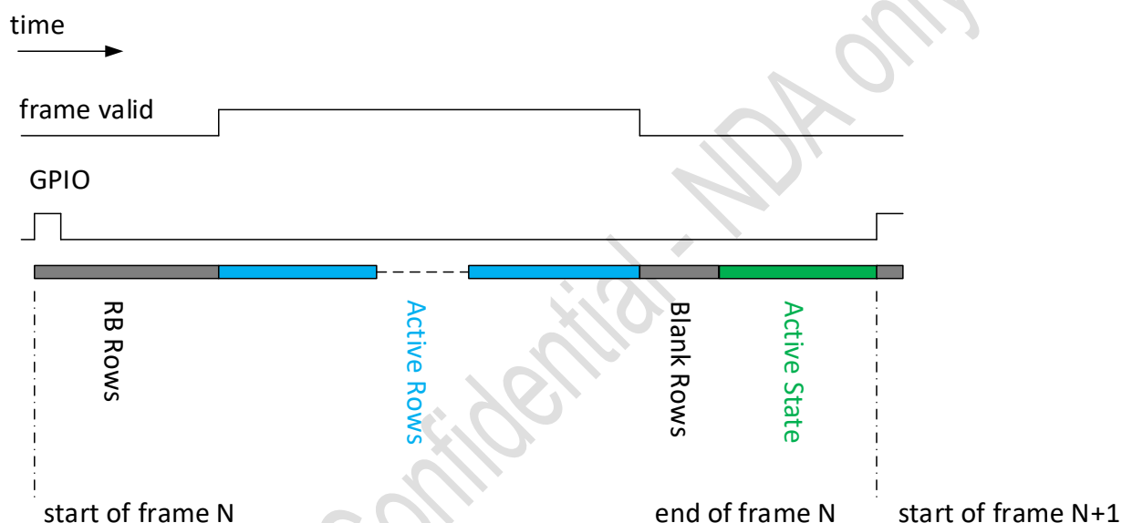
图 2-1 Slave Mode 时序图
