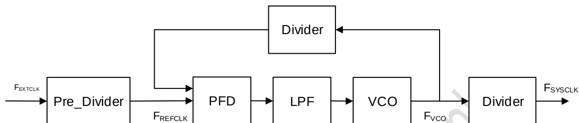
图 1-16 PLL 控制示意图
