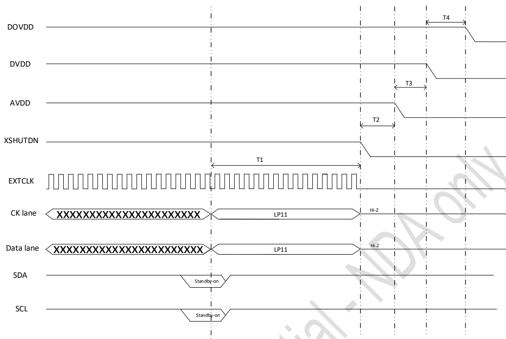
图 1-8 下电时序图(CSP)
