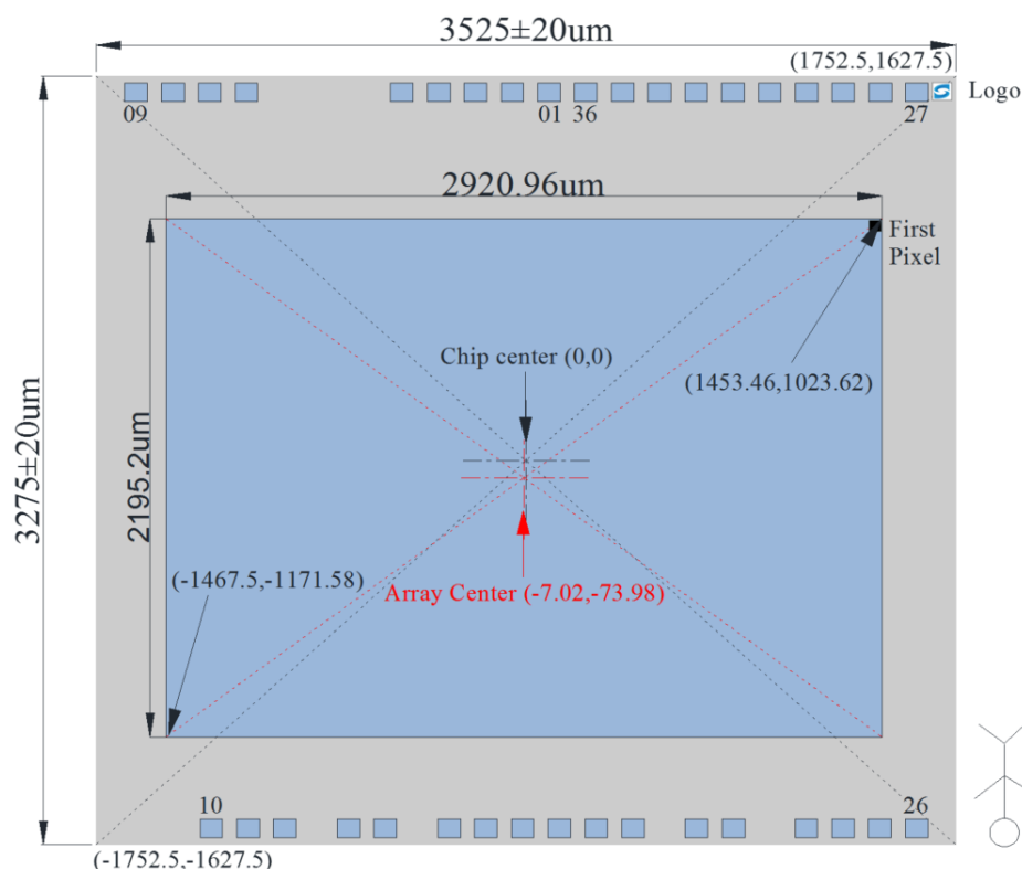
图 5-3 引脚图
