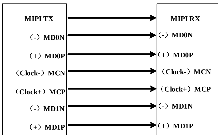
图 1-11 MIPI 接口示意图
