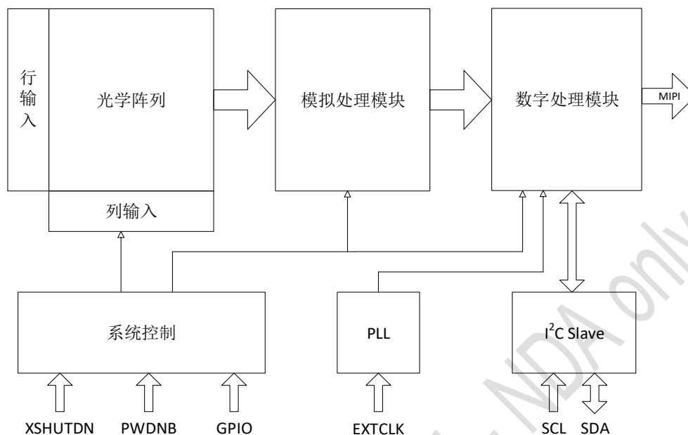
图 1-2 结构图(COB)
