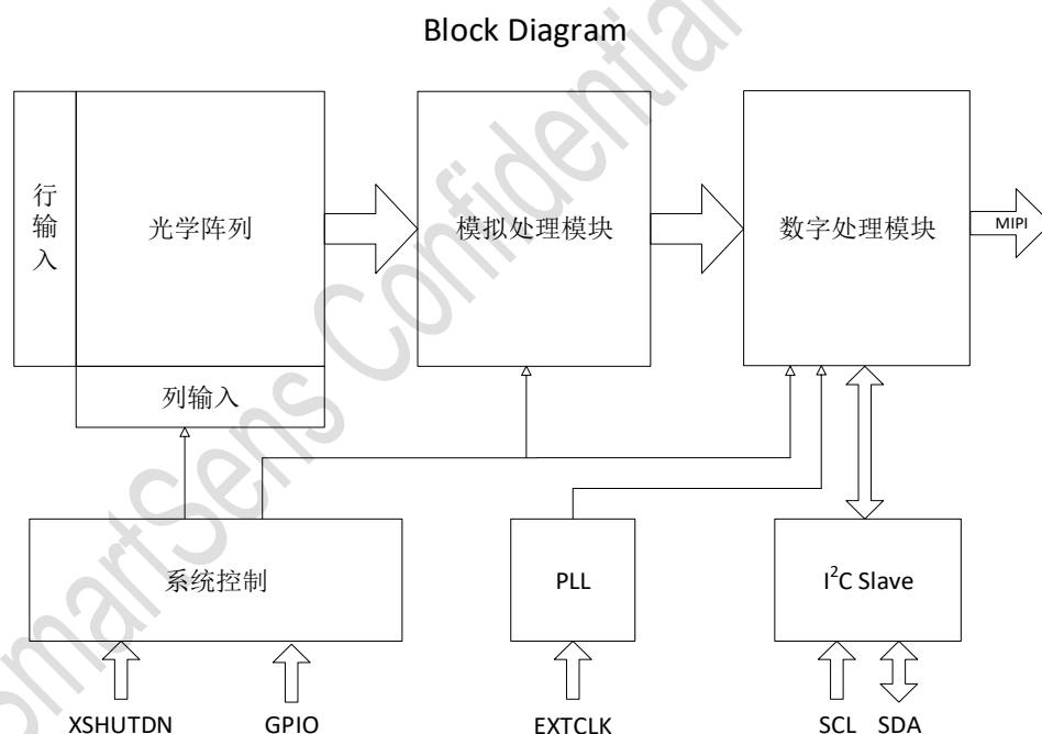
图 1-1 结构图(CSP)
