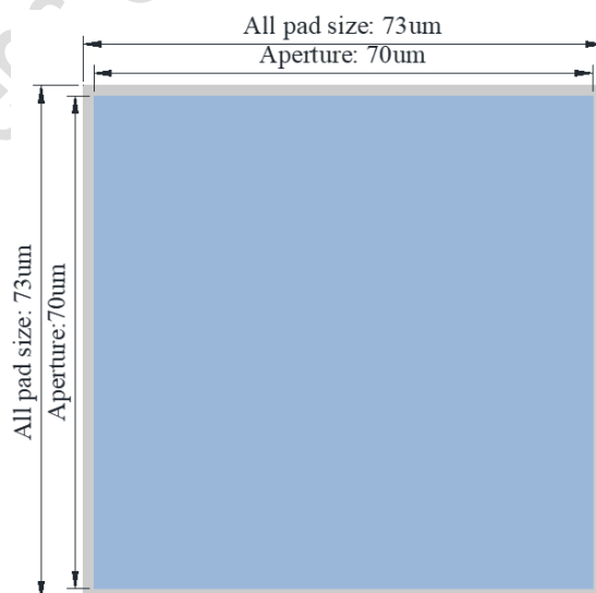
图 5-4 Pad 示意图
