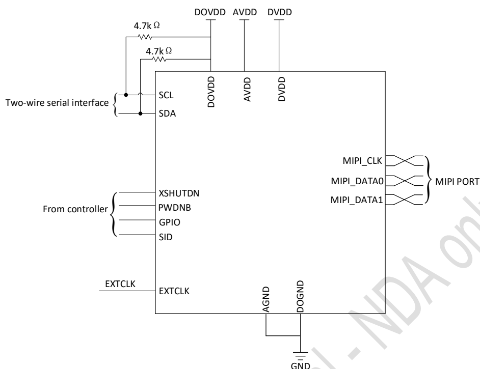
图 1-4 典型应用示意图(COB)
