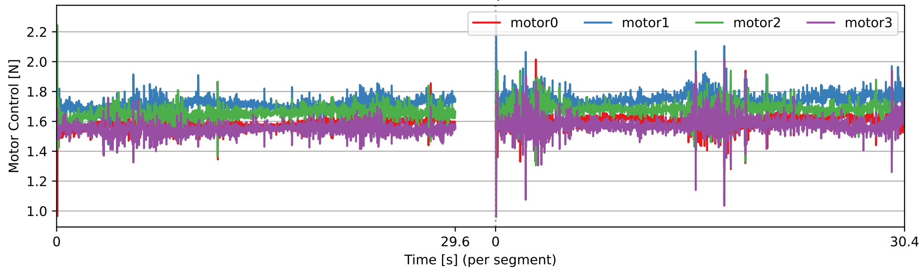
Motor Inputs
