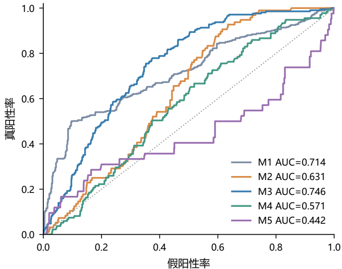
a 一对其余类别ROC
