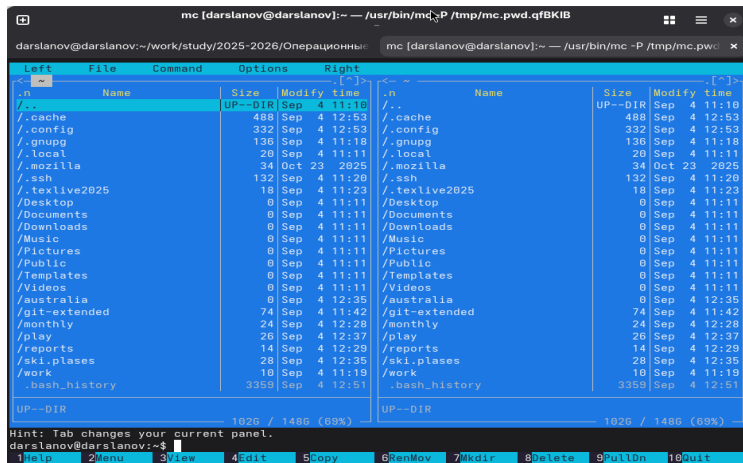
Рисунок 1: Запуск mc
