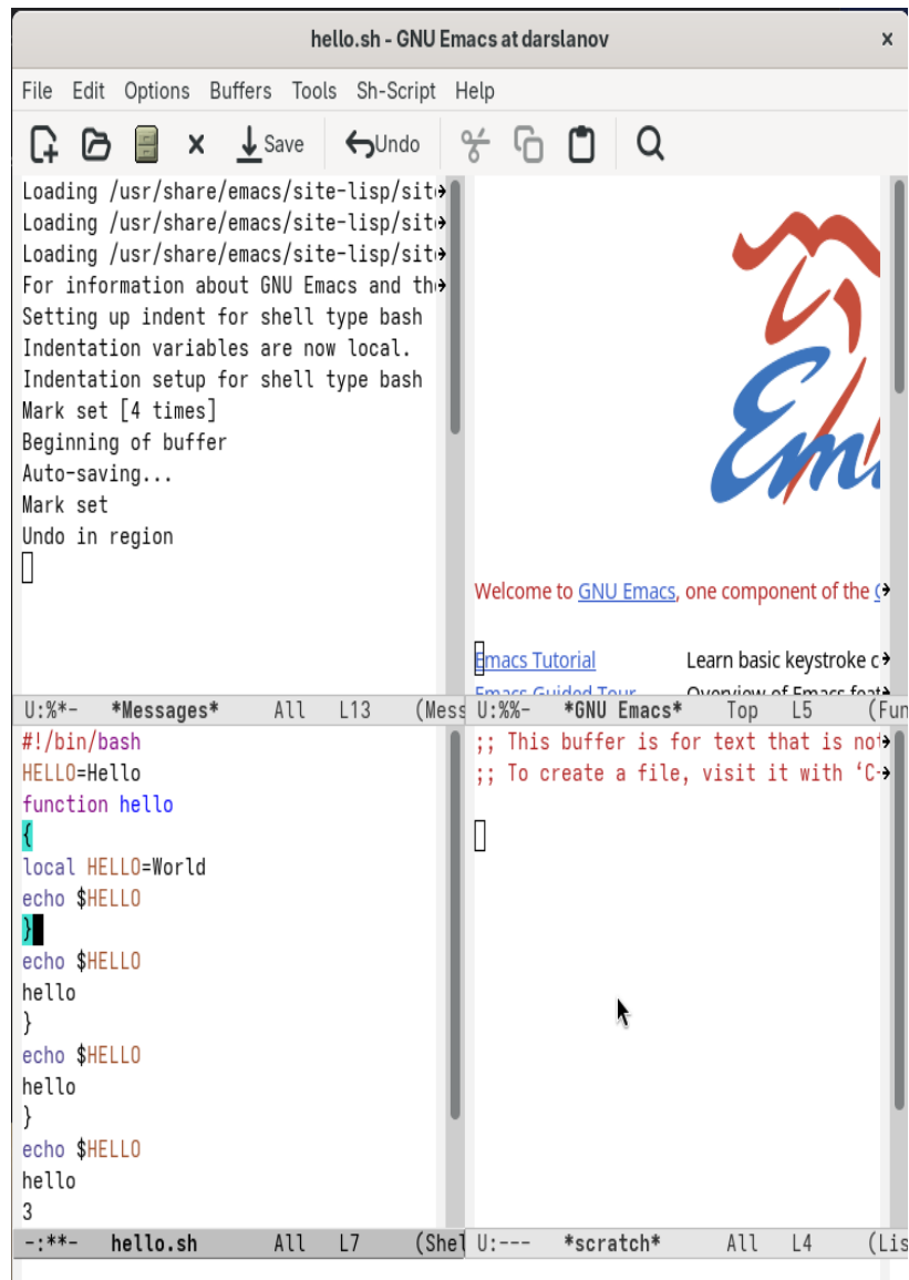
Рисунок 2.11: Четыре буфера
