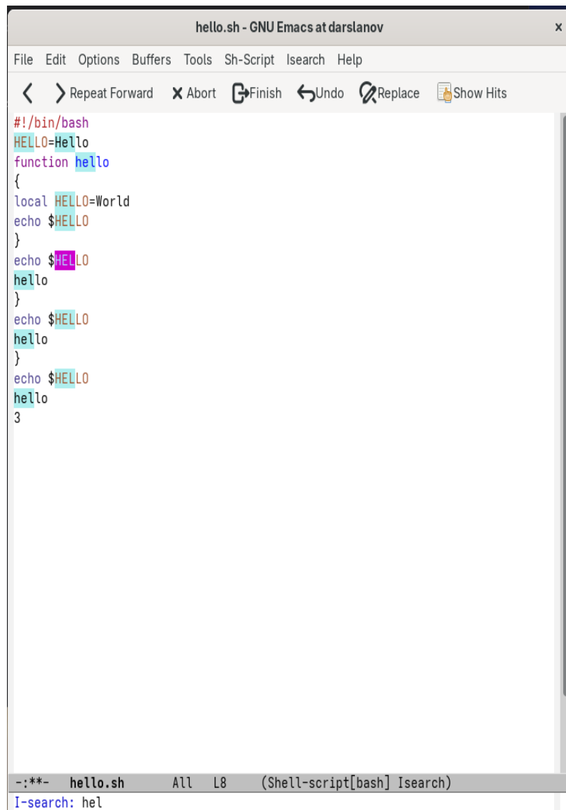
Рисунок 2.12: Режим поиска
