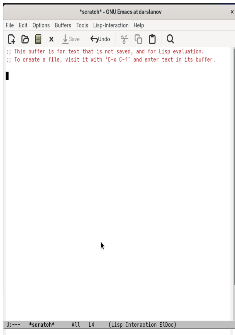
Рисунок 2.9: Закроем буфер
