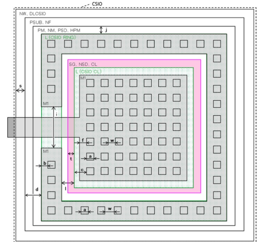
図 I-6-11. CSIOデザインルール
