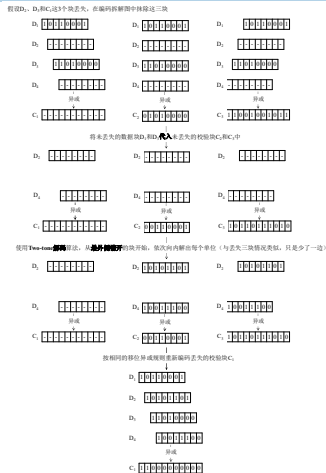
图 5: 丢失 2 数据块 1 校验块解码
