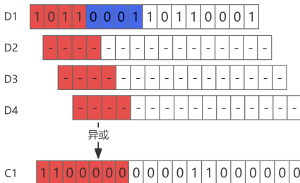
图 8: Cache-Friendly Window 效果演示
