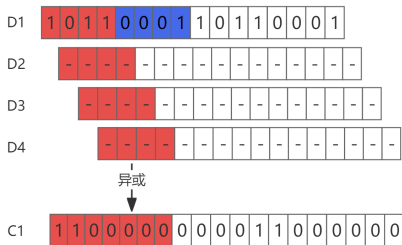
图 8: Cache-Friendly Window 效果演示
