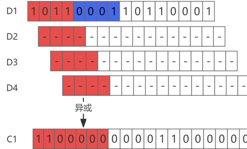
图 3-8 Cache-Friendly Window 效果演示
