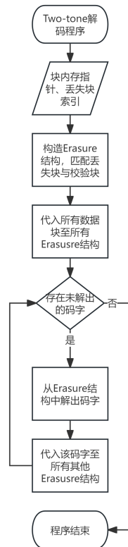
图 3-7 Erasure-Parity Mapping 统一解码实现流程
