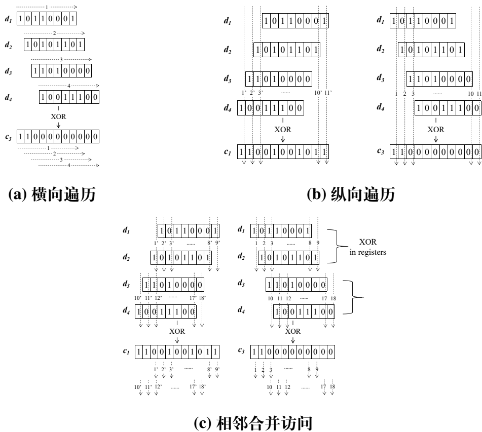
图 2-8 Two-tone 编码的访问模式对比：(a) 横向遍历，数据局部性好但校验写入分散；(b) 纵向遍历，校验写入集中但重复读取数据；(c) 相邻合并访问，相邻数据块窗口先在 SIMD 寄存器内异或合并，再以一次连续存储写回各校验块窗口
