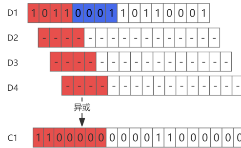
图 3-8 Cache-Friendly Window 效果演示
