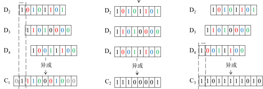
图 3-4 Two-tone 码丢失 3 个数据块的解码举例
