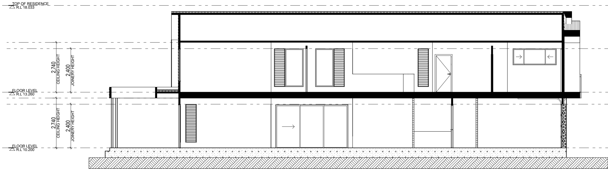
SECTION A-A
