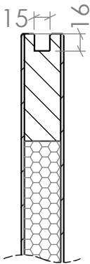
SEZIONE B-B ( teste ) SCALA 1 : 5
