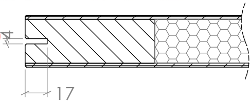
SEZIONE A-A ( lati lunghi ) SCALA 1 : 3
