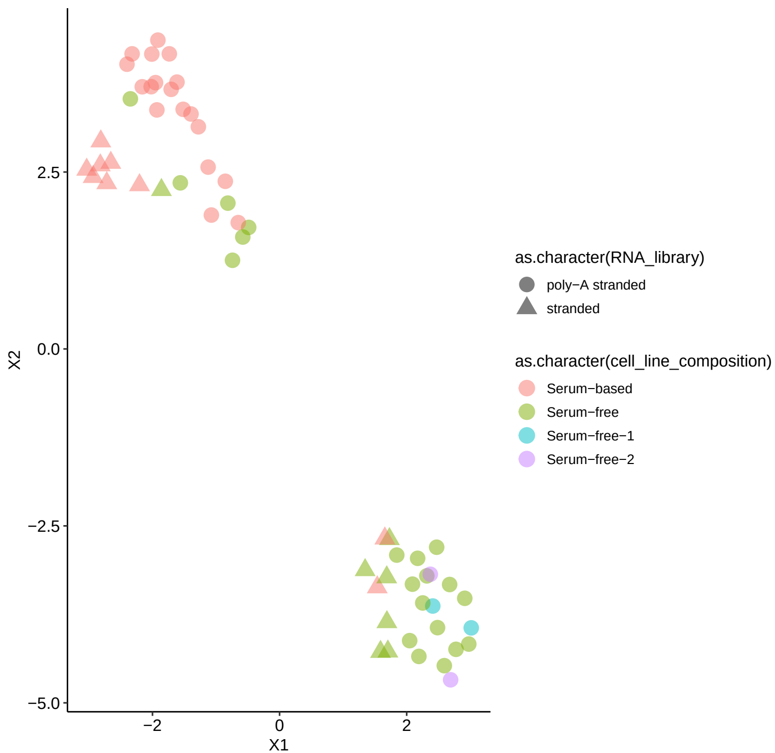
UMAP Clustering
