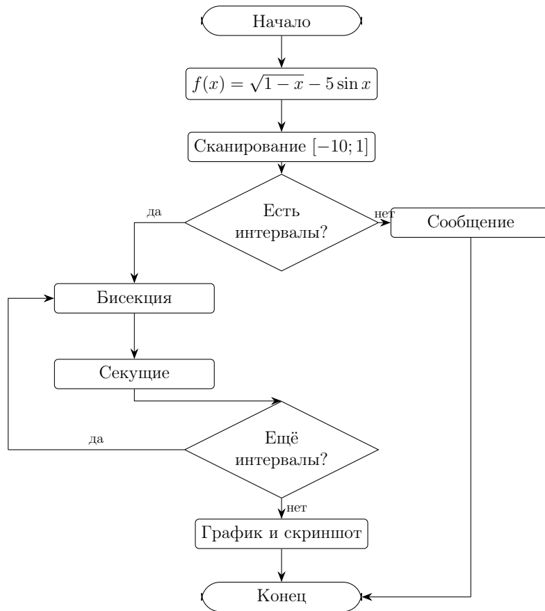
Рис. 2. Блок-схема программы ЛР №1
