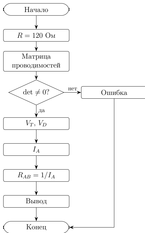
Рис. 8. Блок-схема программы задачи 2.10
