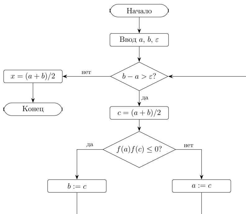
Рис. 1. Блок-схема метода бисекции
