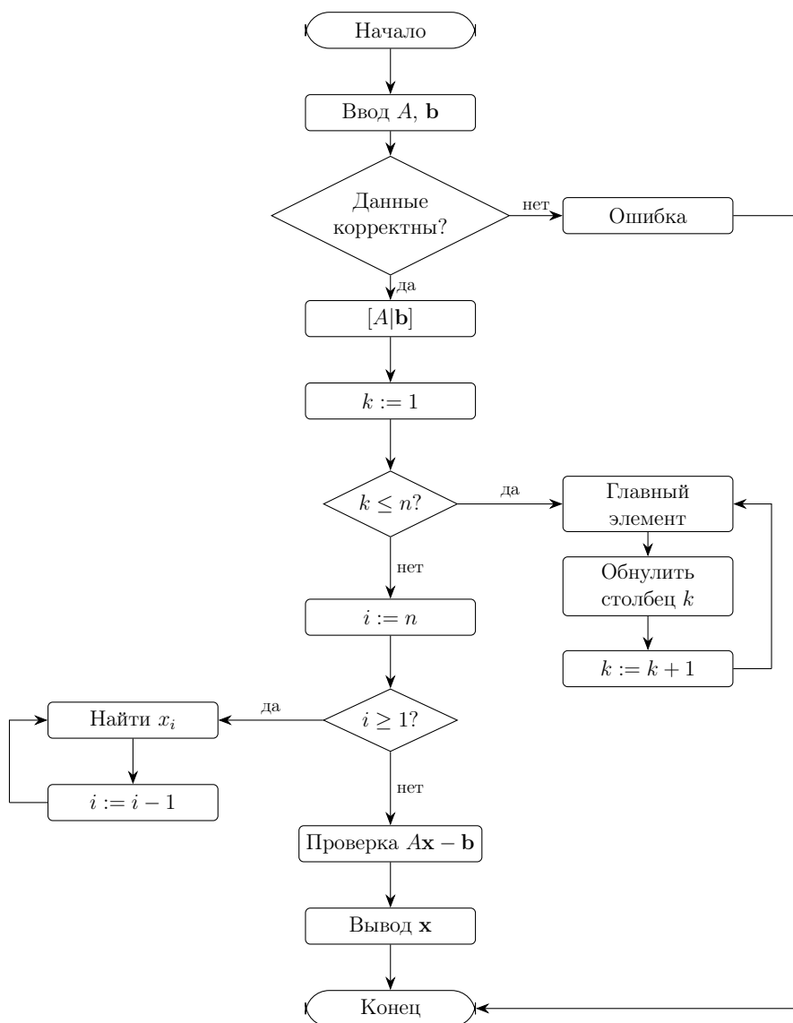
Рис. 5. Блок-схема метода Гаусса
